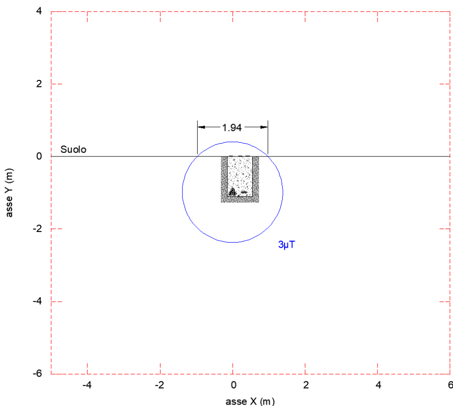
Figura 5.2 - Curva Equilivello 3μT – 1 terna di cavi MT
