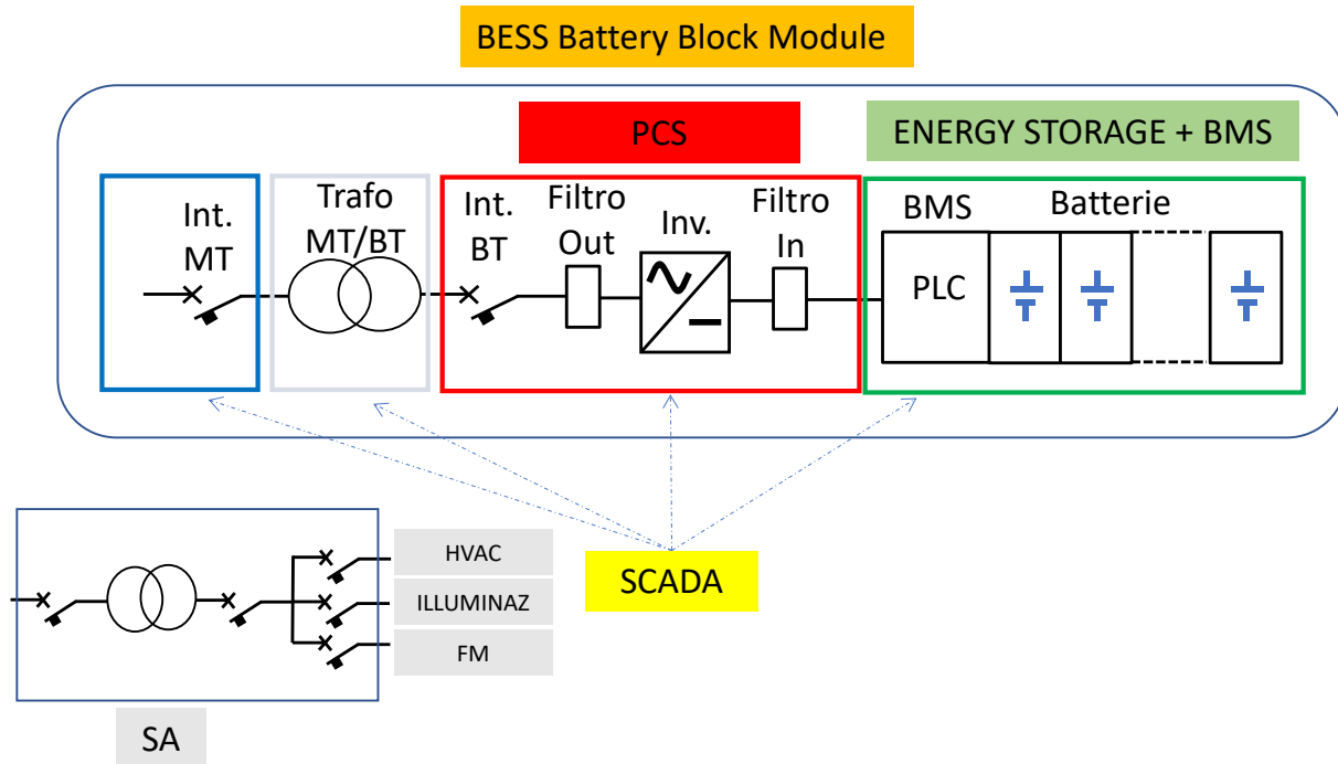
Figura 3.4 – Configurazione di un BESS battery block
