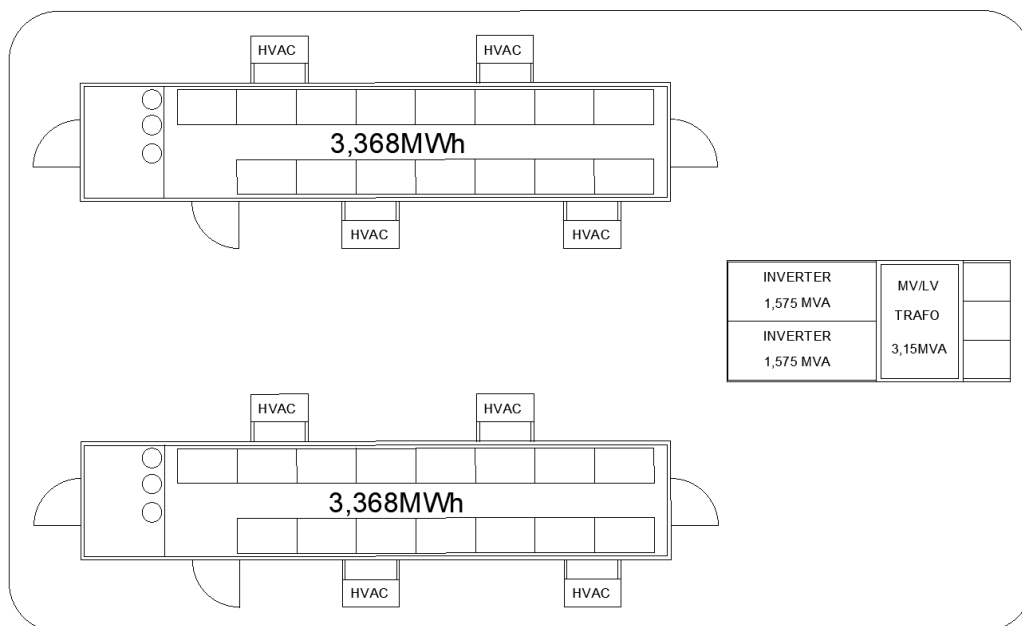
Figura 6.2 - Layout singolo battery block
