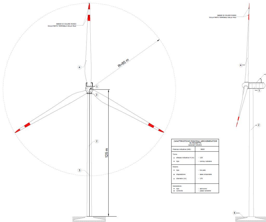
Figura 3.2 – Aerogeneratore tipo SG 6.2-170 altezza al mozzo 125m, e diametro rotore di 170m
