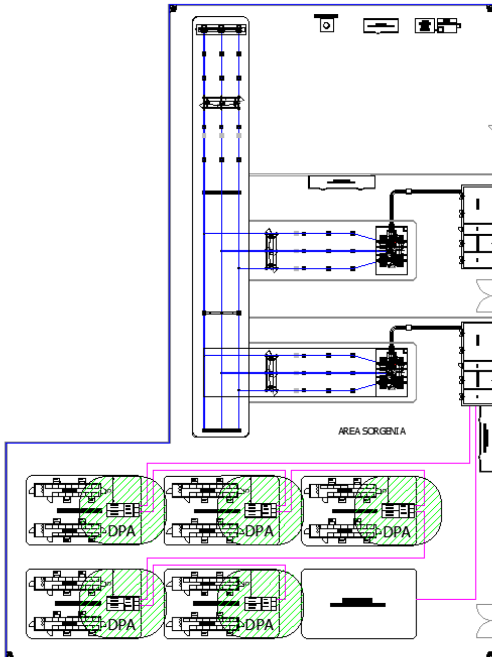
Figura 6.3 - DPA (in m) per le cabine di conversione sistema BESS
