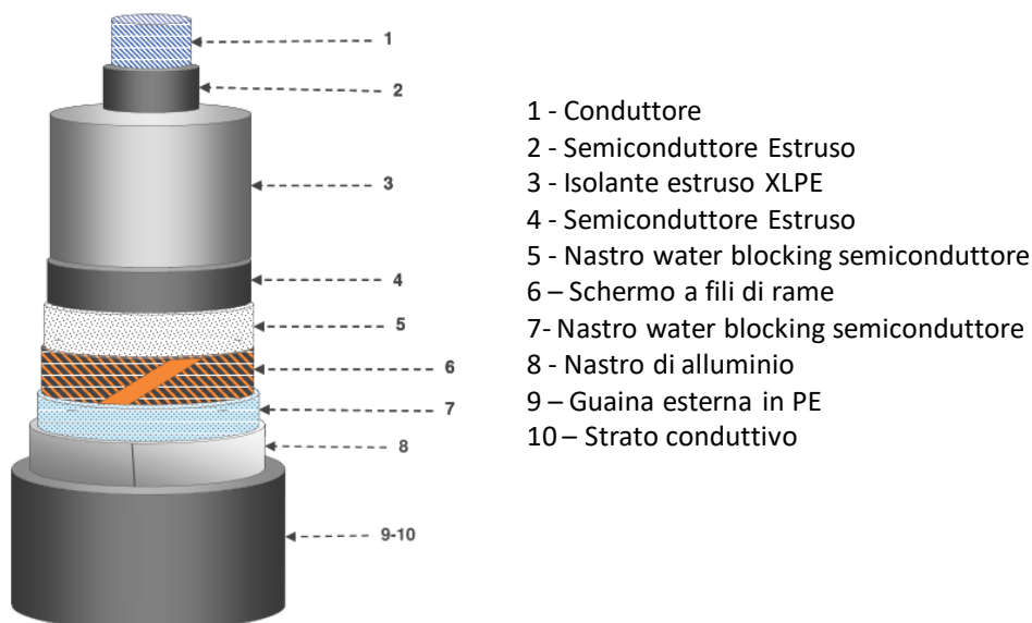
Figura 3.6 – Cavo AT 150 kV tipo ARE4H1H5E 87/150kV
