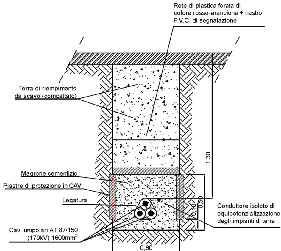
Figura 3.7 – Modalità di posa Cavo AT 150 kV
