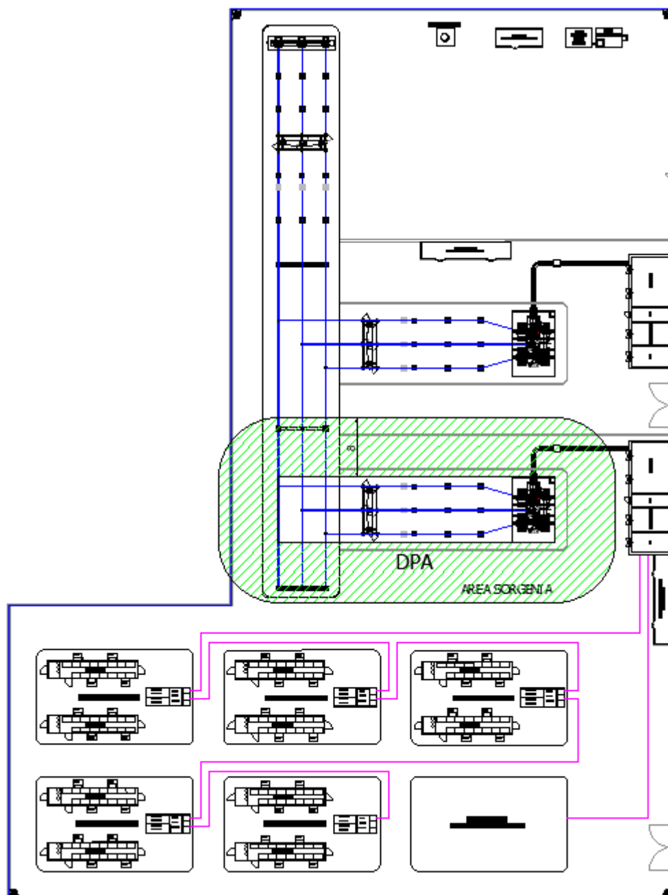
Figura 7.1 - DPA (in m) per lo stallo trasformazione nella SSE Utente 150/30 kV
