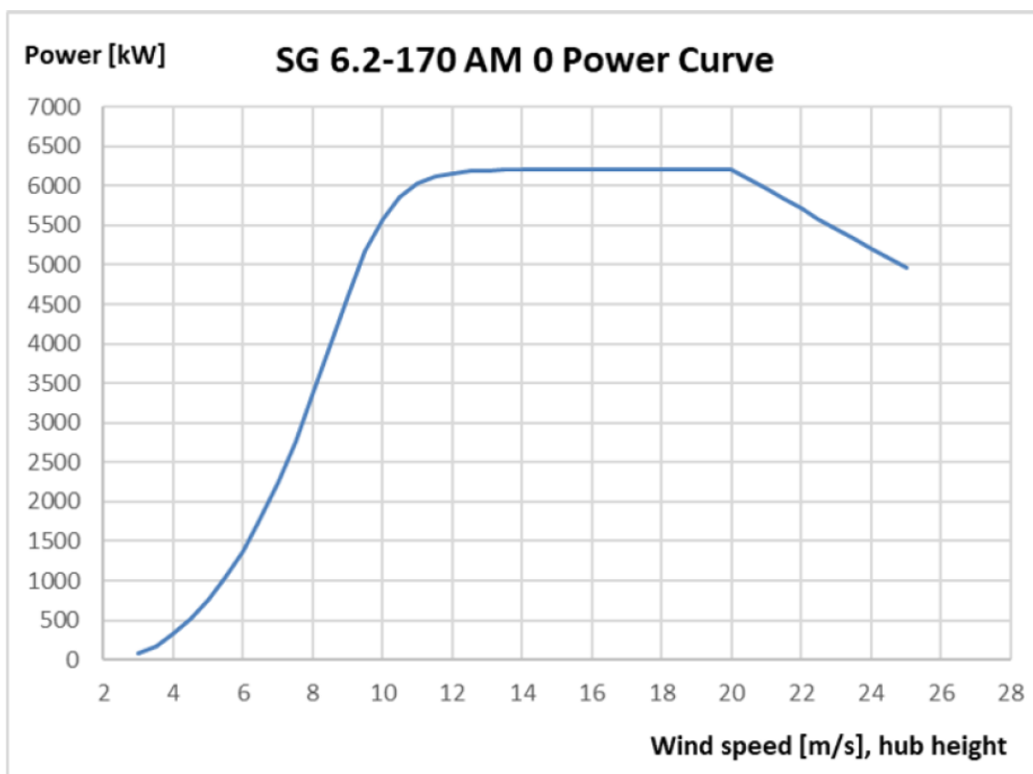
Figura 3.3 – Curva di potenza generatore tipo SG 6.2-170 da 6,2 MW
