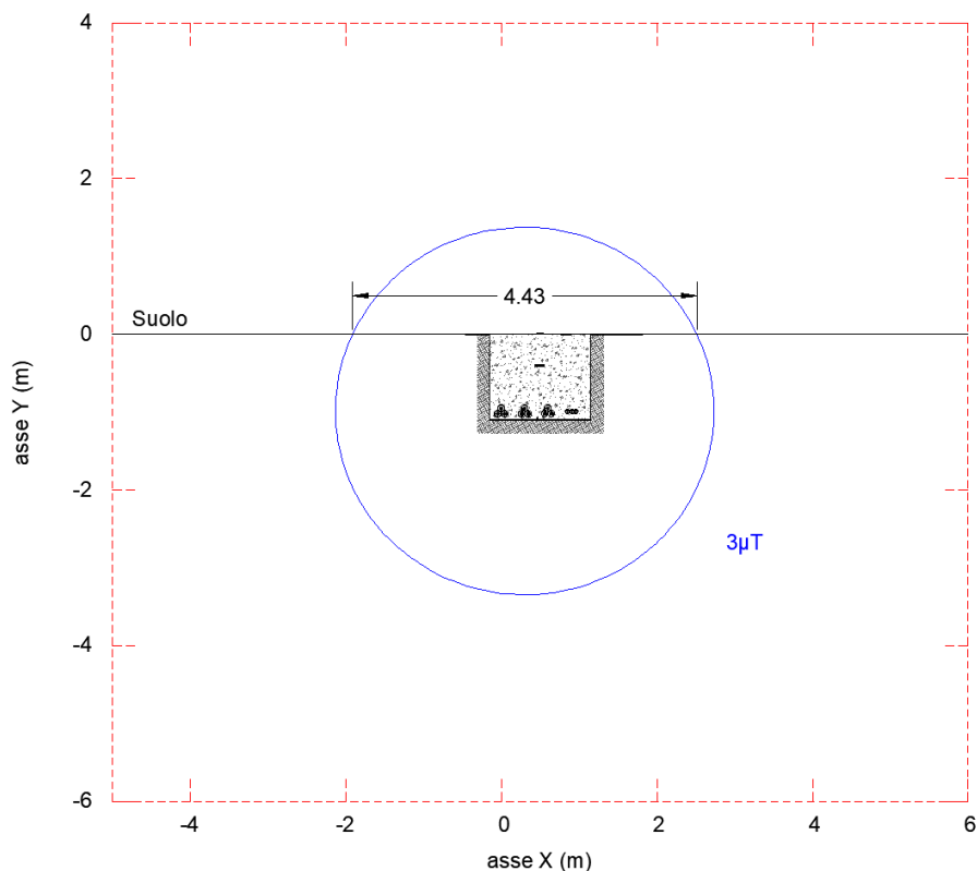
Figura 5.4 - Curva Equilivello 3μT – 3 terne di cavi MT
