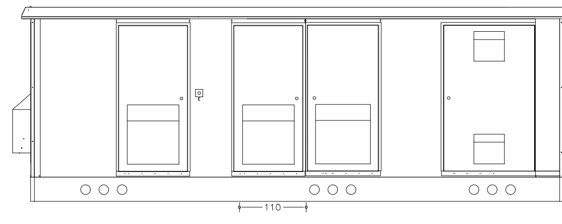
PROSPETTO FRONTALE / FRONT VIEW
