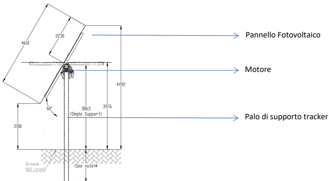
Figura 22- Esempio tracker
