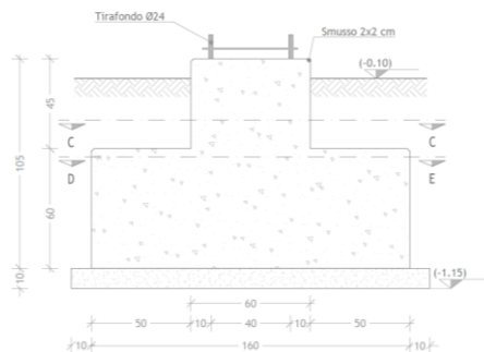
Fig. Pianta e sezione fondazione per sostegno tripolare
