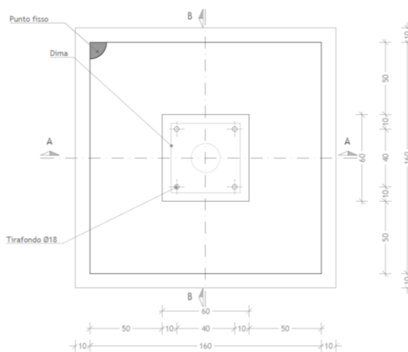
SEZIONE A-A/B-B Scala 1:20
