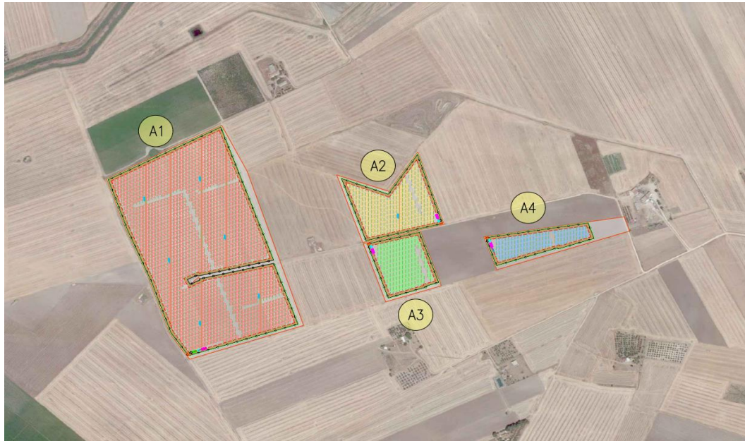
Tav. n. 2 - Schema irriguo Oliveto
