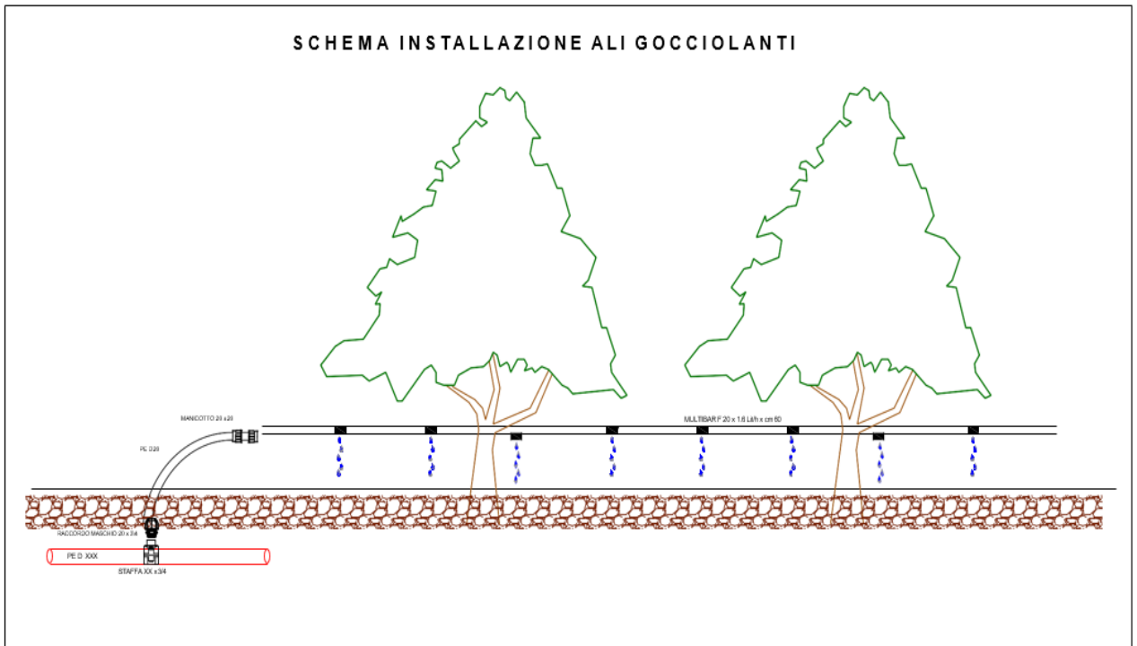
Tav. n. 5 - Installazione valvola di scarico su terminale delle testate
