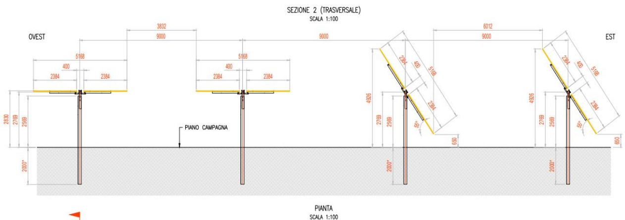
Particolare strutture sostegno moduli pannelli e distanze di campo (interfila m 9)
