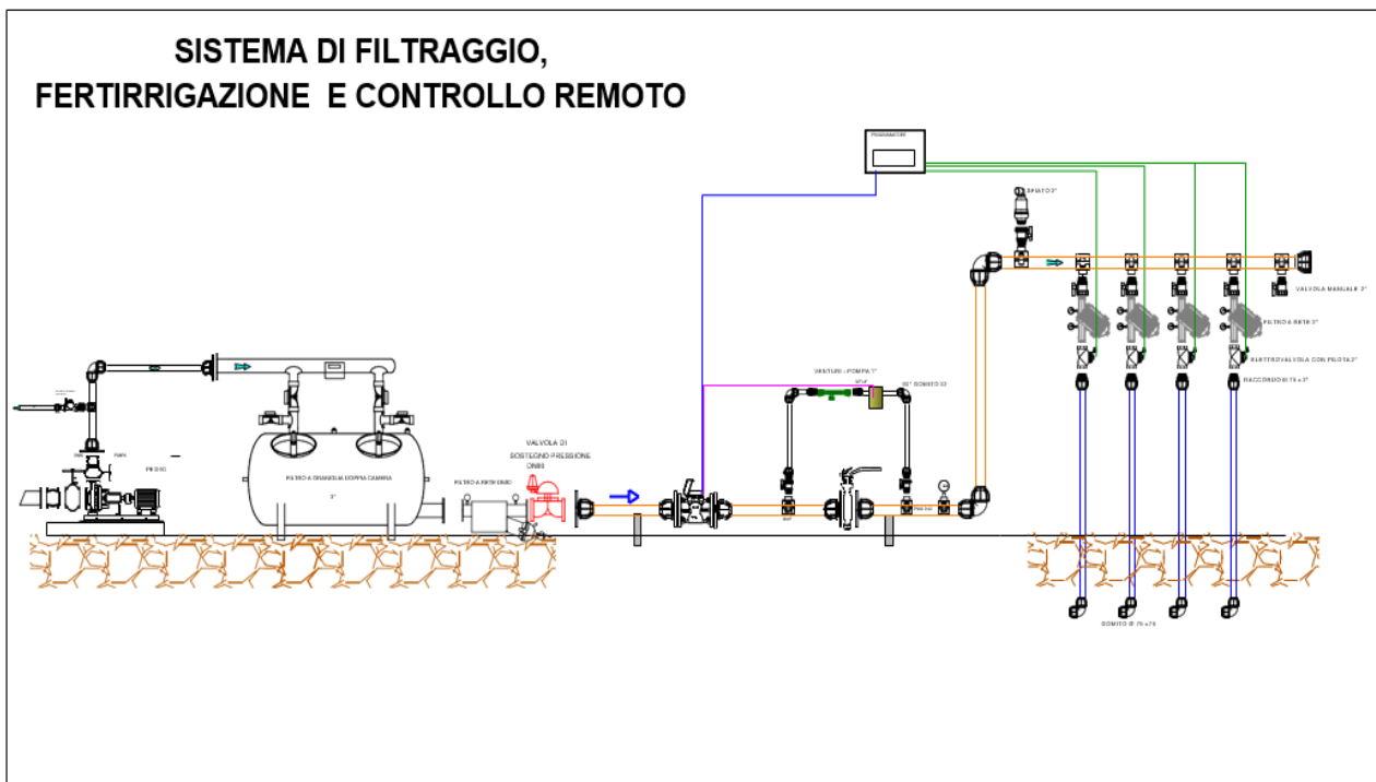
Tav. n. 3 - Sistema di filtraggio, fertirrigazione e controllo remote
