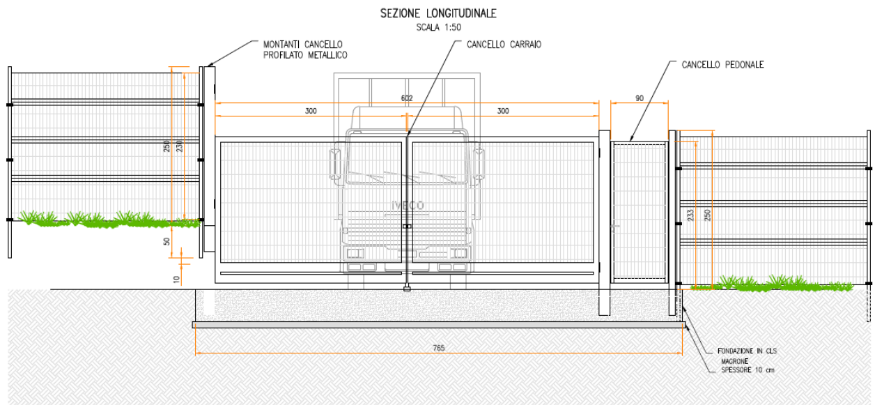
Figura 4.6: Particolare accesso
