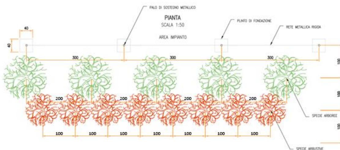
Figura 5.2 - Tipologico del filare di mitigazione
