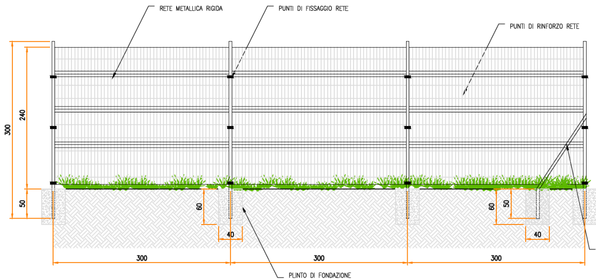
Figura 4.5: Particolare recinzione
