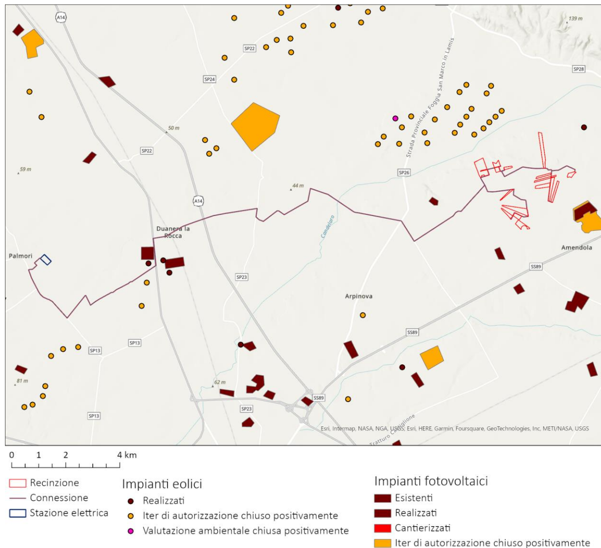
Figura 10.1: Impianto in progetto (in blu) e impianti fotovoltaici/eolici presenti nell'area oggetto di studio – Elaborazione Montana S.p.A.
