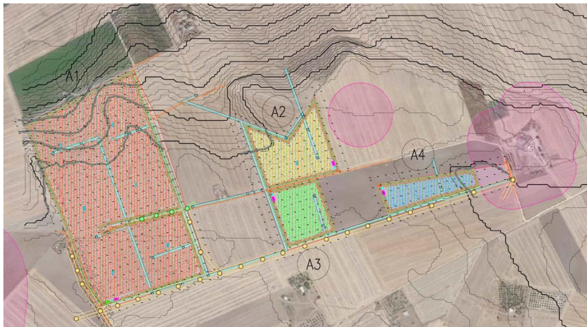
Figura 4.1 - Layout di progetto – Sezione A
