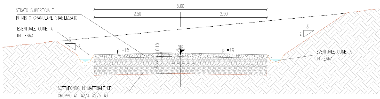
Figura 4 A_16_d_1 Sezioni tipo – Strade di nuova realizzazione
