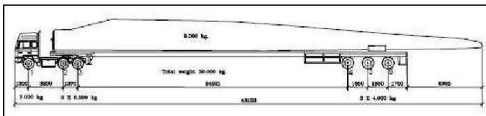
Figura 11 - Dimensioni autoarticolato
