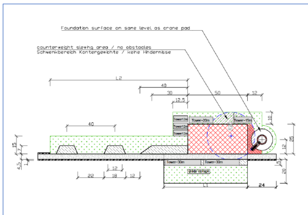
Figura 14 – tipologico della piazzola di montaggio
