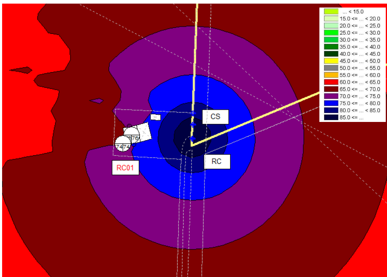
Figura 8 – Stralcio planimetrico della mappa acustica calcolata in corrispondenza del recettore residenziale RC01 nelle fasi di cantiere maggiormente critiche (Fase 19).
