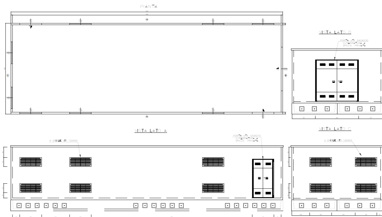
Pianta e Prospetti – Tipologico (15x5m)
