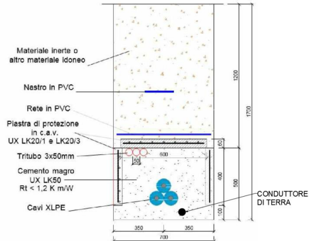
ESEMPIO DI POSA A TRIFOGLIO IN TERRENO AGRICOLO
