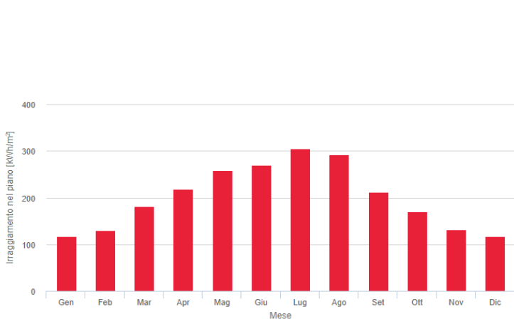
Figura12 - Irraggiamento mensile nel piano di inseguimento
