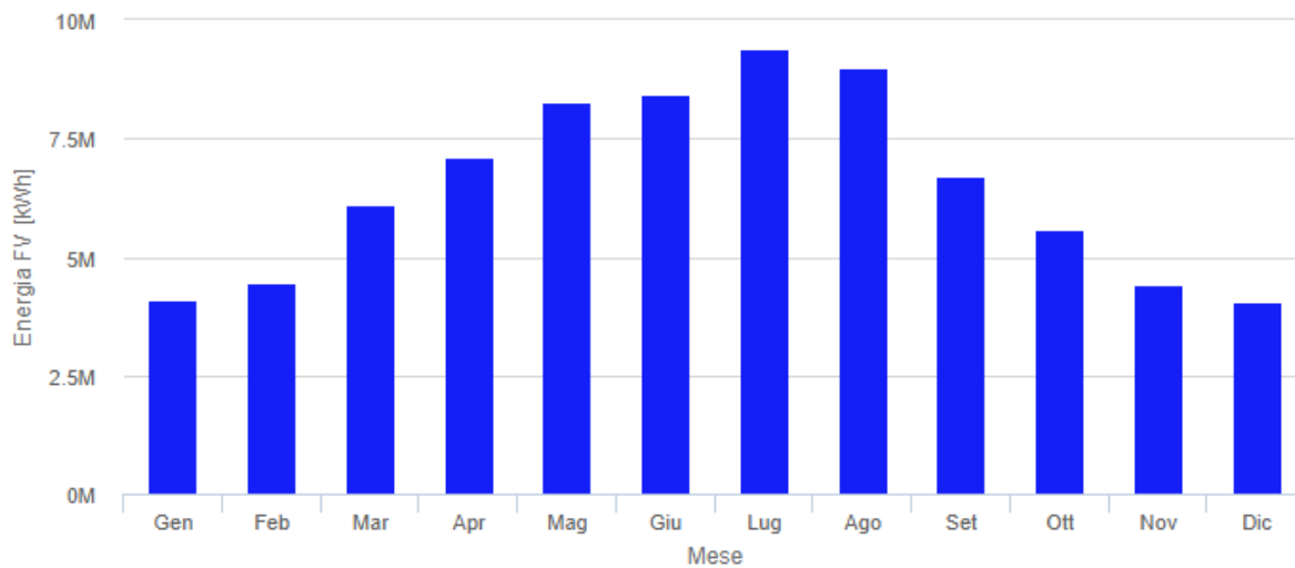
Figura 11- Energia mensile da sistema FV ad inseguimento
