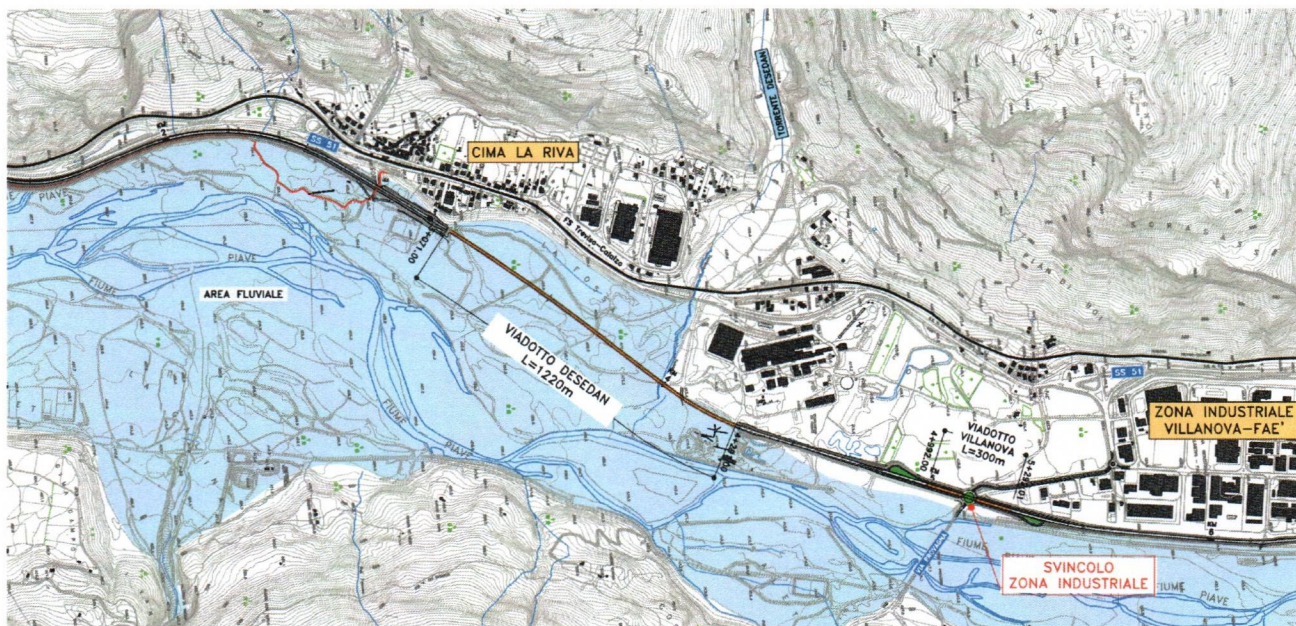
Fig. 2 Planimetria Alternativa 1 (selezionata), stralcio elaborato VA407-T00EG01GENPF01-A-signed
