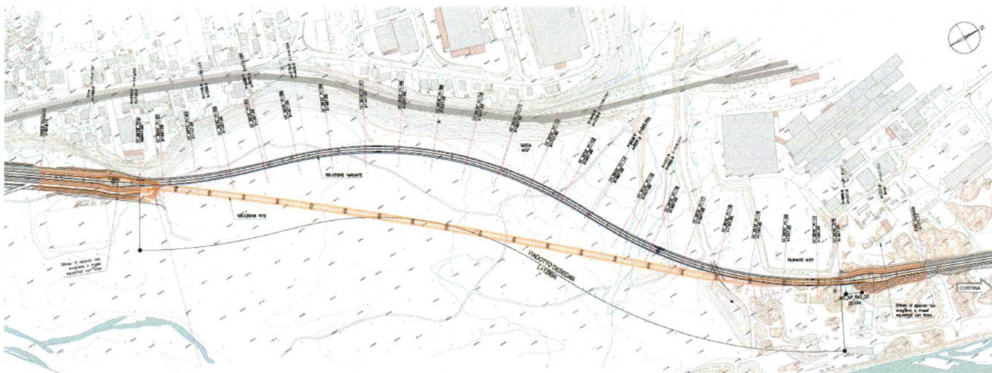
Fig. 1 Planimetria di progetto con indicazione Variante Desedan.
