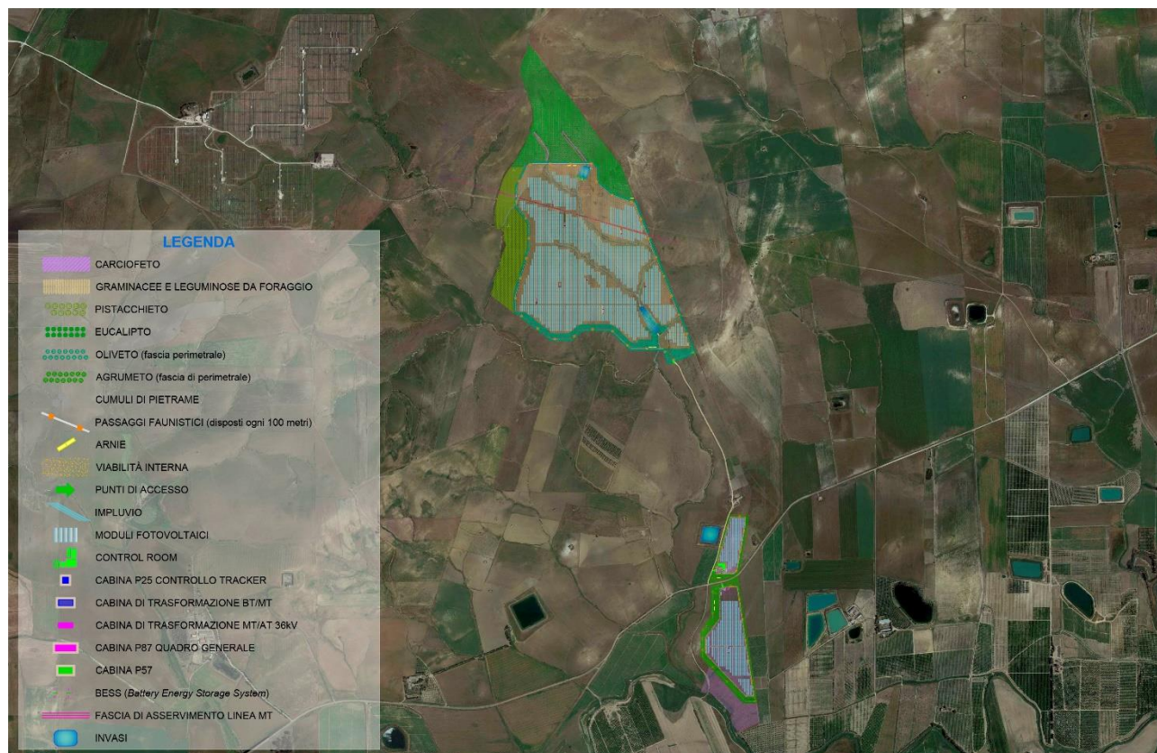
Figura 5 – Layout impianto agrivoltaico
