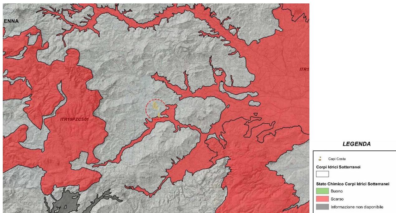
Figura 8 – Stralcio Tav. B4 – Carta dello stato chimico dei corpi idrici sotterranei
