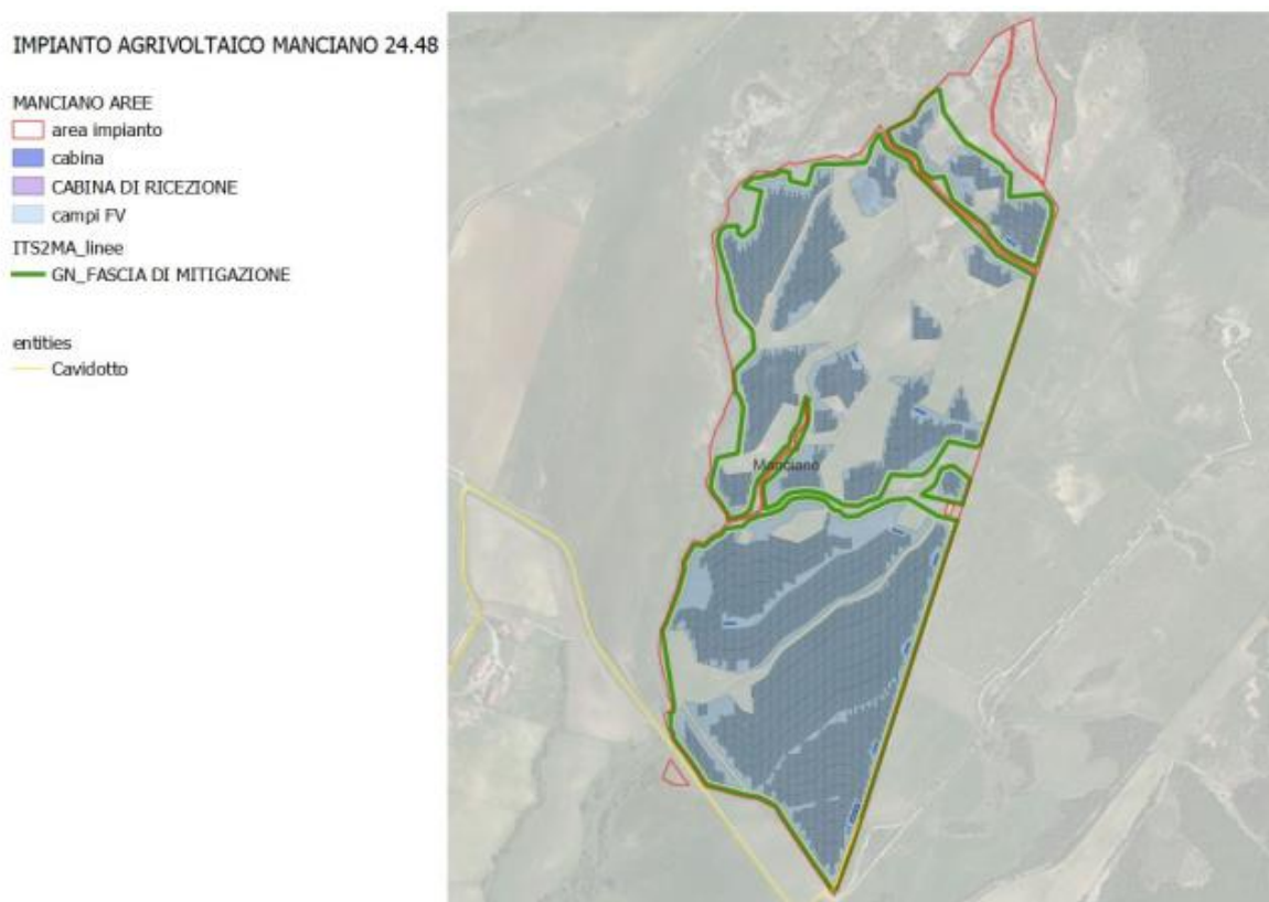
Fig. 25 – Fascia perimetrale produttiva di mitigazione
