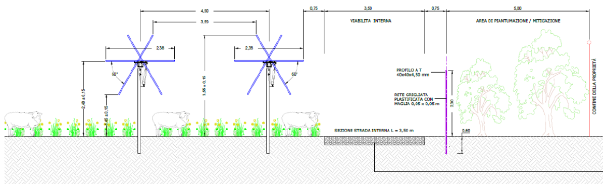
Fig. 32 - Distanze caratteristiche struttura coltivazione
