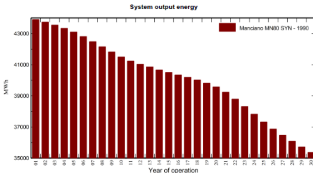
Fig. 37 – Producibilità dell’impianto con degrado moduli (30 anni)
