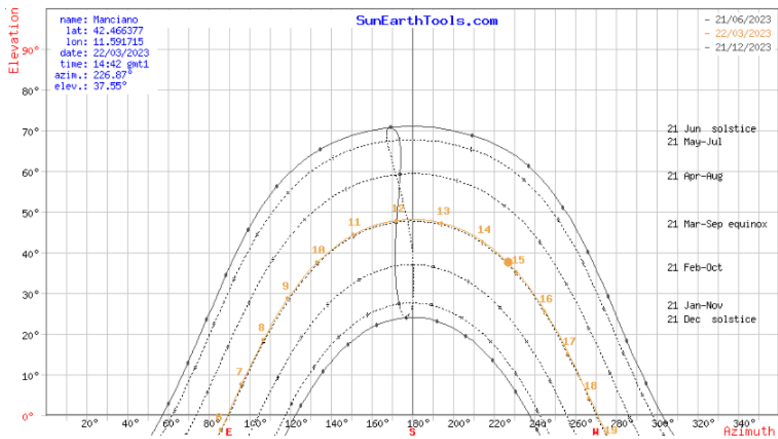
Fig. 35 - Diagramma Solare Polare (Manciano)
