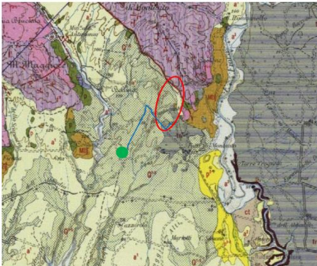
Fig. 8- Carta geologica
