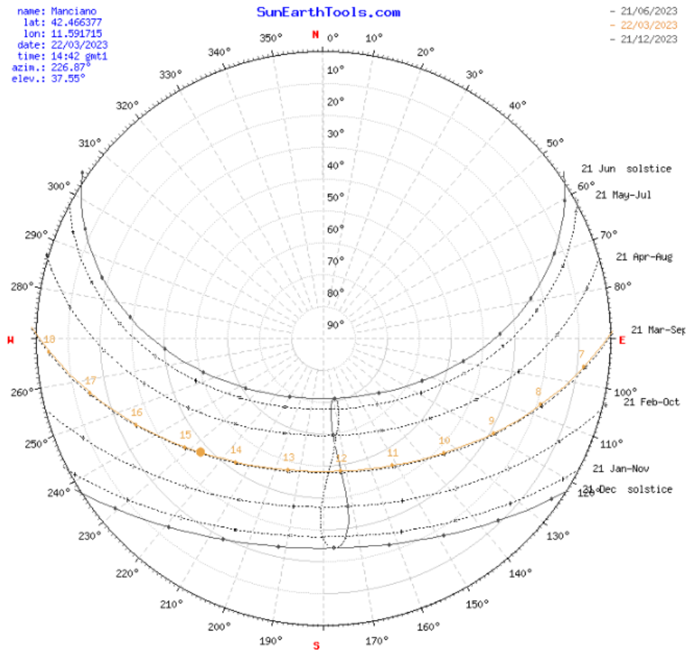
Fig. 34 - Diagramma Solare Polare (Manciano)
