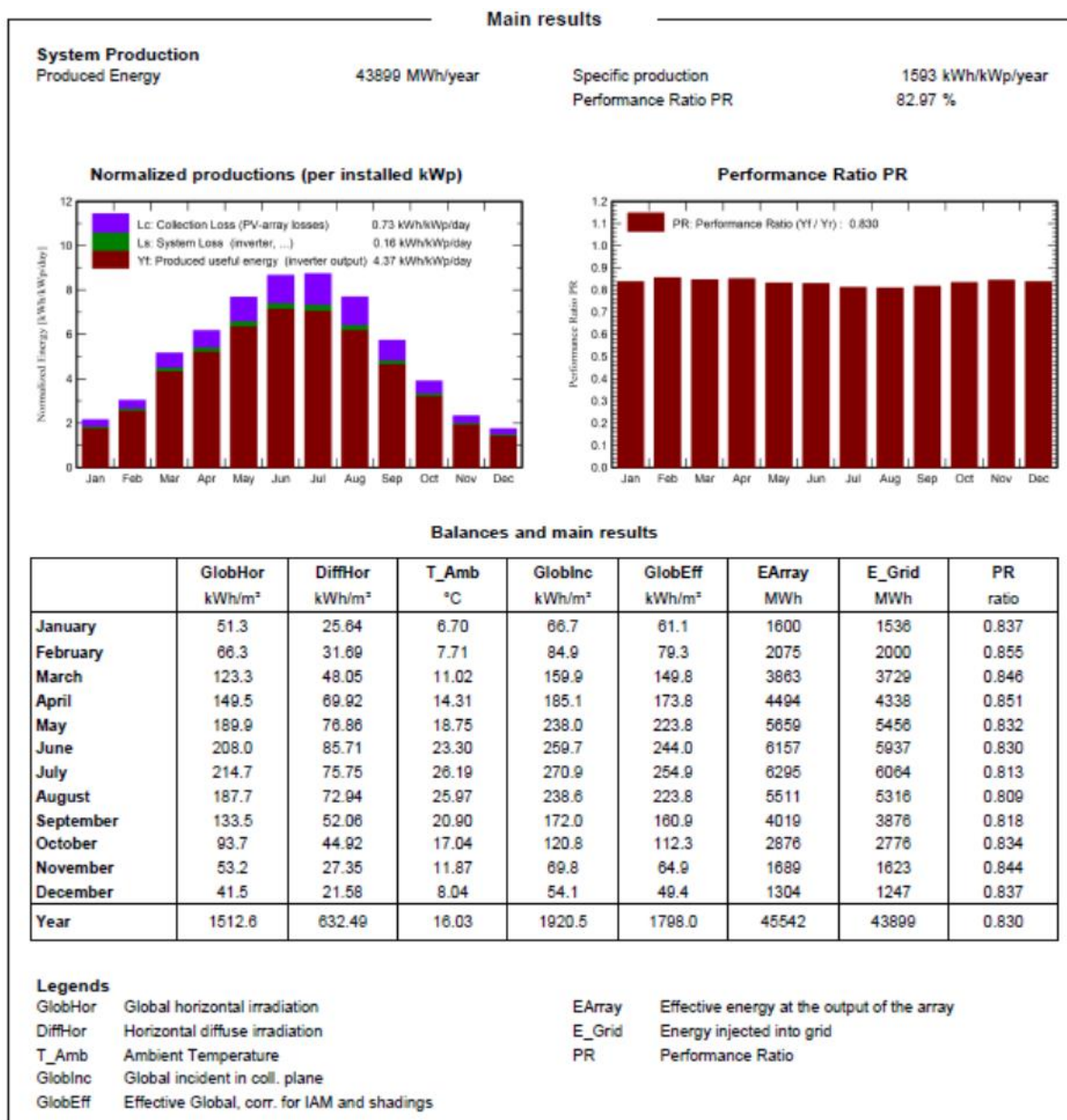
Fig. 36 - Risultati di calcolo (Fonte: PVsyst - Meteonorm)
