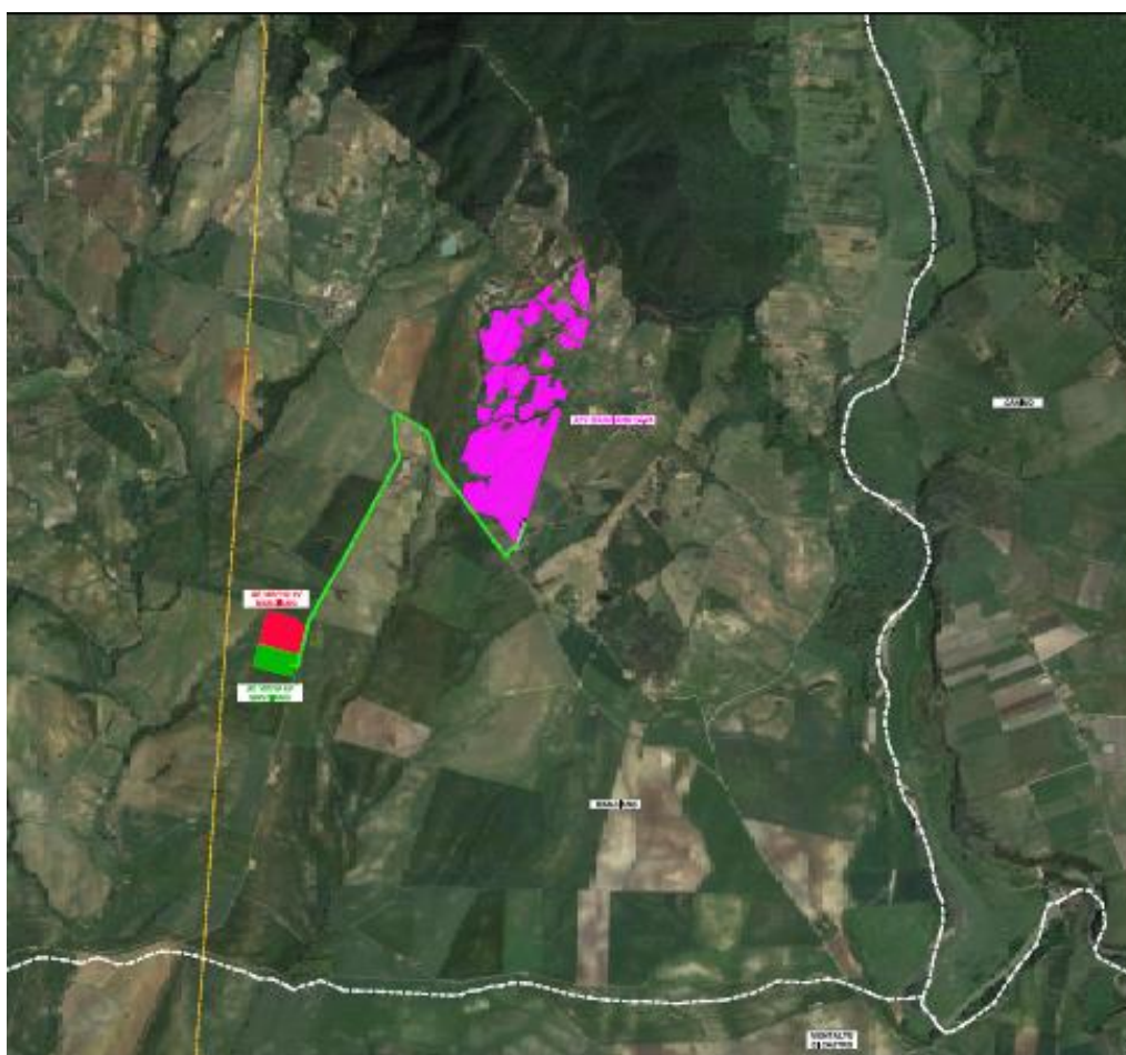
Fig. 45 – Ortofoto con indicazione del percorso del cavidotto
