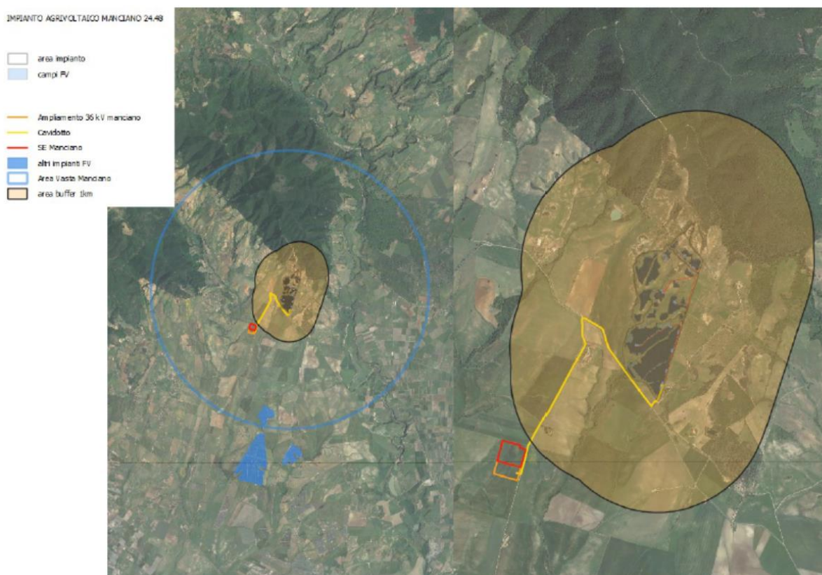
Fig. 10 – Impianti fotovoltaici esistenti in area buffer 1km e area vasta 5 km.
