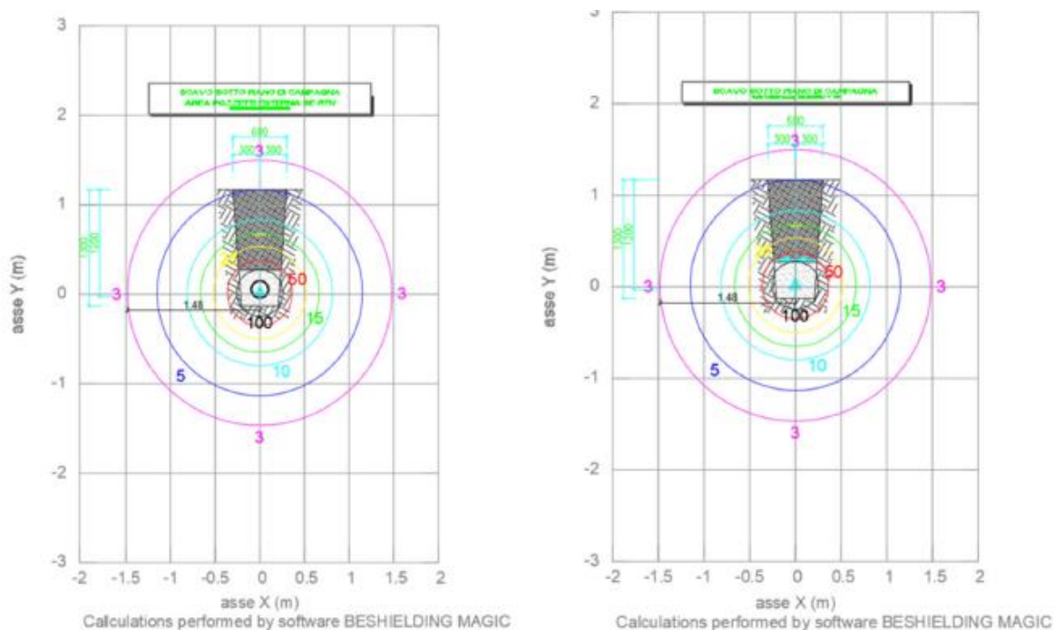
Fig. 46 – Livelli di campo magnetico generati dal cavidotto
