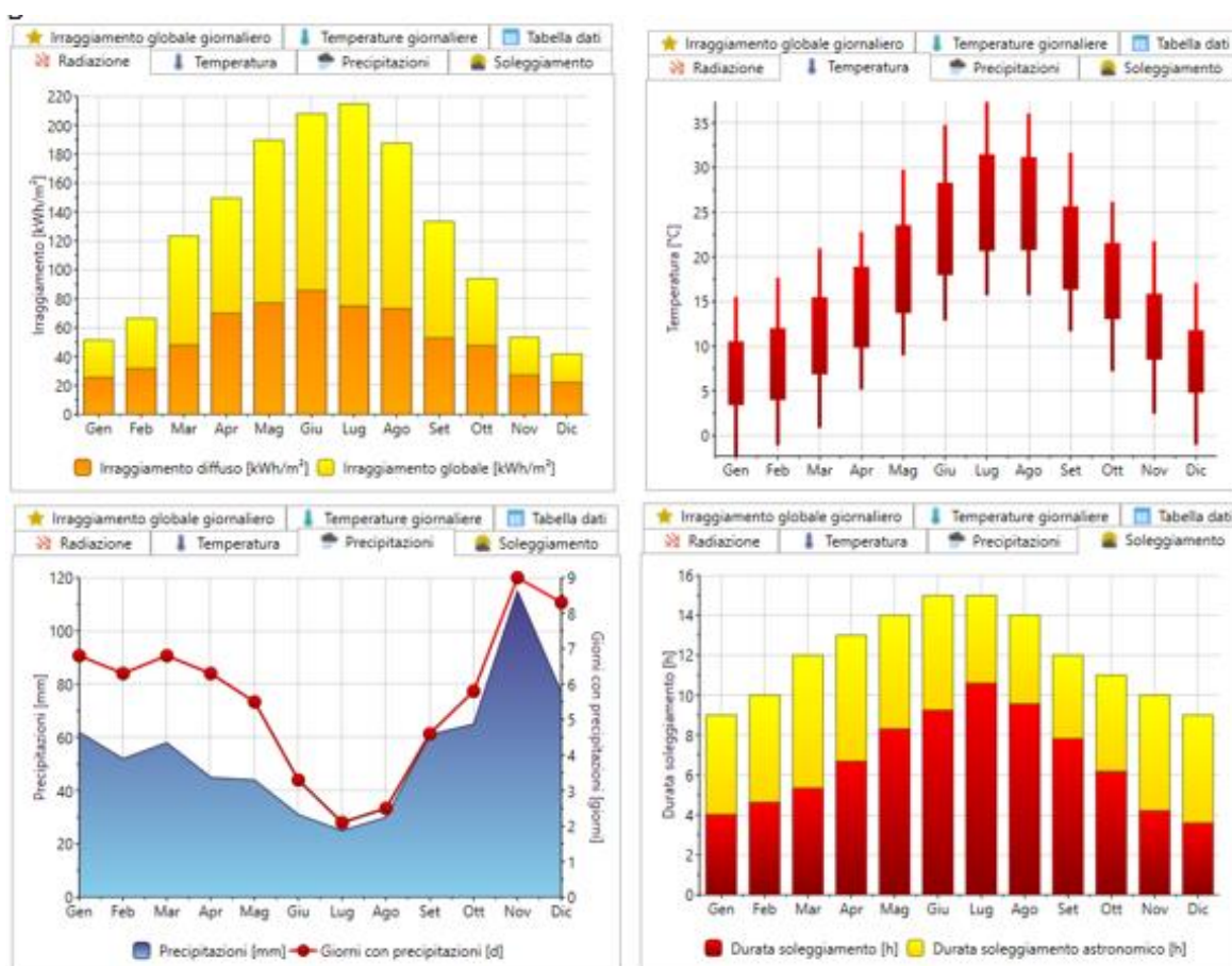
Fig. 33 – Dati di radiazione, temperatura, precipitazioni e soleggiamento (Riferiti al sito di Manciano)
