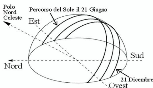
Fig. 39 - Movimento apparente del disco solare per un osservatore situato ad una latitudine nord attorno ai 45°. Per tutte le località situate tra il Tropico del Cancro e il Polo Nord Geografico il disco solare non raggiunge mai lo zenit.
