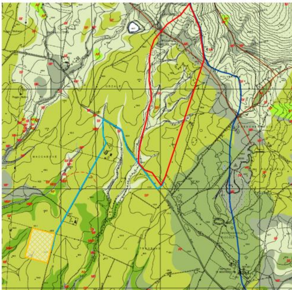
Fig. 9 – Stralcio della carta idrogeologica e delle aree con problematiche idrogeologiche- TAV.6.e.7. (Ai sensi del DPGRT 26/R/07)
