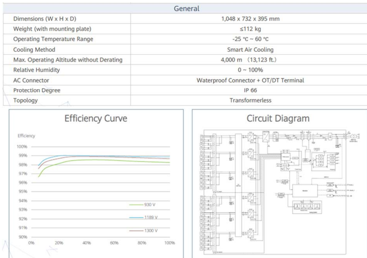
Fig. 13 - Dimensioni, specifiche tecniche e prestazionali dell'inverter
