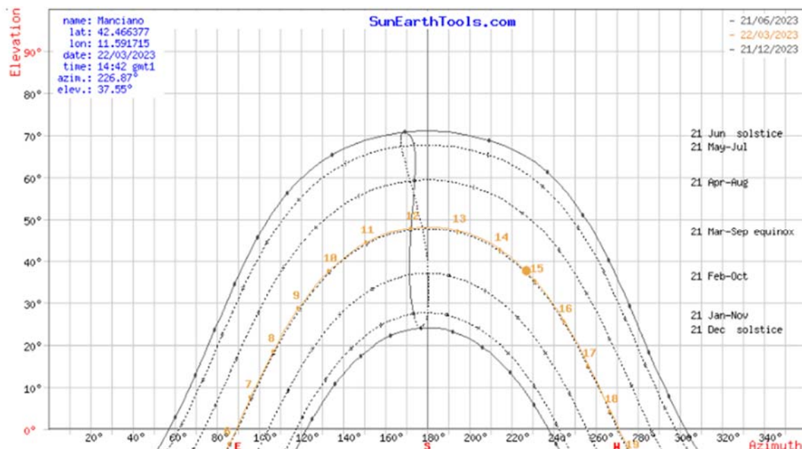
Fig. 26 - Diagramma Solare Polare (Manciano)
