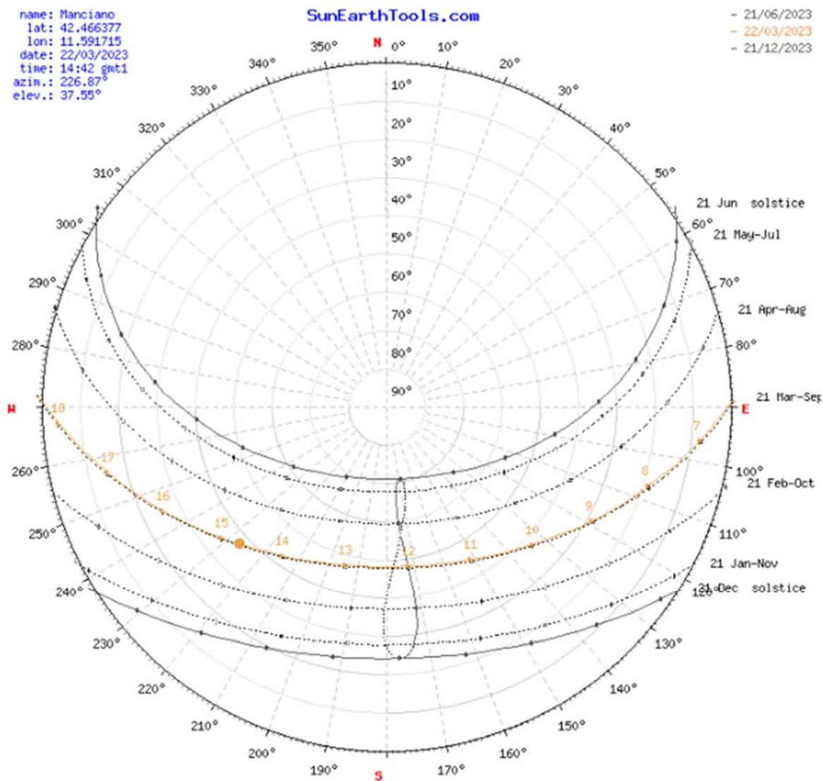
Fig. 25 - Diagramma Solare Polare (Manciano)
