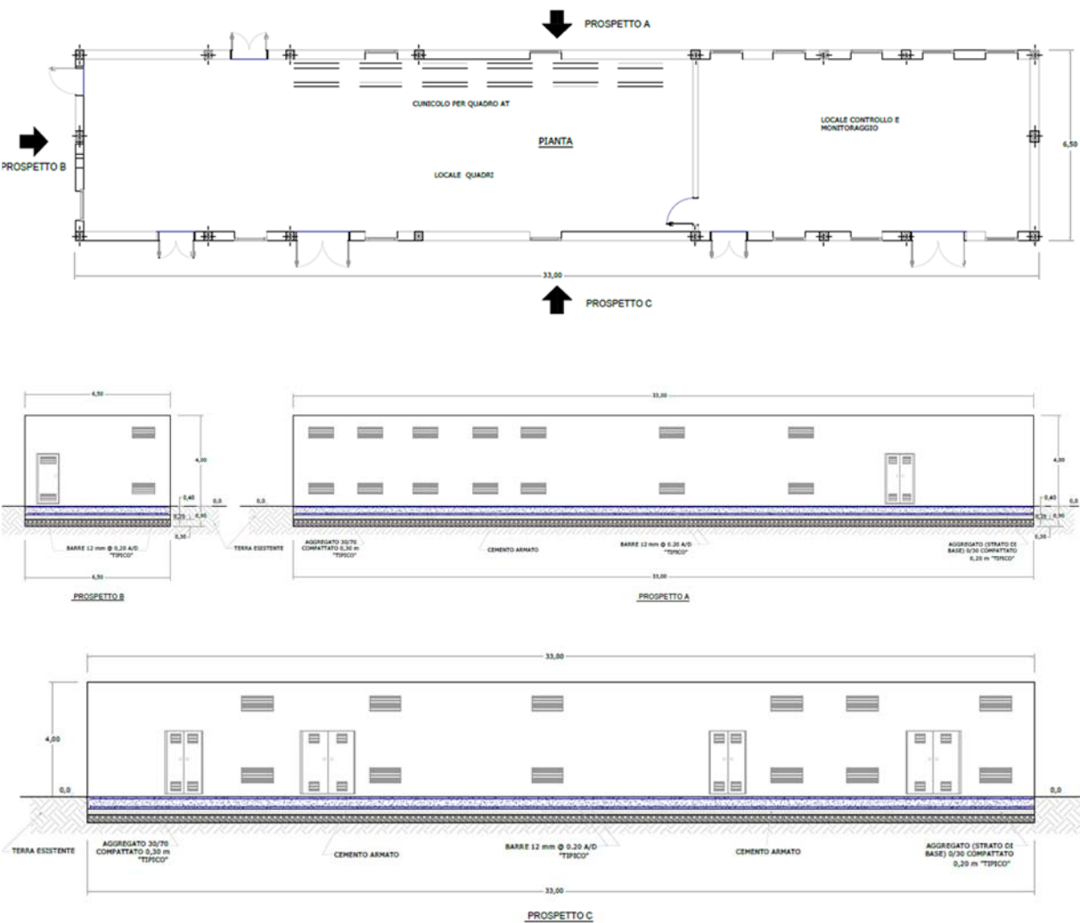
Fig. 20 - Cabina di ricezione
