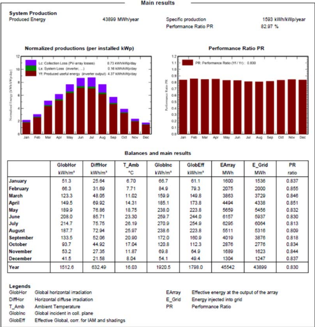
Fig. 27 - Risultati di calcolo (Fonte: PVsyst - Meteonorm)
