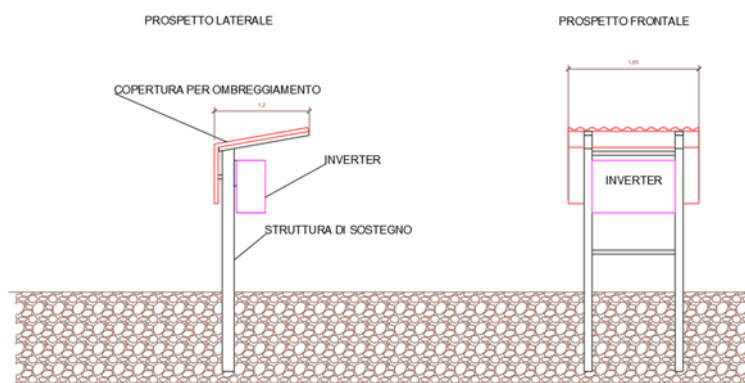
Fig. 10 - Tipico struttura supporto inverter
