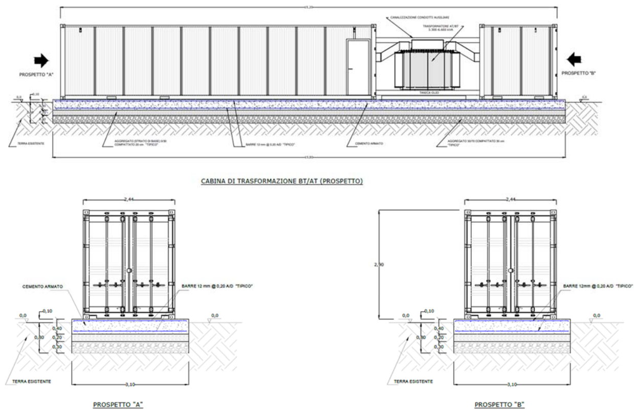
Fig. 19 - Cabina di trasformazione BT / AT
