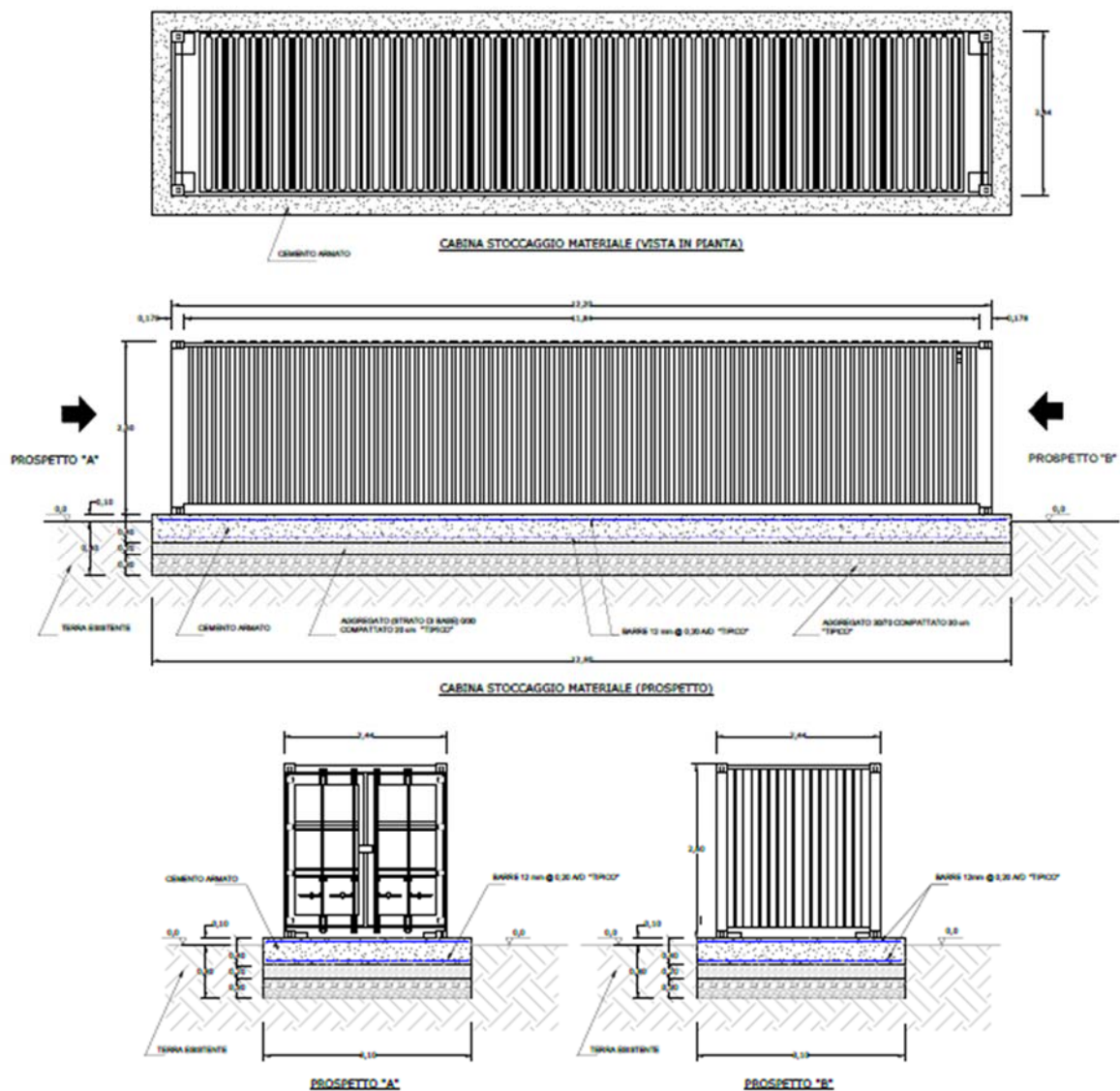
Fig. 21 - Cabina stoccaggio materiale
