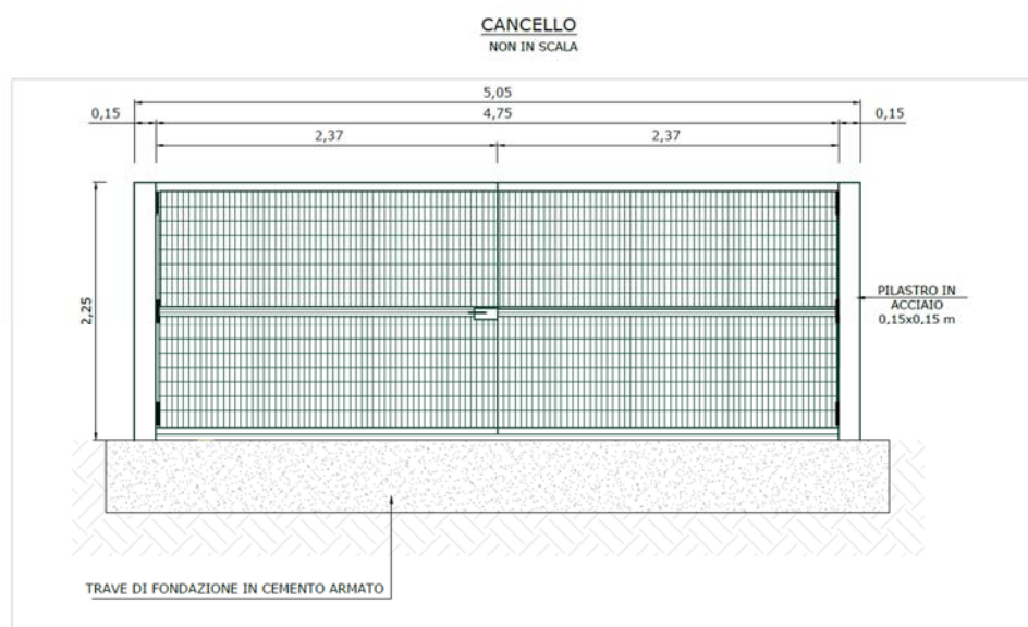
Fig. 16 – Cannello a doppia anta
