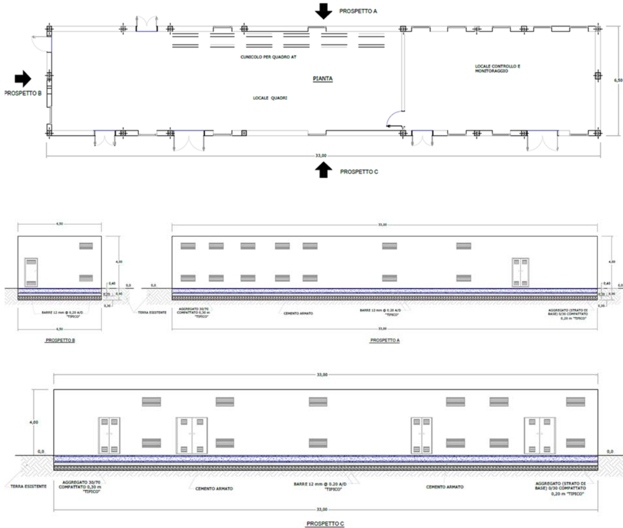
Fig. 13 - Cabina di ricezione
