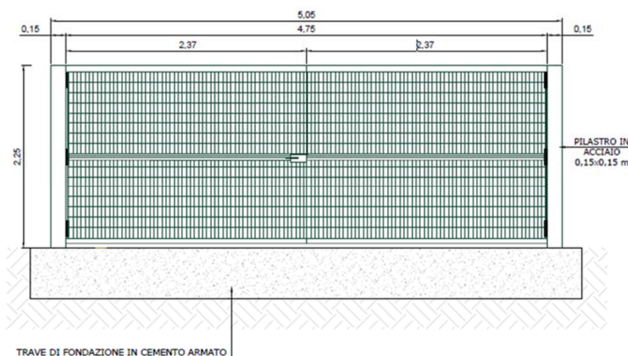
Fig. 17 – Cancelli carrabile
