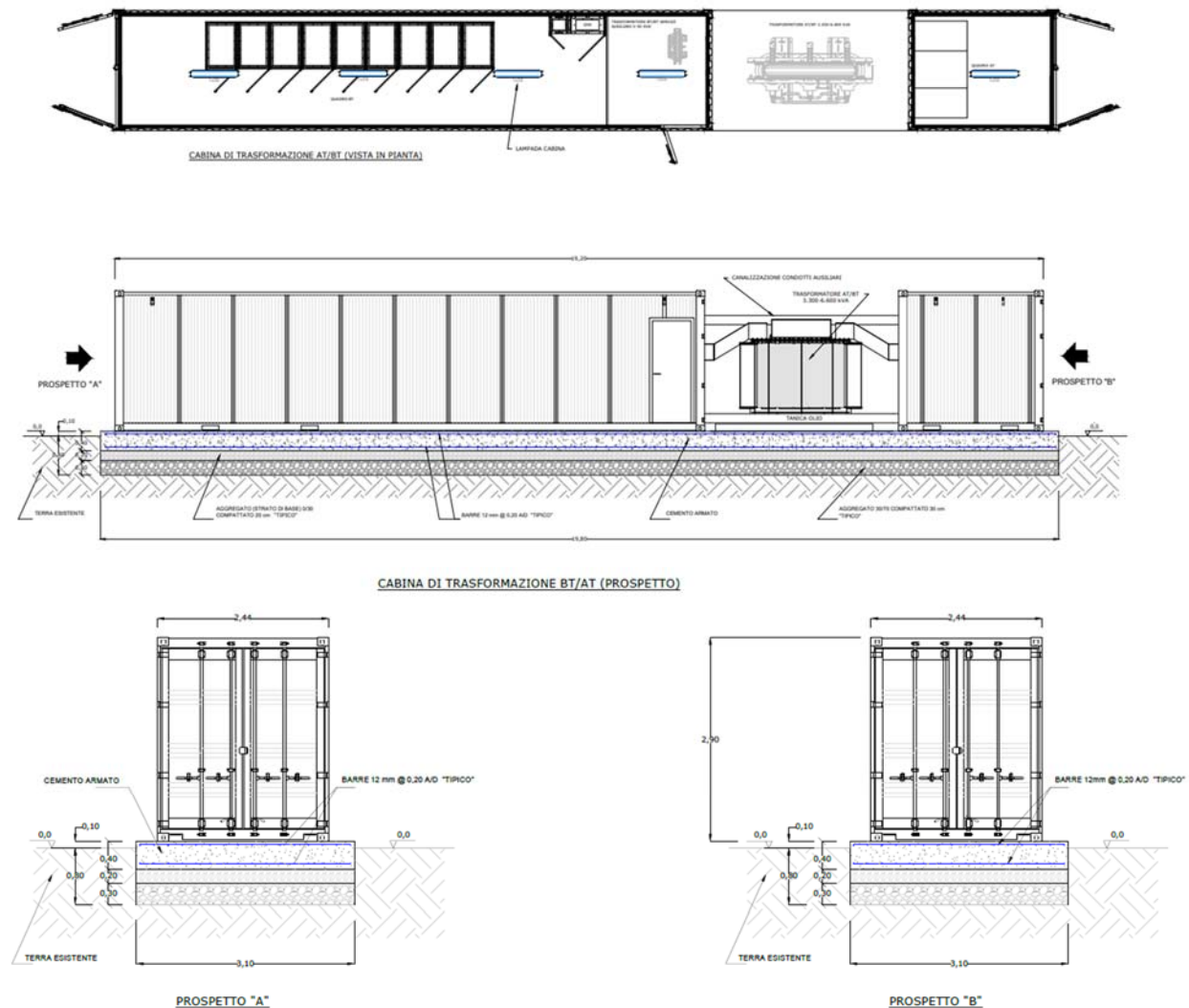
Fig. 12 - Cabina di trasformazione BT/AT
