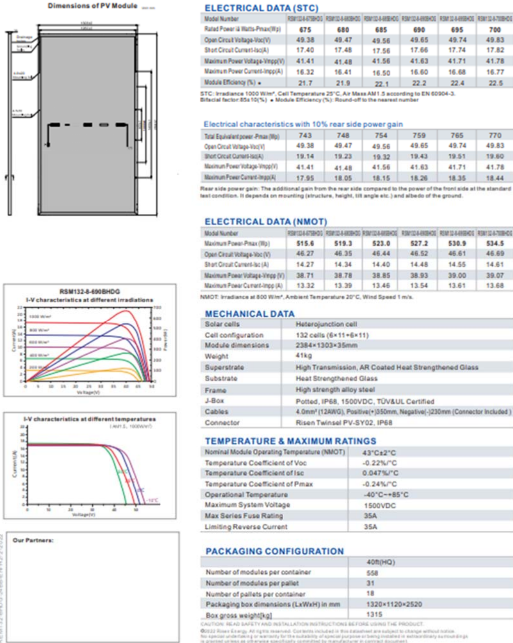
Fig. 1 - Dimensioni, specifiche tecniche e prestazionali pannelli fotovoltaici Risen
