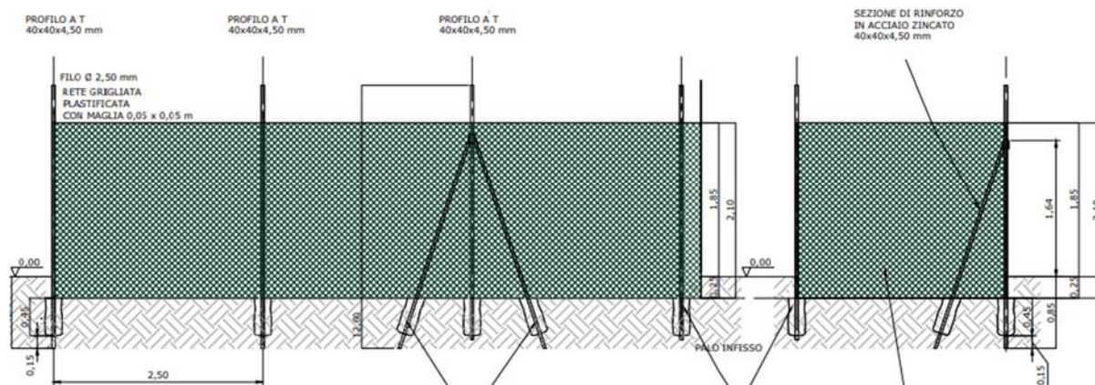
Fig. 16 – Particolare della recinzione
