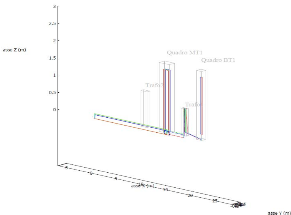
Fig.7 - Modello spaziale cablaggi nelle cabine di ricezione
