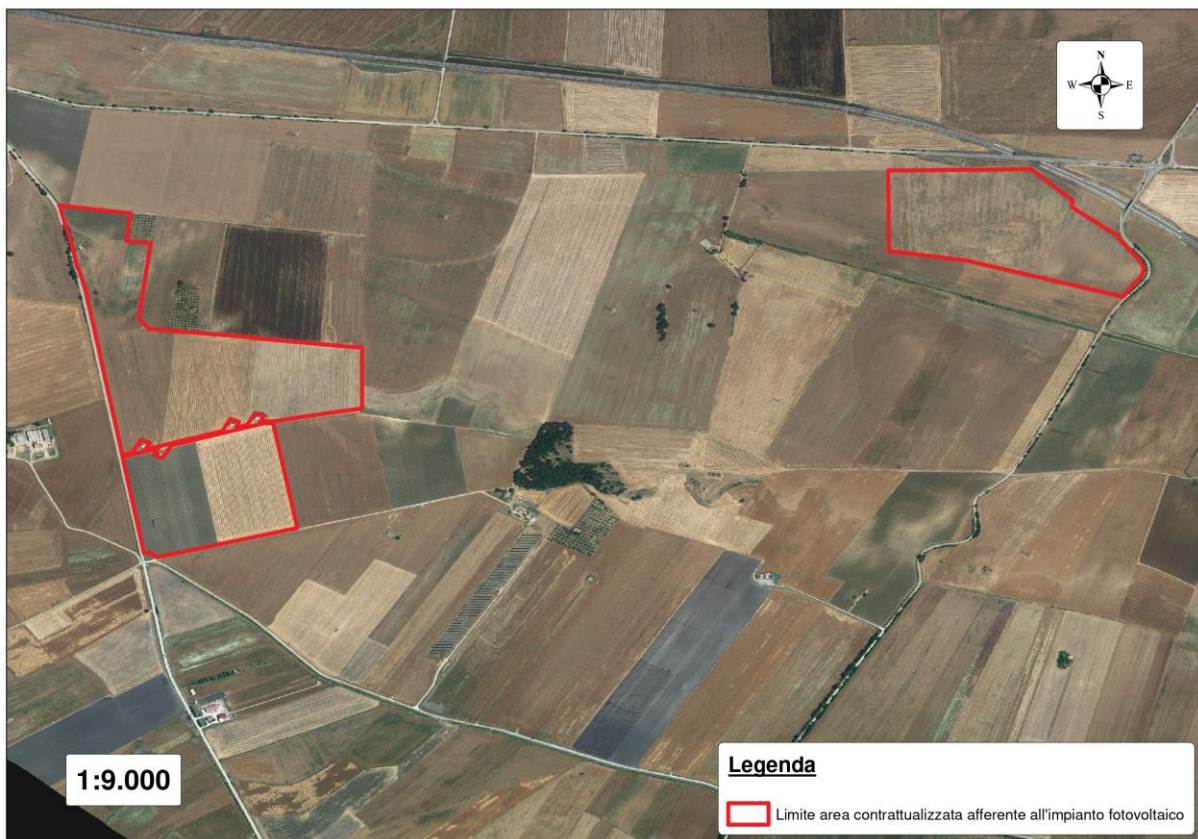
Figura 1 – Area di progetto dell'impianto agrivoltaico su ortofoto.
