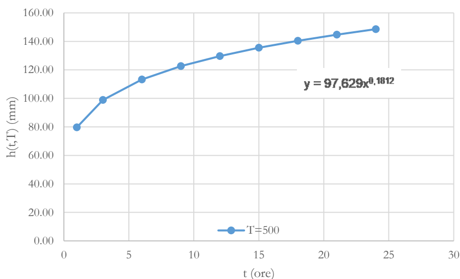
Figura 3 Curva di Possibilità Pluviometrica per T = 500 anni.
