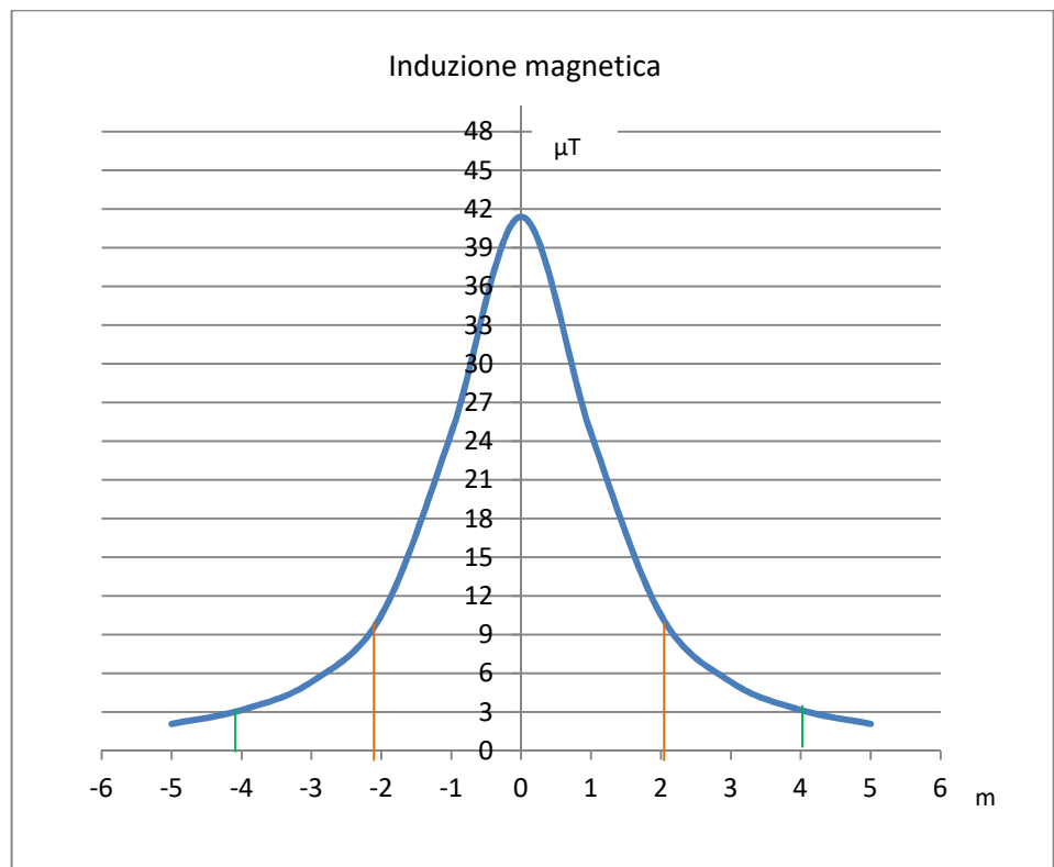
Figura 1 | Rappresentazione grafica del campo elettromagnetico generato dal cavidotto MVC_06 – SE RTN
