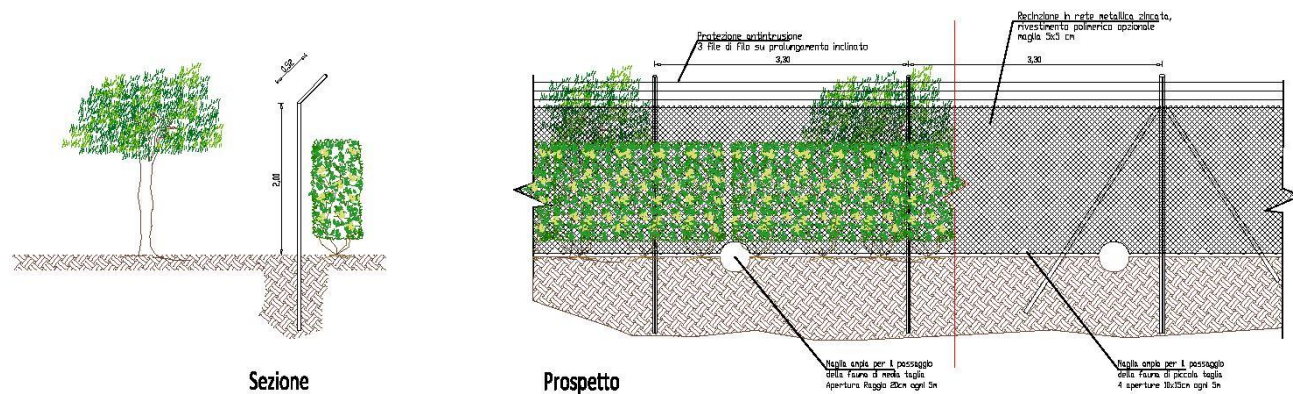
Figura 2 Particolare recinzione impianto agrivoltaico
