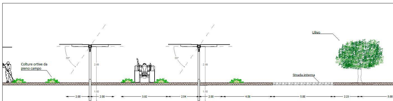
Figura 3 sezione tipo impianto agrivoltaico
