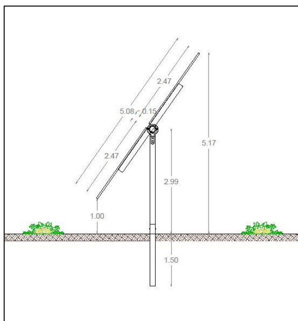
Figura 4 sezione tipo con inclinazione massima del tracker monoassiale pari a 55°
