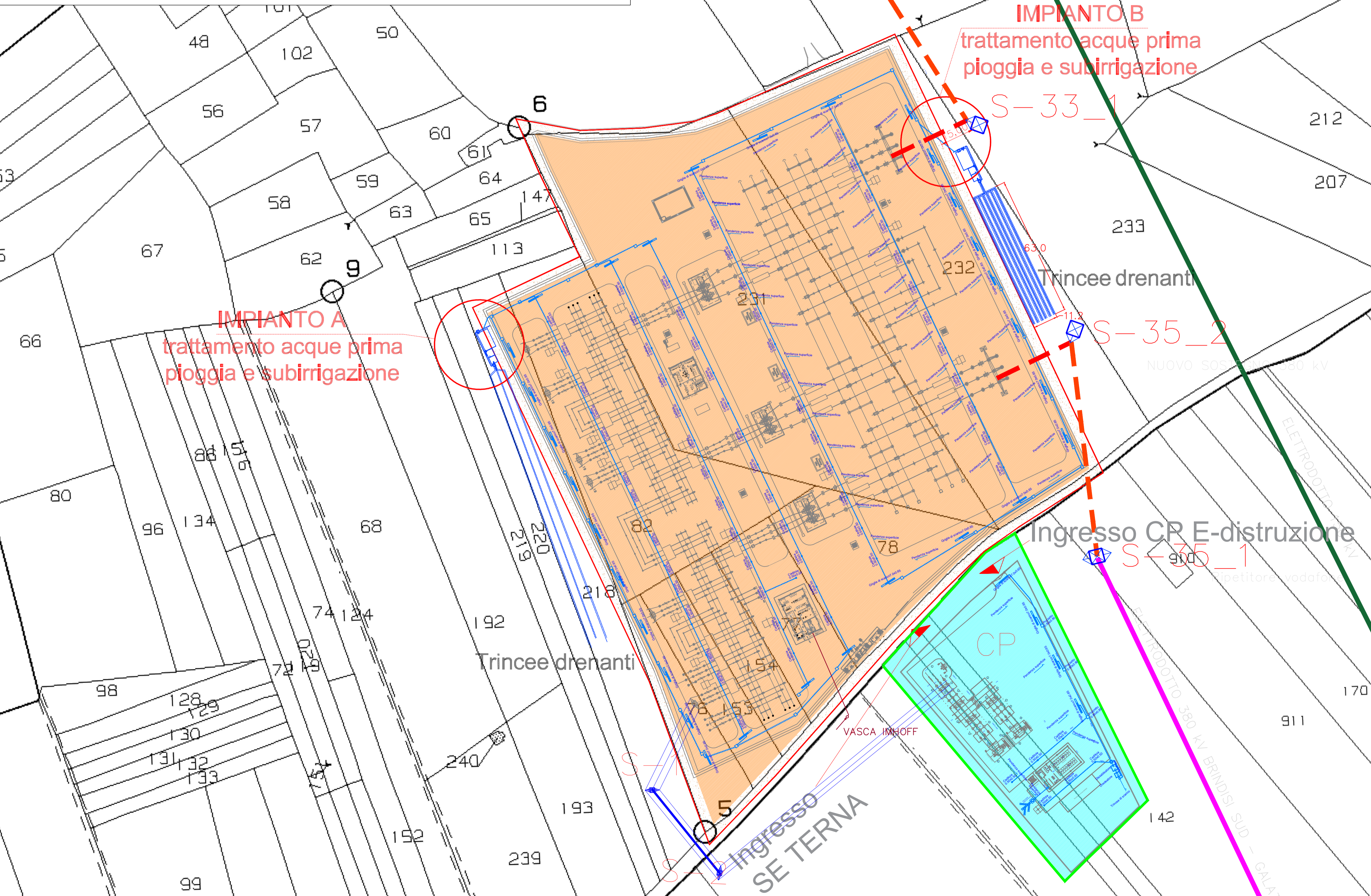
IMPIANTO TRATTAMENTO ACQUE PRIMA PIOGGIA E SUBIRRIGAZIONE
