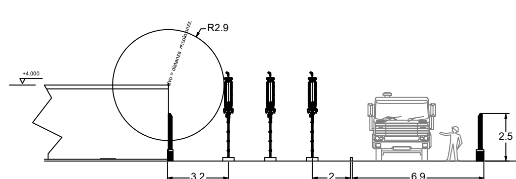
SEZIONE C-C - Scala 1:100
