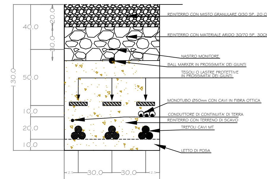
SEZIONE "S3"
