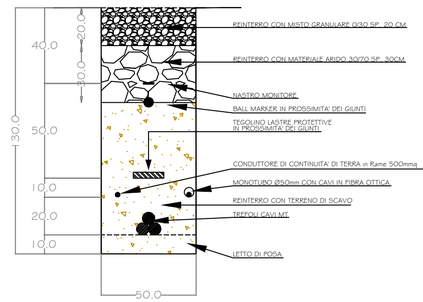
SEZIONE "S1"
