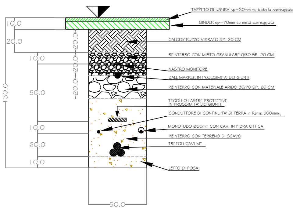
SEZIONE "A1"
