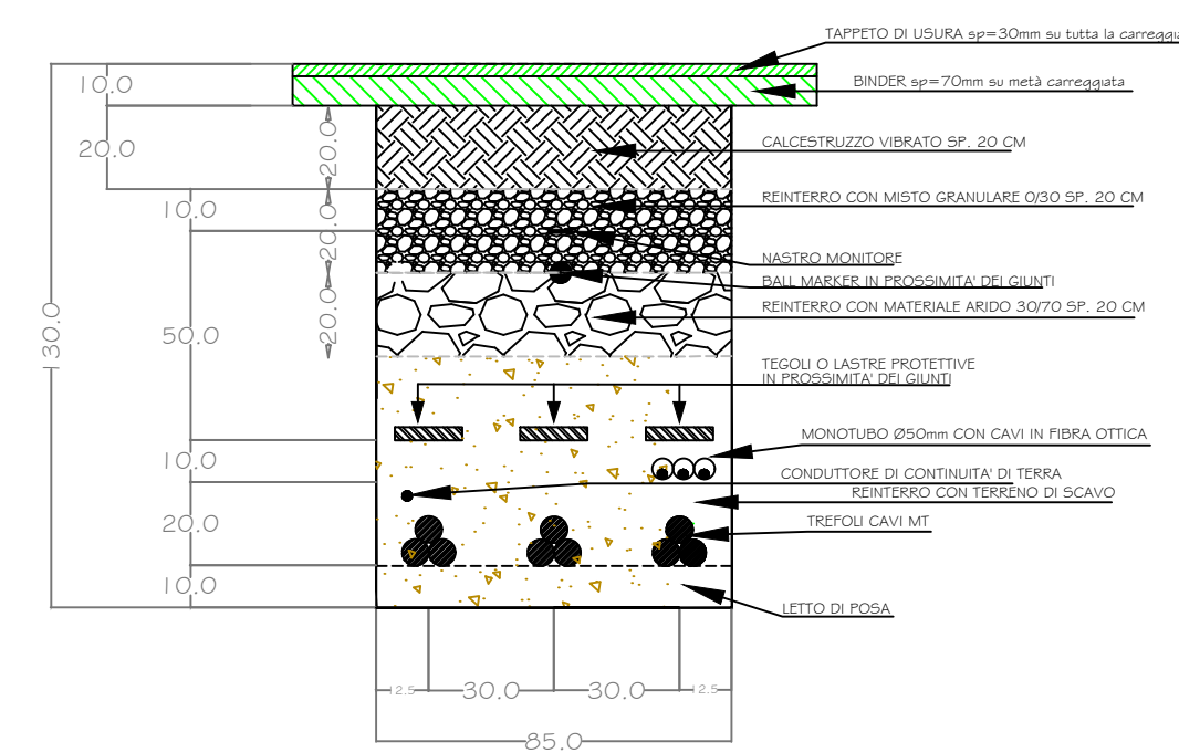
SEZIONE "A3"
