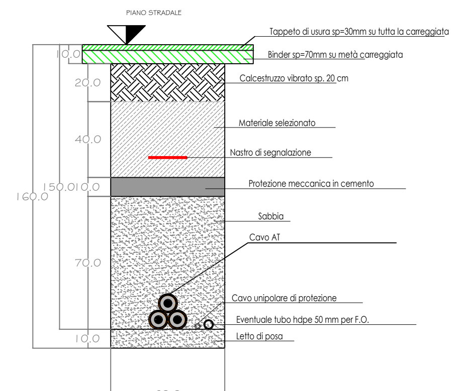
SEZIONE "A1"
