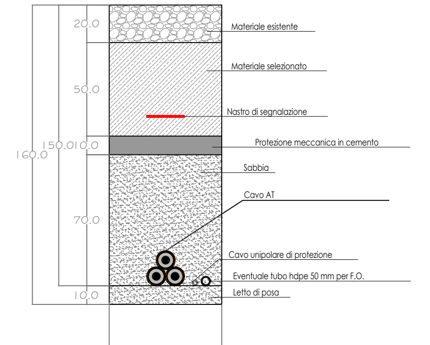
SEZIONE "T1"
