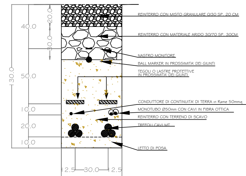
SEZIONE "S2"
