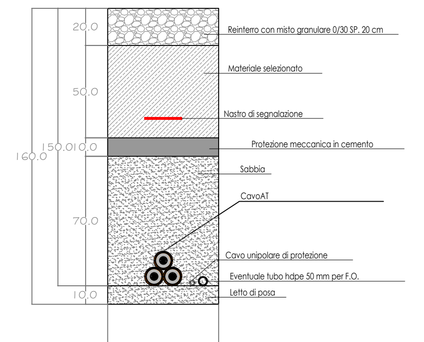
SEZIONE "S1"
