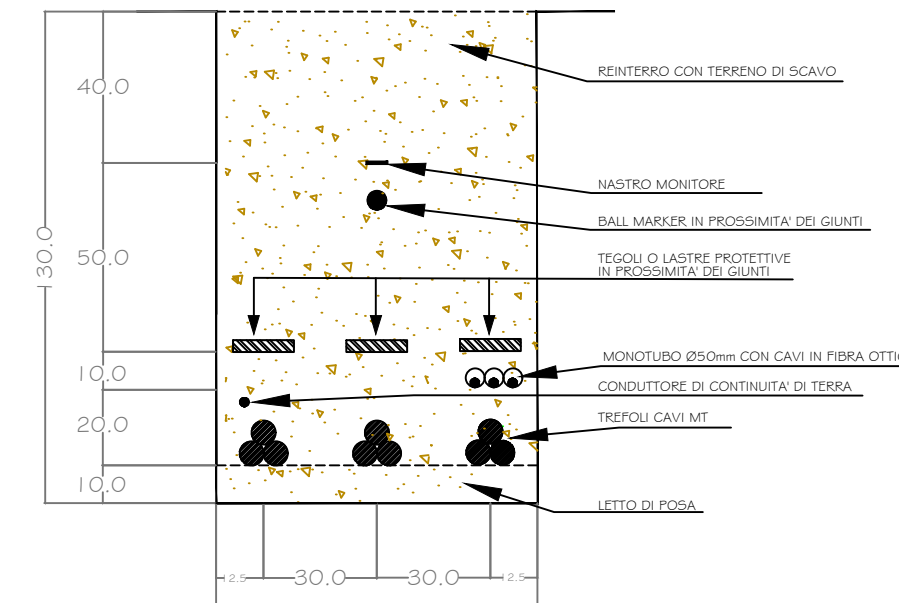
SEZIONE "T3"
