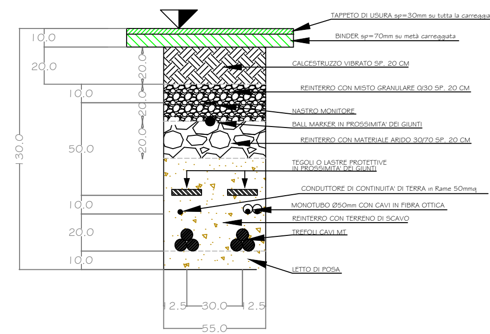
SEZIONE "A2"
