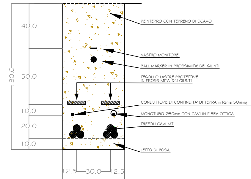
SEZIONE "T2"
