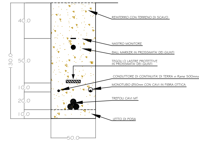
SEZIONE "T1"
