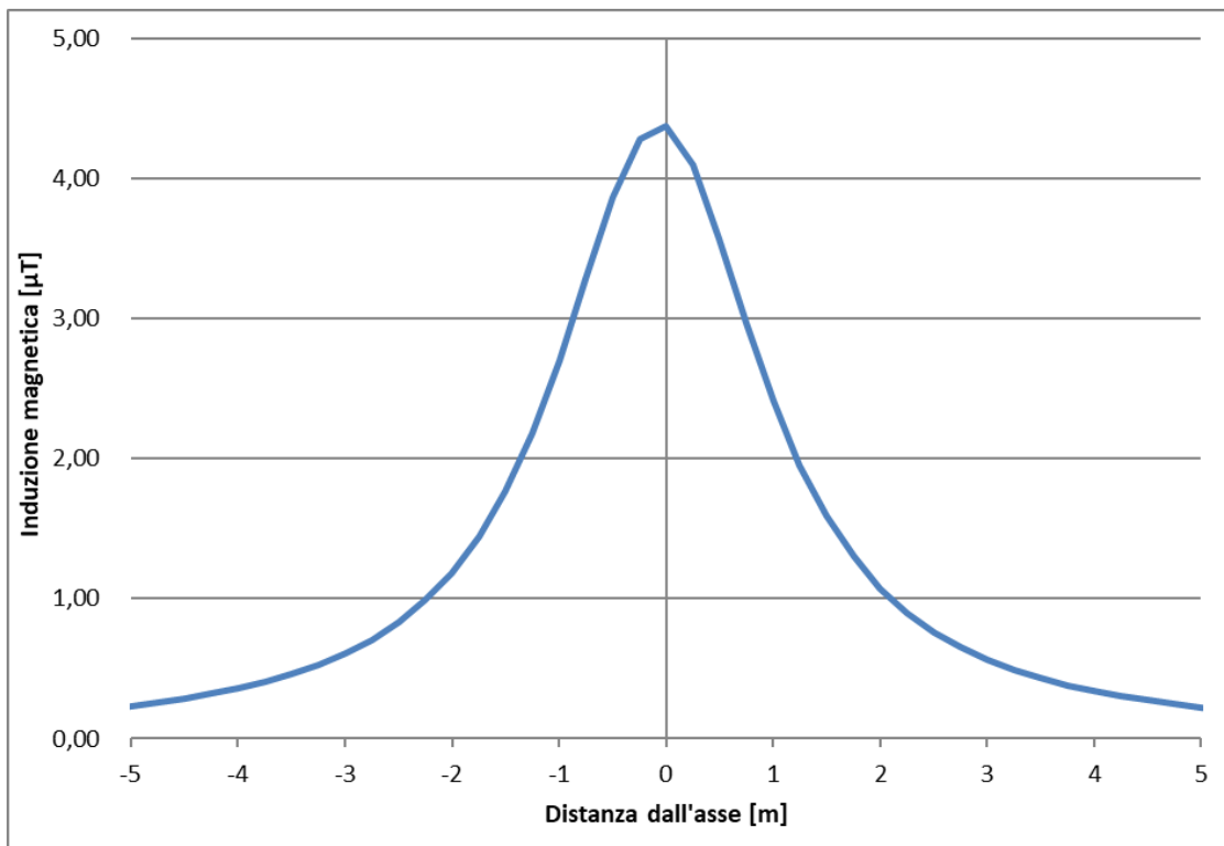
Figura 5-9 – Andamento campo magnetico – Sezione 8
