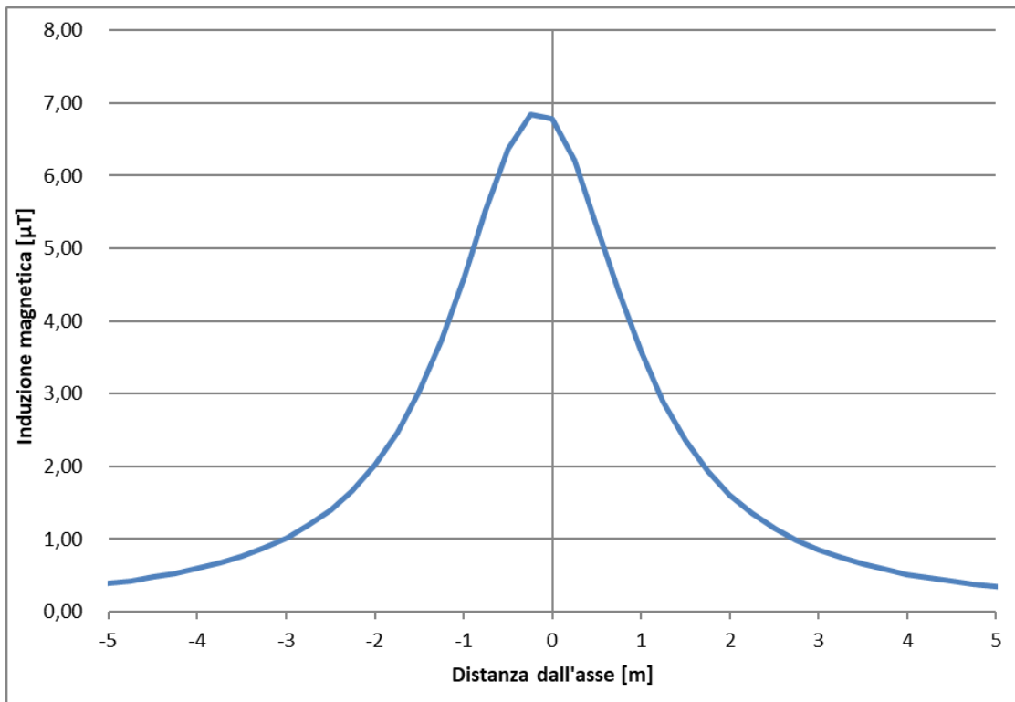
Figura 5-7 – Andamento campo magnetico – Sezione 6
