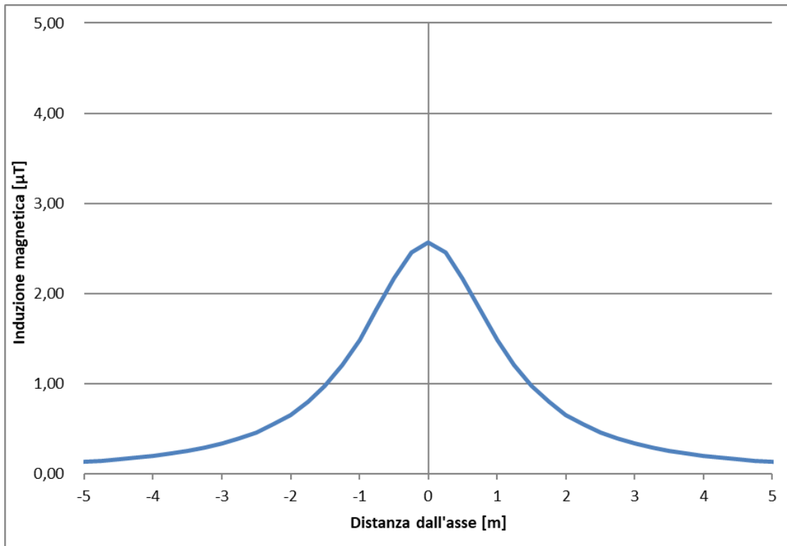
Figura 5-6 – Andamento campo magnetico – Sezione 5
