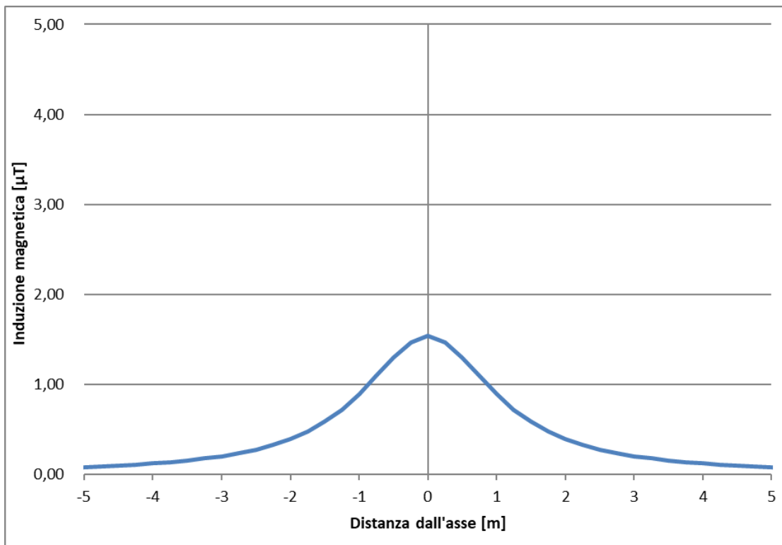
Figura 5-4 – Andamento campo magnetico – Sezione 3
