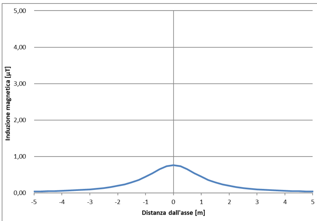
Figura 5-2 – Andamento campo magnetico – Sezione 1
