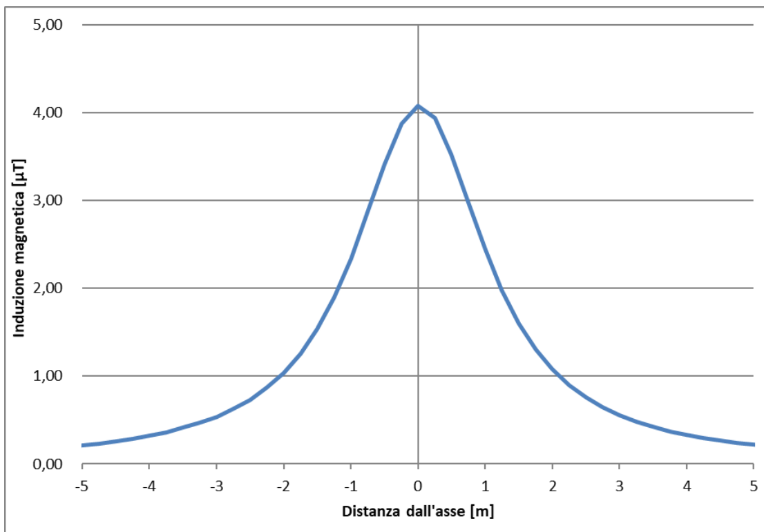
Figura 5-5 – Andamento campo magnetico – Sezione 4
