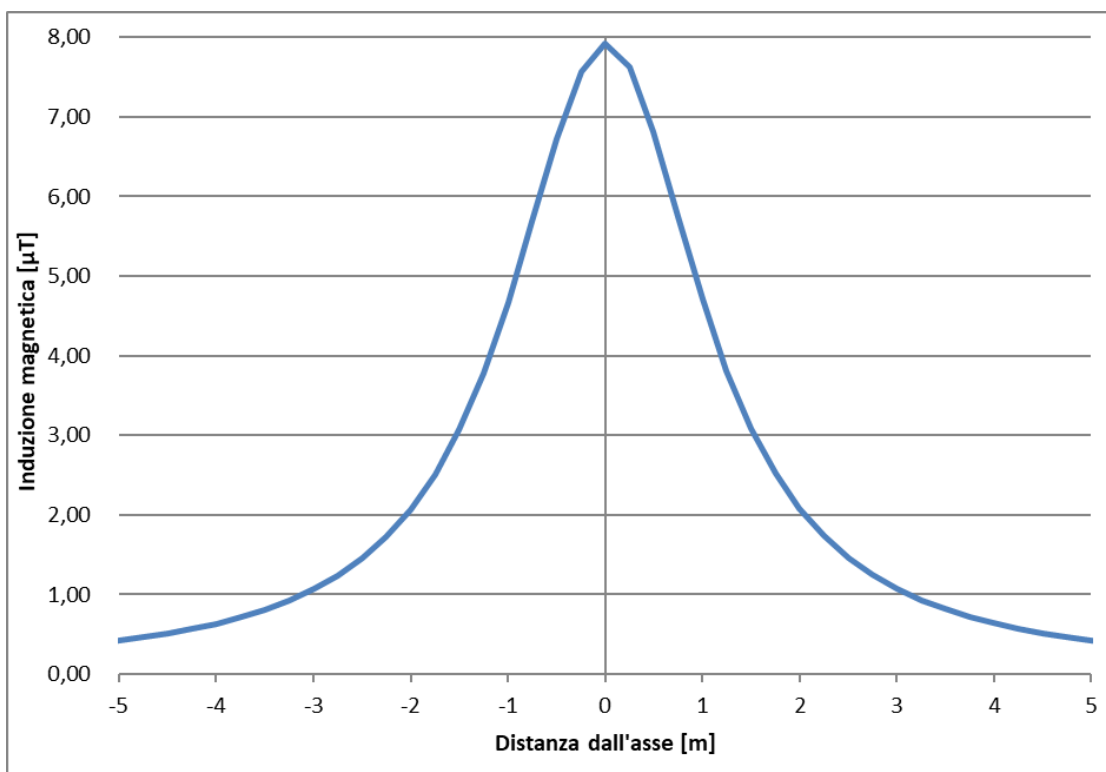
Figura 5-12 – Andamento campo magnetico – Sezione 11
