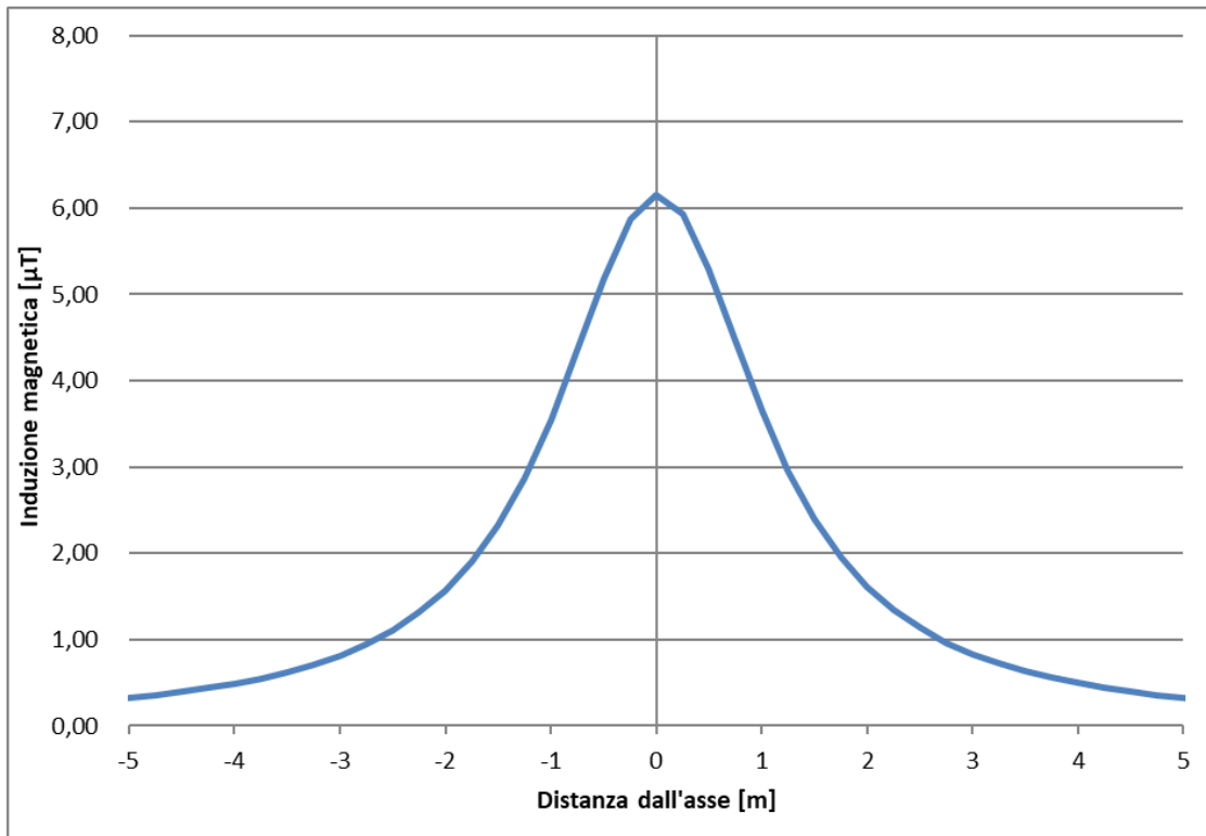
Figura 5-8 – Andamento campo magnetico – Sezione 7
