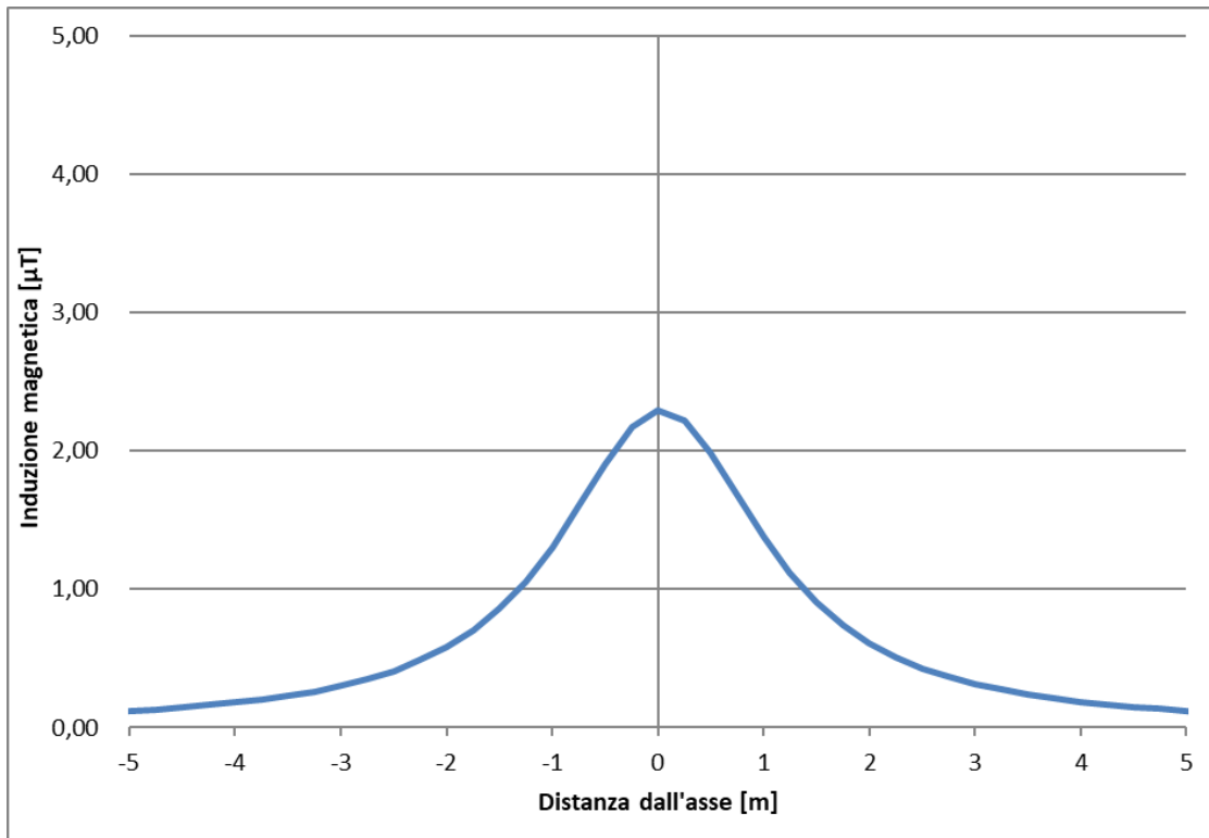
Figura 5-10 – Andamento campo magnetico – Sezione 9
