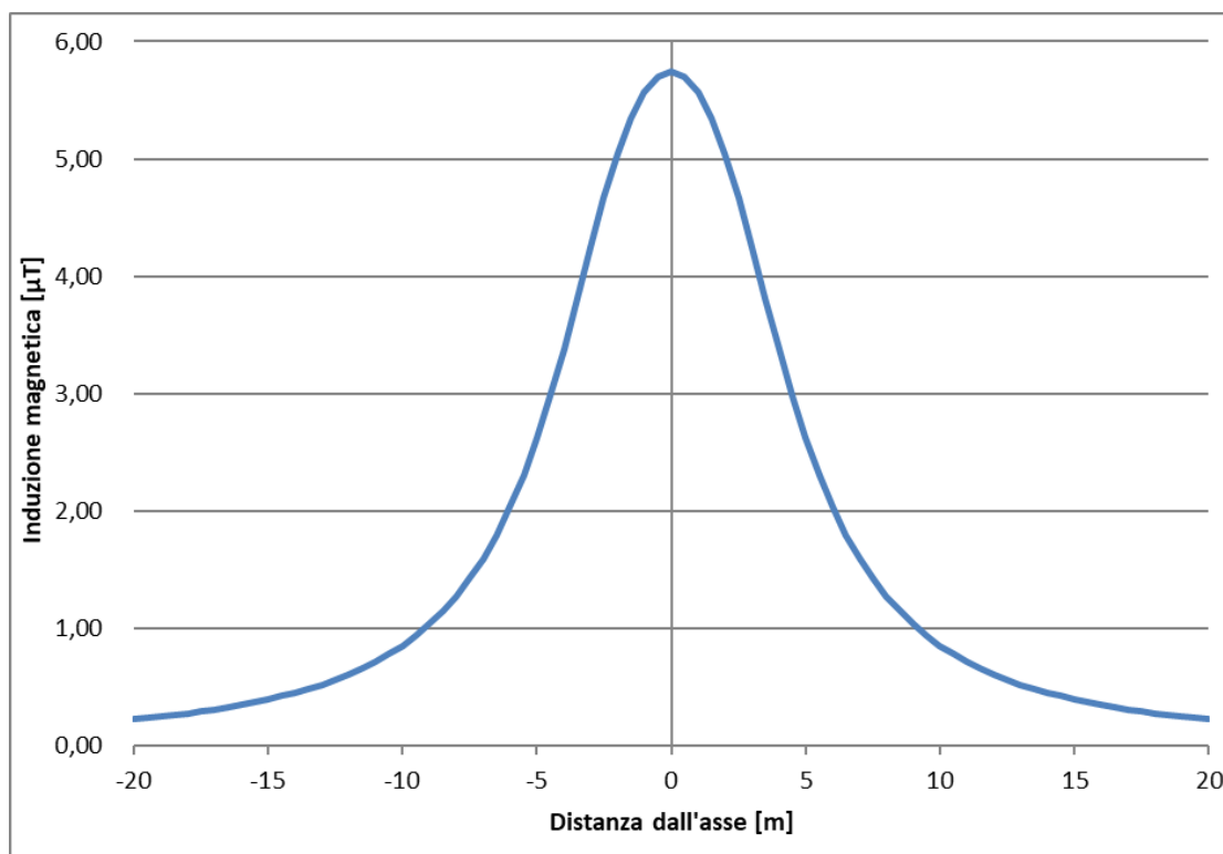
Figura 5-15 – Andamento campo magnetico sbarre AT stazione utente
