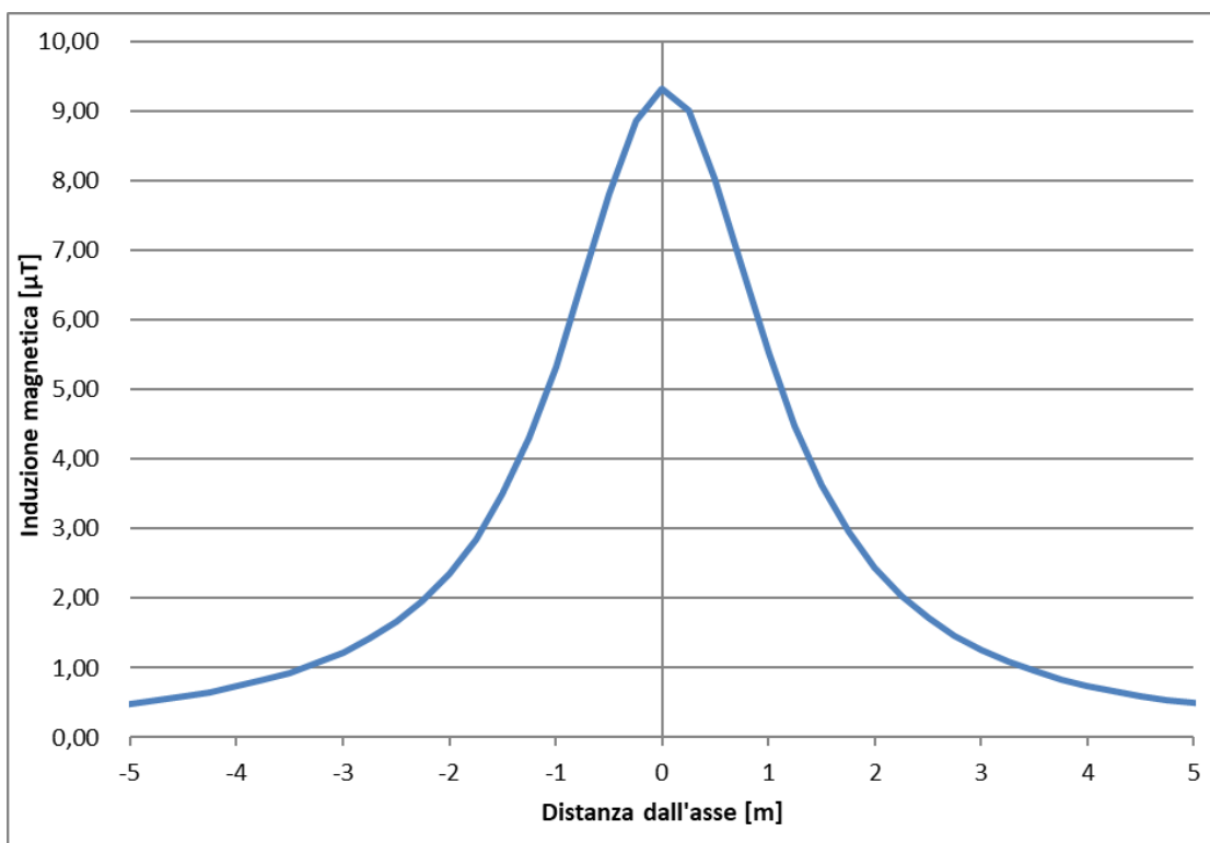
Figura 5-13 – Andamento campo magnetico – Sezione 12
