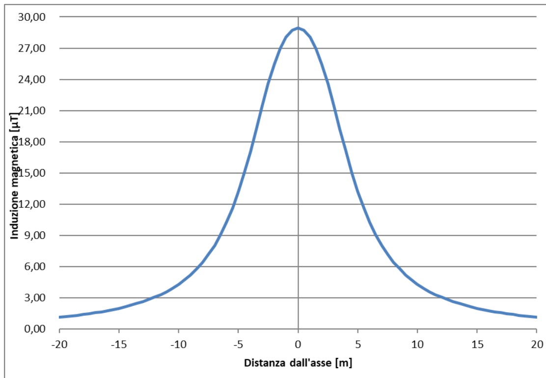
Figura 5-16 – Andamento campo magnetico sbarre AT stazione utente
