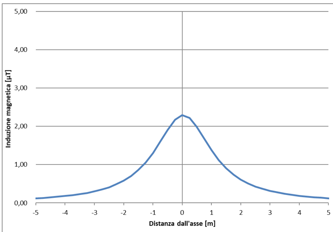
Figura 5-3 – Andamento campo magnetico – Sezione 2
