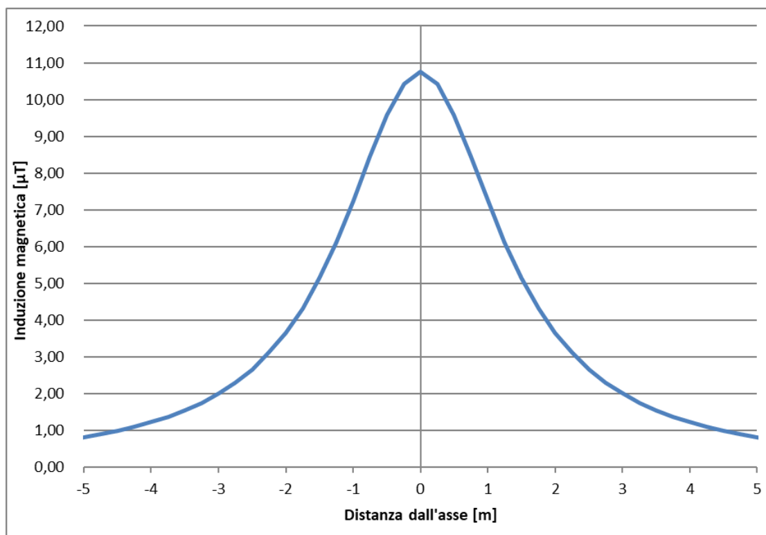
Figura 5-14 – Andamento campo magnetico – Sezione 13
