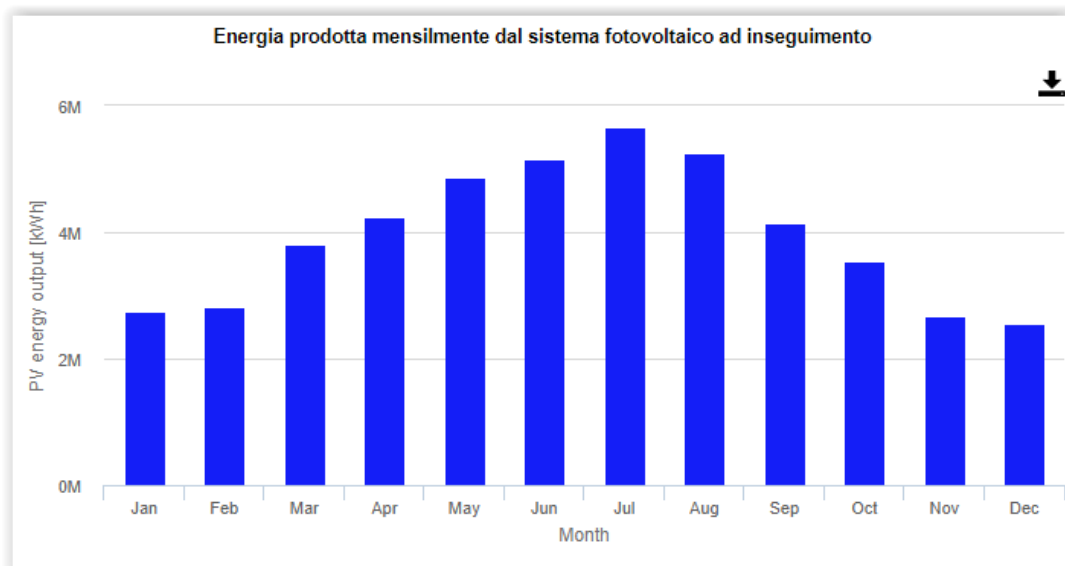
Fig. 7. Grafico rendimento energetico mensile dell'impianto interessato
