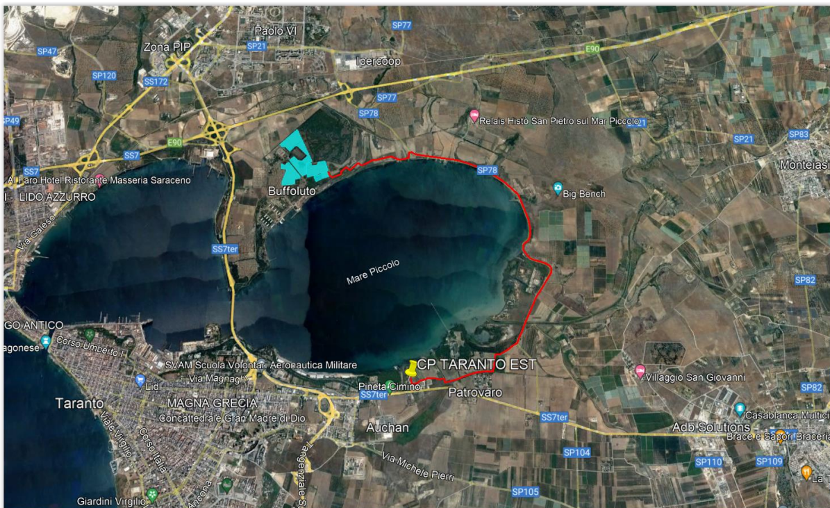
Fig. 4. Planimetria su ortofoto del progettato impianto Fotovoltaico: in ciano è riportata l’area del generatore fotovoltaico; in rosso è indicato l’elettrodotto dorsale MT di collegamento tra il generatore e la SSE Utente; a sud vi è indicata la CP “TARANTO EST” alla quale si collegherà la SSE Utente, accanto alla quale si prevede il posizionamento della SSE Utente e dello Storage
