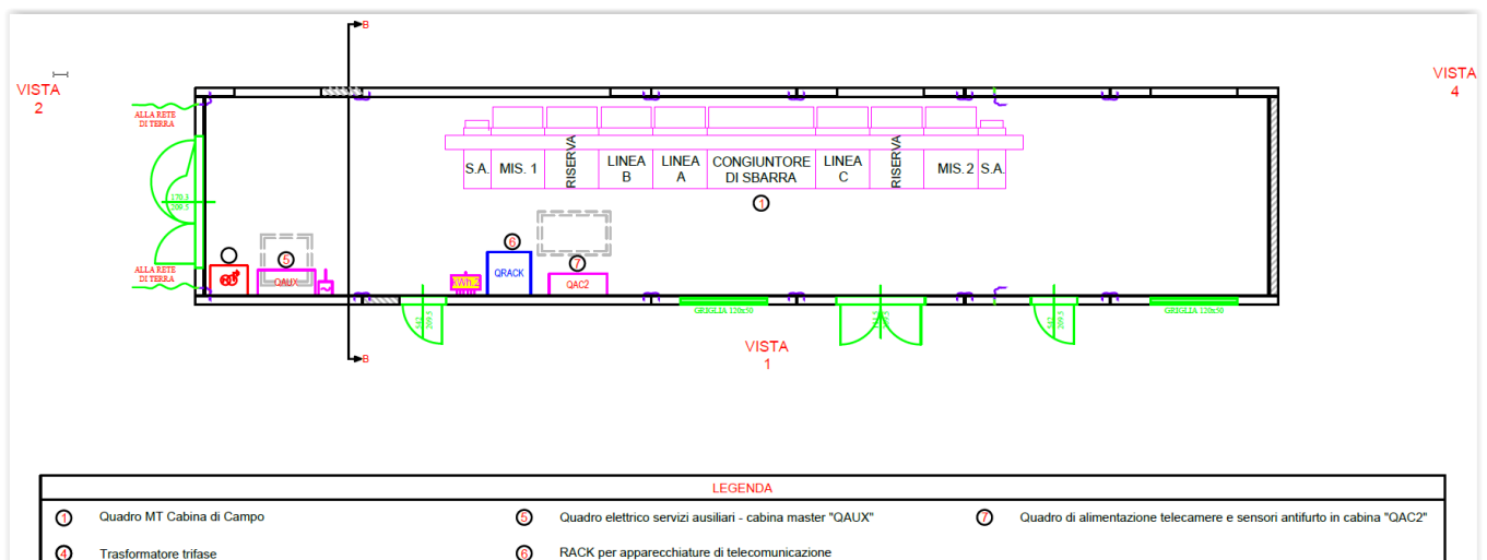
Fig. 20. Tipico Pianta della Cabina di Raccolta: locale destinato a soli Quadri MT (dimensioni principali 15,00 x 3,00 x 4,50h).
