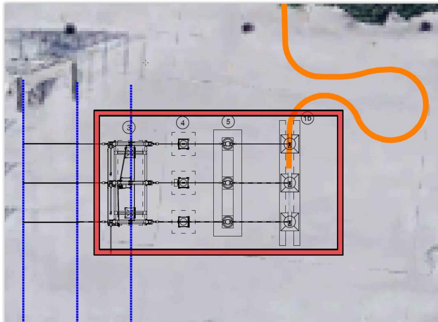
Fig. 33. Stralcio planimetrico dello stallo in area Cabina Primaria Enel
