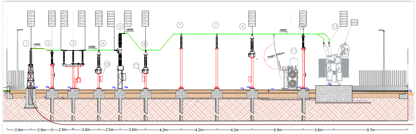
Fig. 29. Sezione elettromeccanica delle apparecchiature nella SSE Produttore
