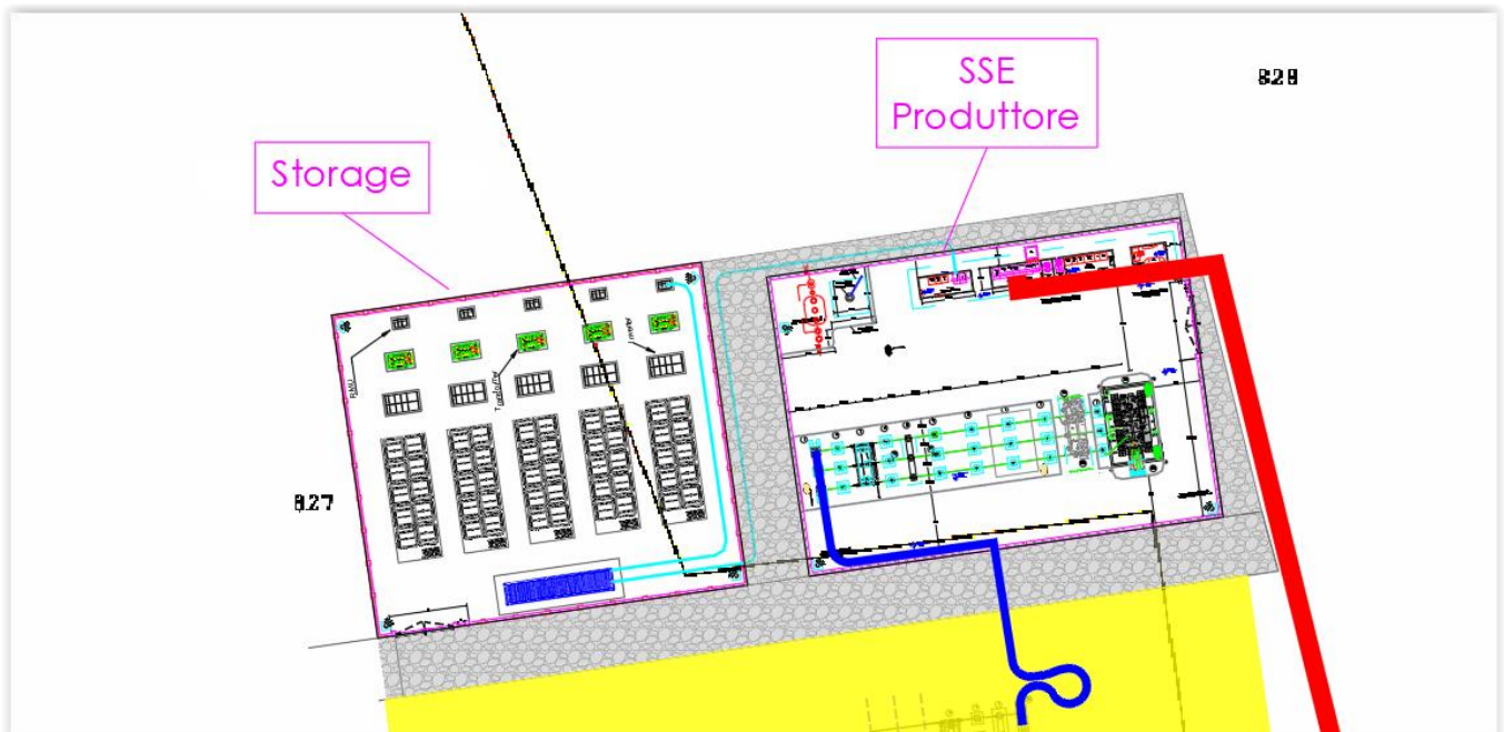
Fig. 42. Layout della Stazione di accumulo, su planimetria catastale, e posizione reciproca rispetto alla futura SSE Produttore
