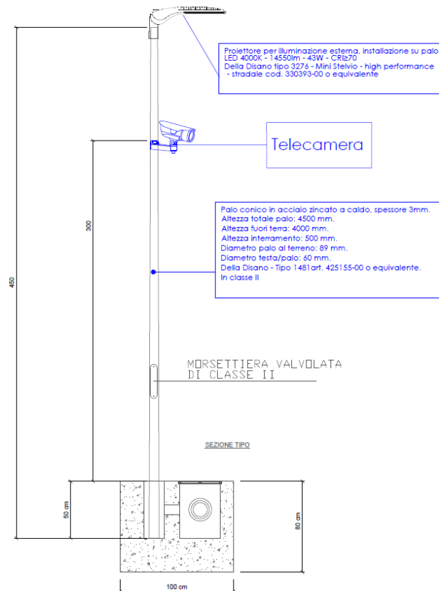
Fig. 46. Installazione telecamera su palo preposto.
