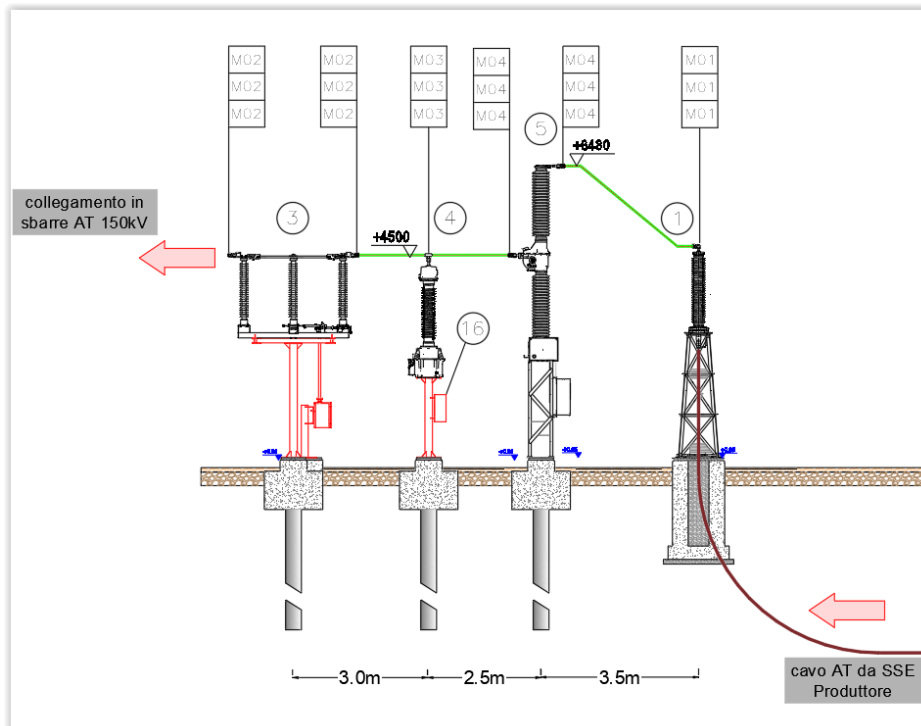
Fig. 34. Sezione elettromeccanica dello stallo in area Cabina Primaria Enel
