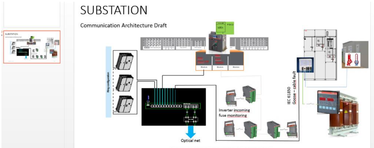
Fig. 47. Architettura del sistema di supervisione e controllo
