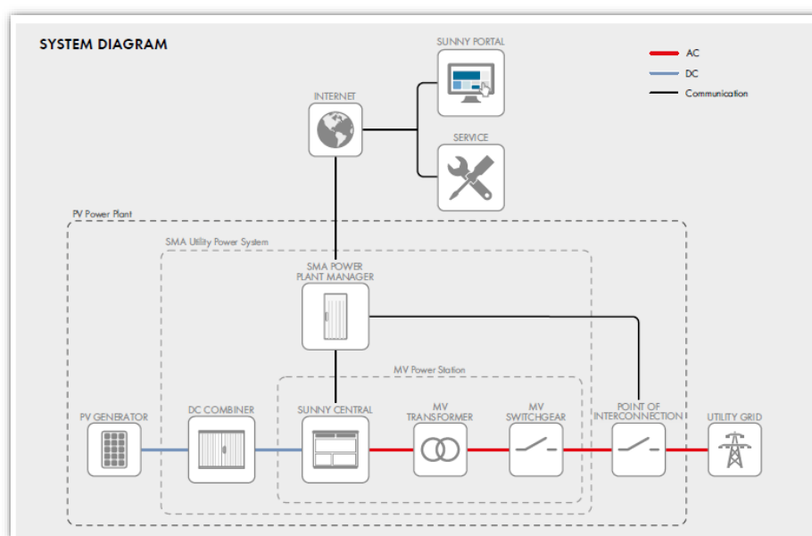
Fig. 15. Schema di collegamento al Sunny Central, dal lato Generatore e dal lato RTN.
