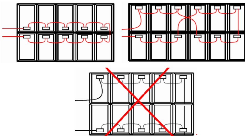
Fig. 49. Estratto dalla guida tecnica CEI 82-25 relativa alla modalità di cablaggio di stringa.
