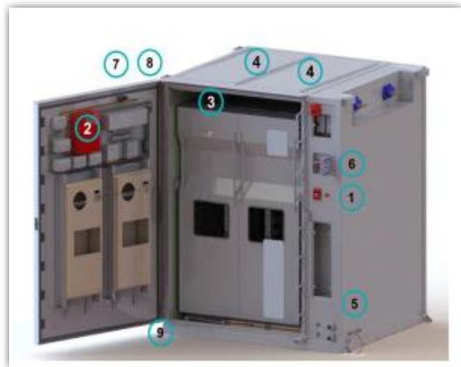
Fig. 39. Esempio Modulo batterie
