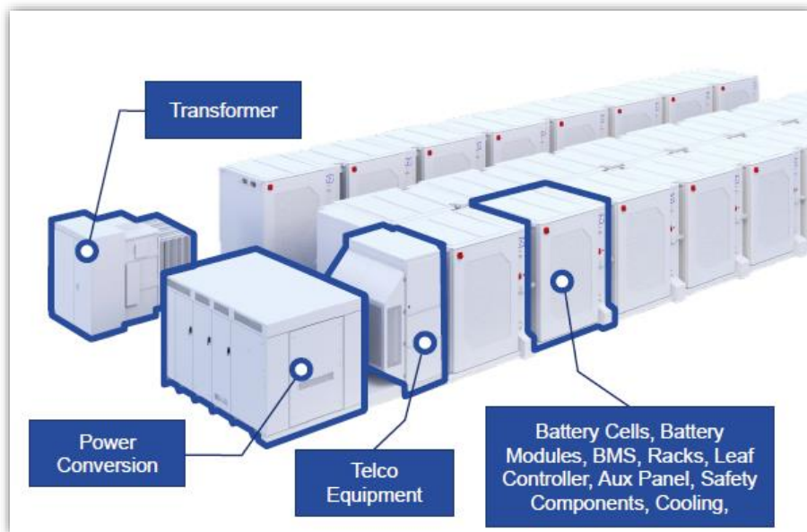
Fig. 41. Layout del sistema costituito da moduli batterie
