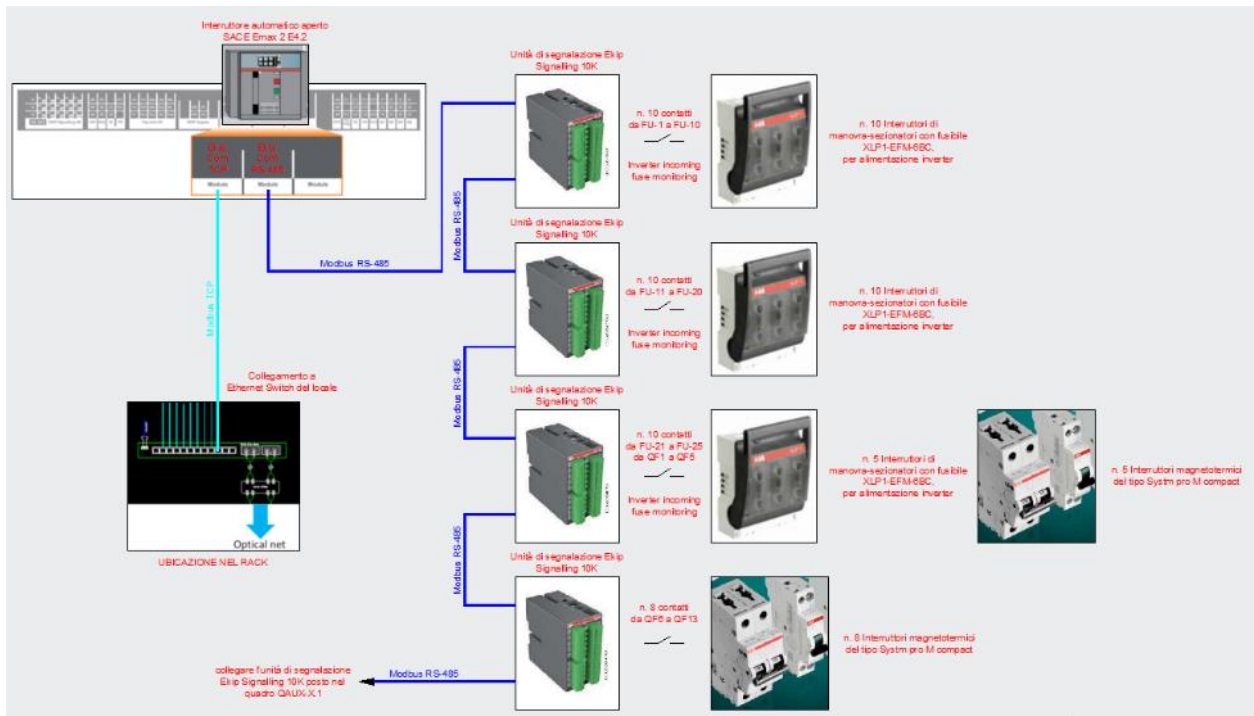
Fig. 48. Architettura del sistema di supervisione e controllo bt
