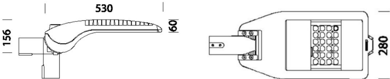
Fig. 45. Tipico apparecchio Illuminante a LED da montaggio a parete.
