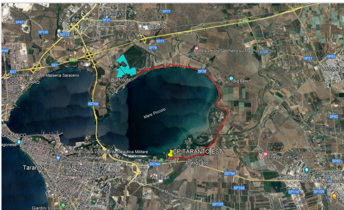
Fig. 2. Planimetria su ortofoto del progettato impianto Fotovoltaico: in ciano è riportata l'area del generatore fotovoltaico; in rosso è indicato l'elettrodotto dorsale MT di collegamento tra il generatore e la SSE Utente; a
