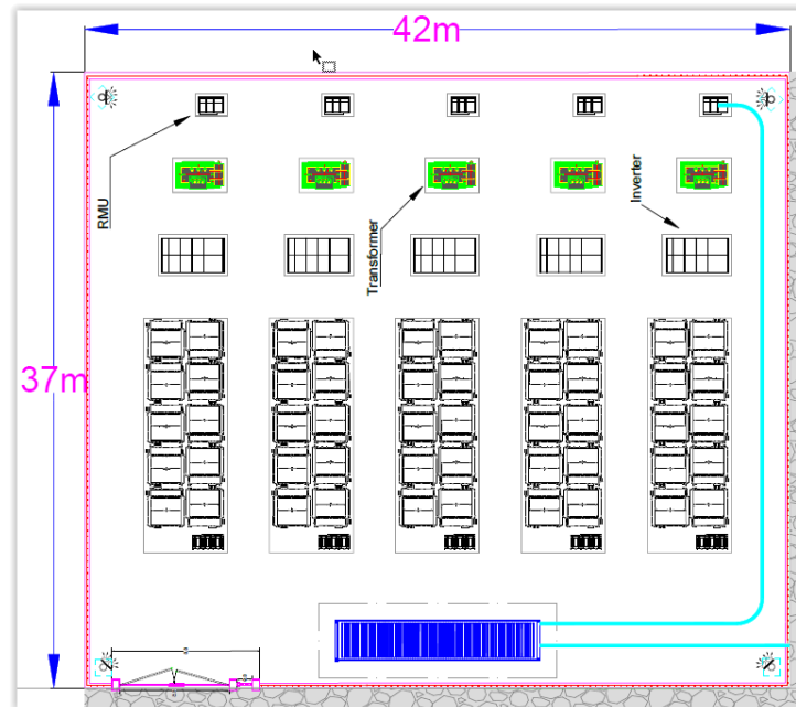
Fig. 43. Planimetria della Stazione di Accumulo con individuazione dei componenti principali
