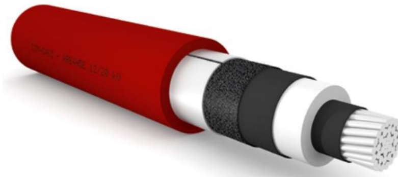
Fig. 22. Particolare degli strati costitutivi di un cavo MT ARE4H5E.
