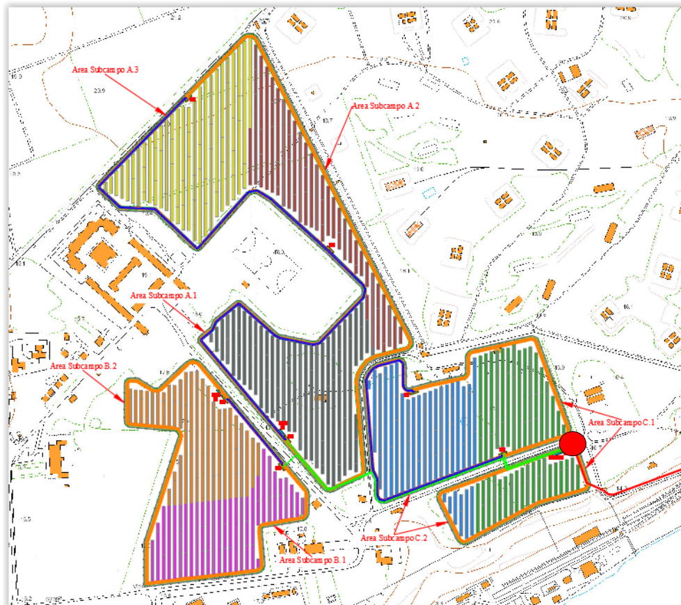
Fig. 6. Posizione della Cabina di raccolta contrassegnata con cerchio rosso; inoltre, vengono rappresentati tutti i subcampi con colori diversi
