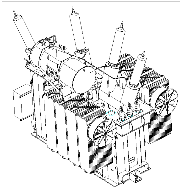
Fig. 25. Vista assonometrica del trasformatore di progetto
