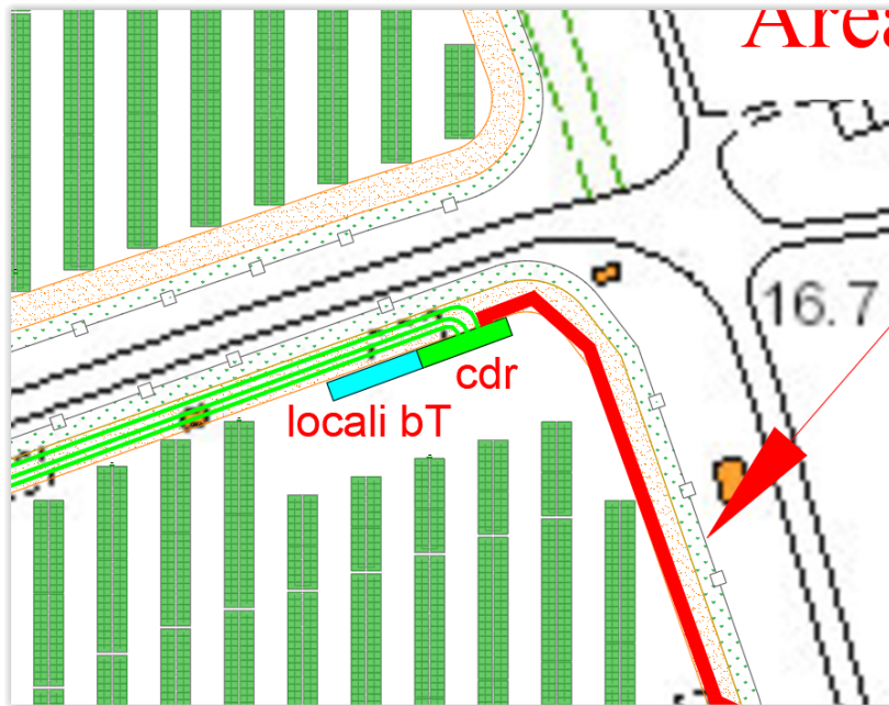
Fig. 7. Dettaglio della CdR: in verde le linee provenienti dai sottocampi; in rosso la linea dorsale verso la SSE.
