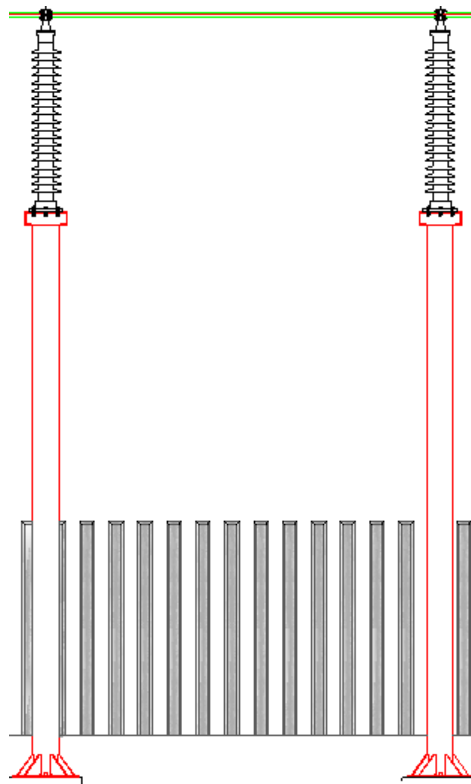
Fig. 23. Particolare prospettico dei supporti rompitratta unipolari
