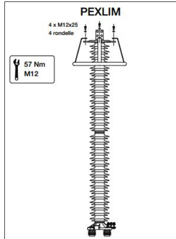
Fig. 19. Particolare di dettaglio dello scaricatore AT
