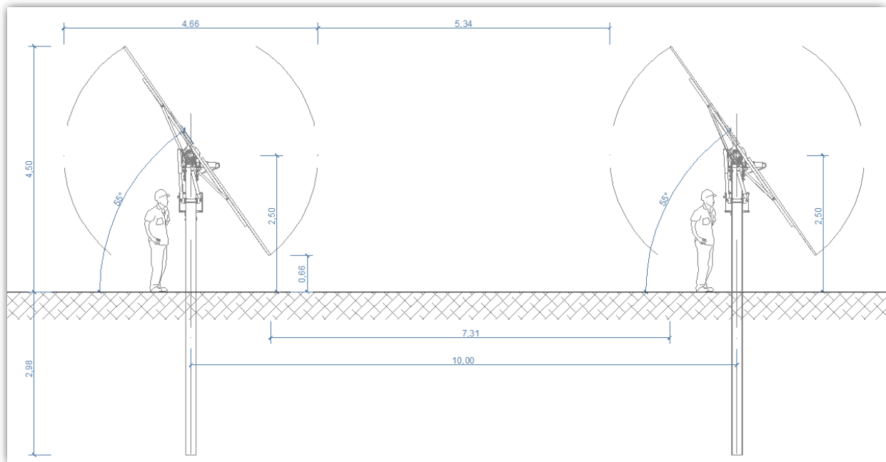
Fig. 3. Vista in sezione laterale del tracker-tipo, con altezze minime e massime raggiunte dai moduli nelle posizioni di estrema rotazione
