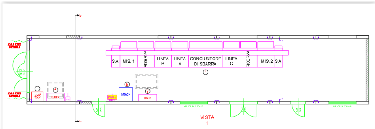
Fig. 8. Tipico PIANTA della Cabina di Raccolta: locale destinato a soli Quadri MT (dimensioni principali 15,00 x 3,00 x 4,50h).
