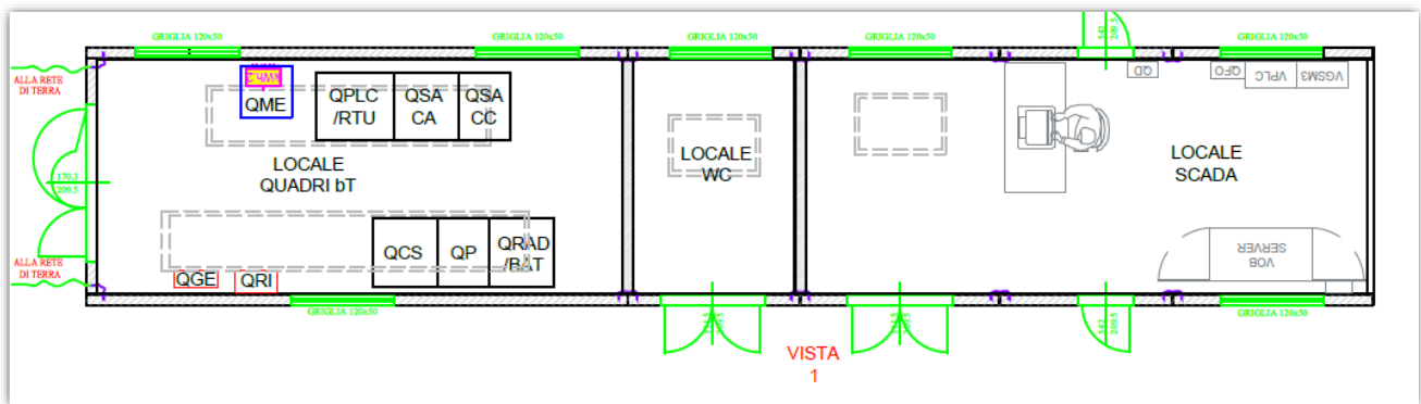
Fig. 9. Tipico Pianta locali bT (dimensioni principali 15,00 x 3,00 x 4,50h)
