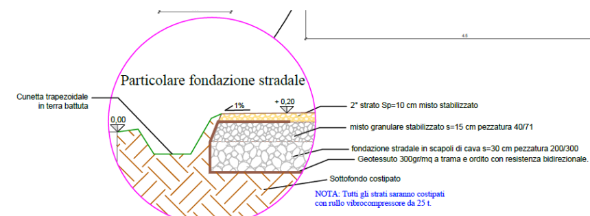
Fig. 10. Sezione tipo viabilità interna al parco
