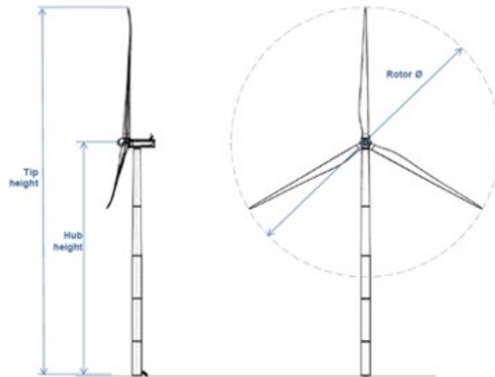
Figura 3-3: Vista e caratteristiche di un aerogeneratore da 6,0 MW
