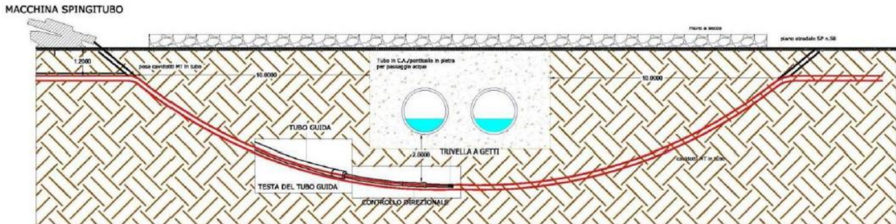
Figura 4. Schema tipo attraversamento interferenze in TOC
