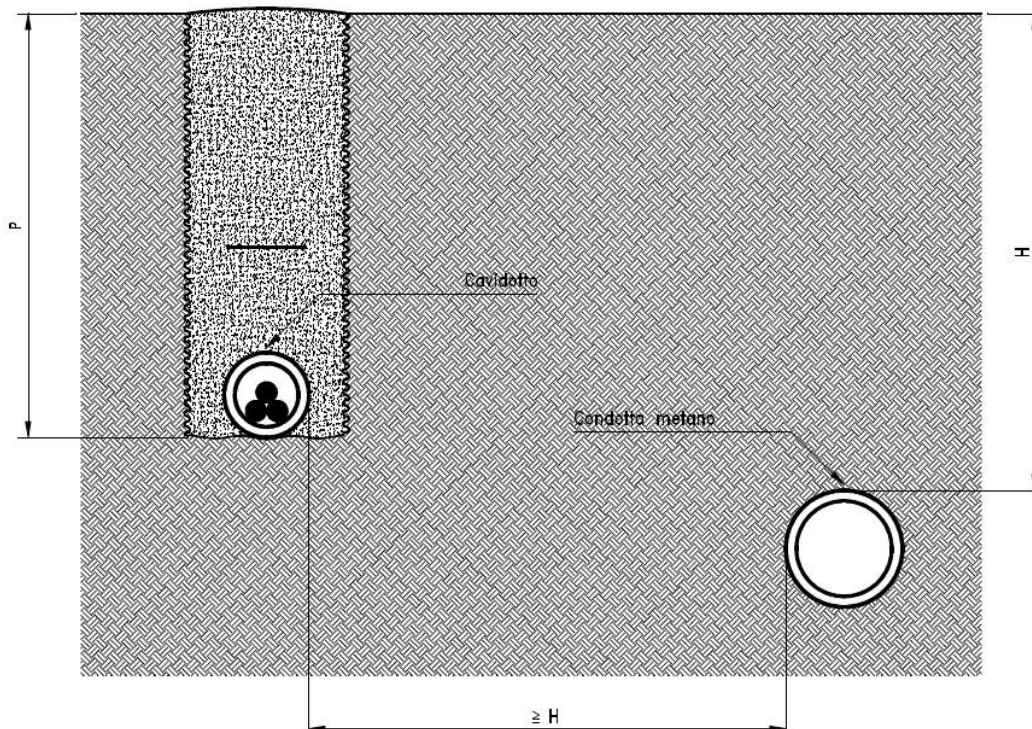
Figura 9 - Parallelismi con gasdotti - pressione gas >5 bar
