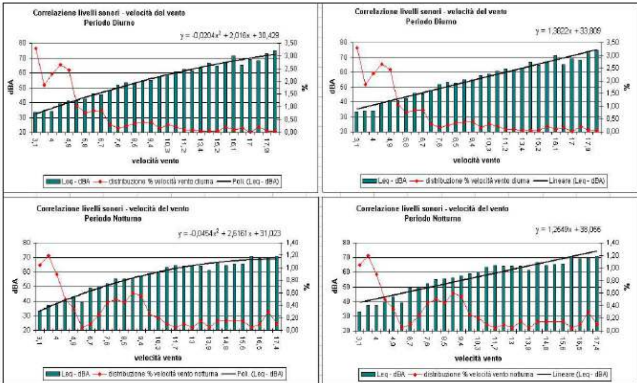
Figura 7_ Grafici di correlazione LAeq-vel. vento (TECNICOOP)
