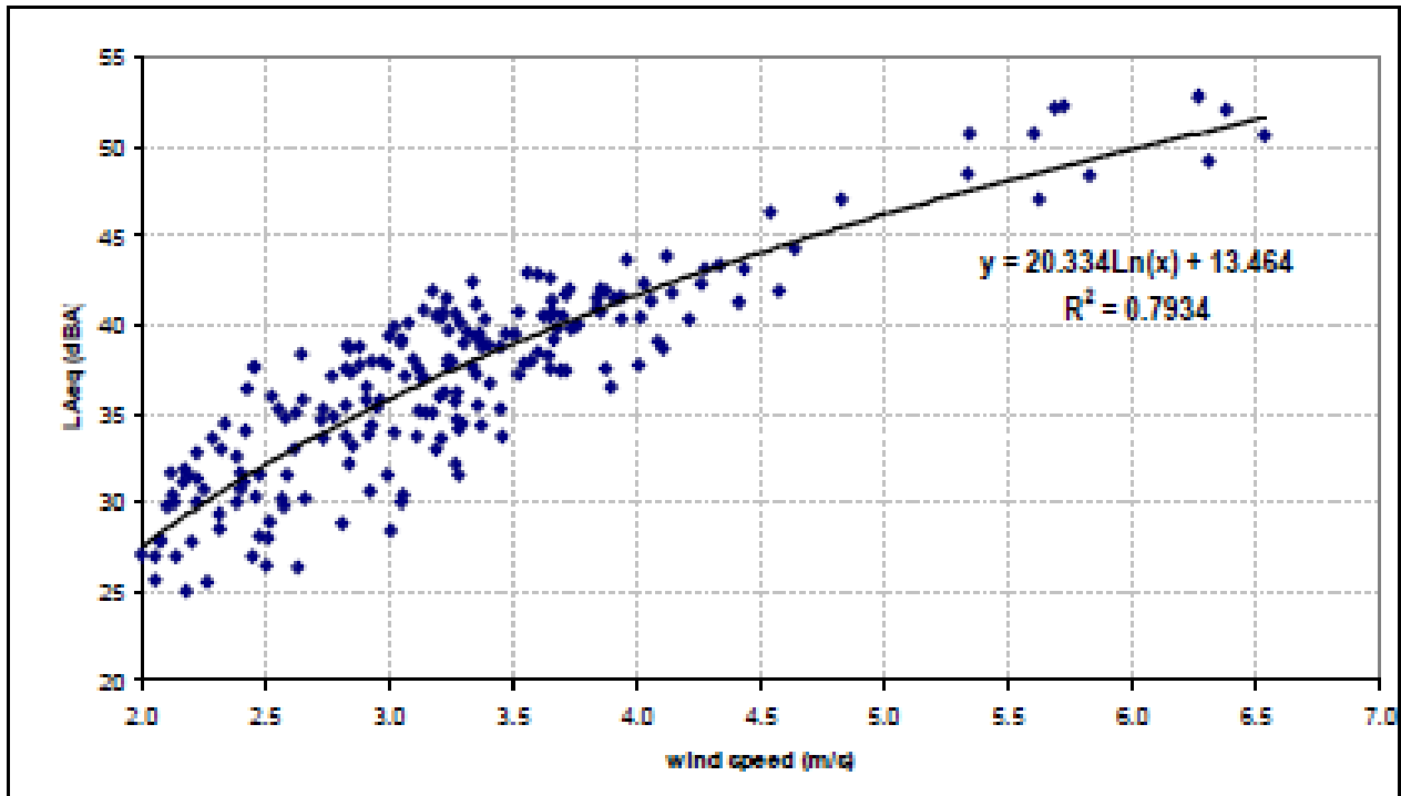
Figura 8_ Grafico di correlazione LAeq-vel. vento (ISPRA)
