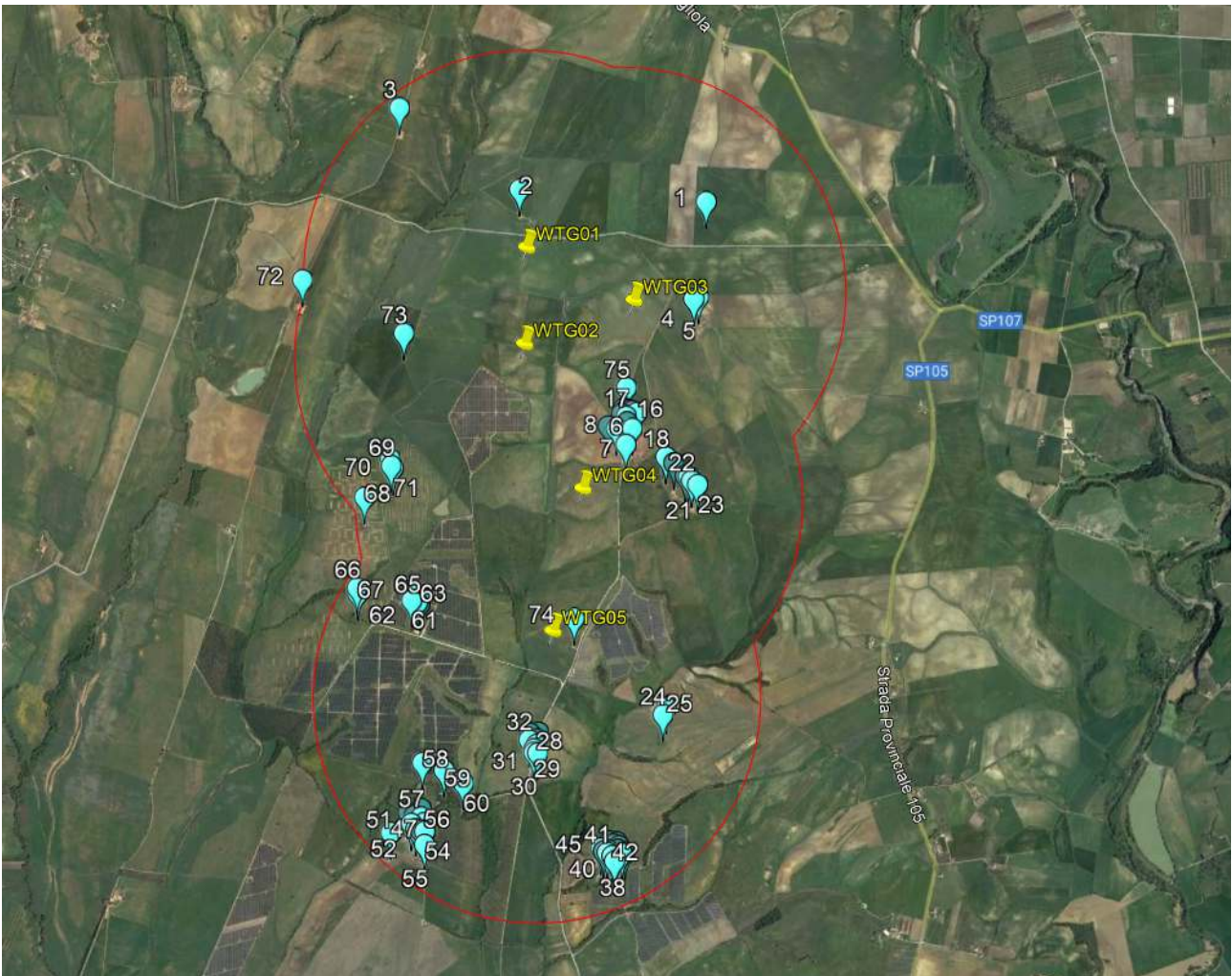
Figura 3_Localizzazione ricettori
