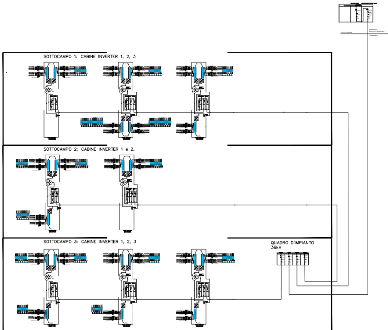
Figura 3 – Schema Elettrico Unifilare
