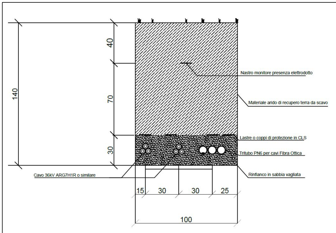
Figura 6 – Sezione tipo su terreno vegetale
