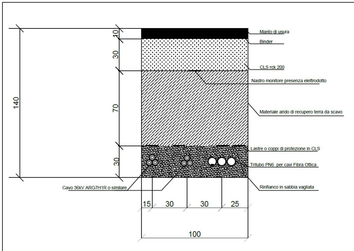
Figura 5 – Sezione tipo su manto stradale
