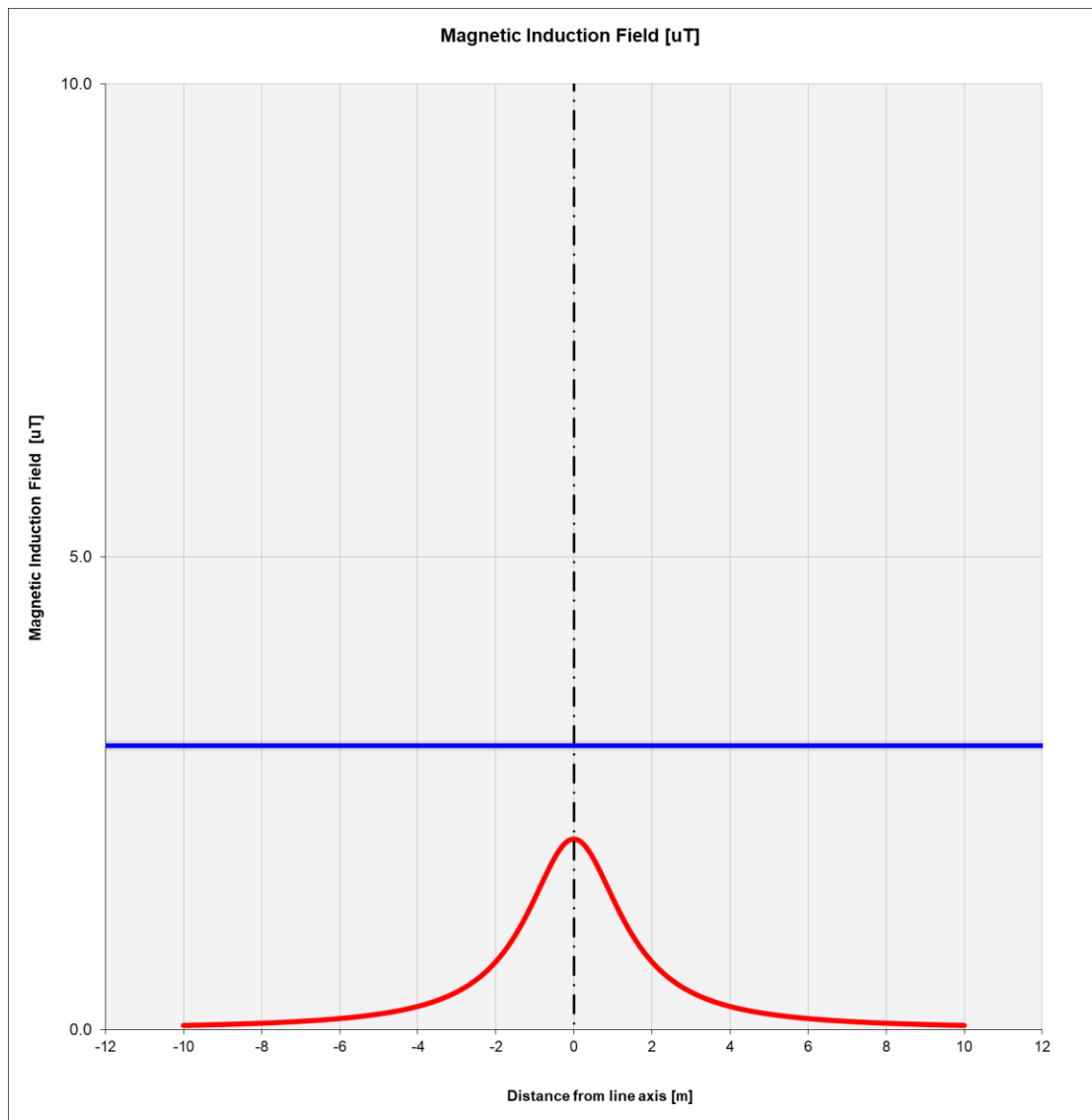
Figura 3: Andamento dell'induzione magnetica prodotta dalla linea in cavo per la sezione 1 (una terna a 36 kV)
