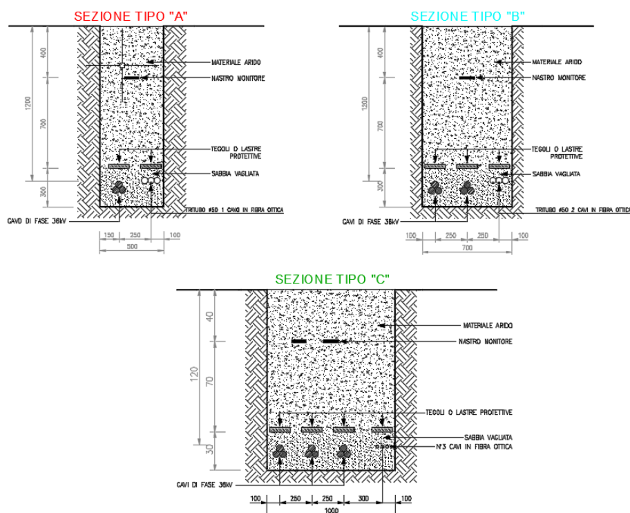
Figura 1: Sezioni tipiche di posa della linea in cavo su strade sterrate e terreno agricolo
