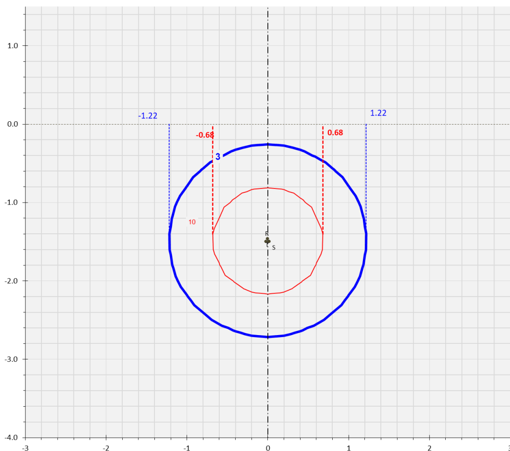
Figura 6: Curve di equilivello per il campo di induzione magnetica generato dalla linea AT (Sezione 1 – una terna AT)
