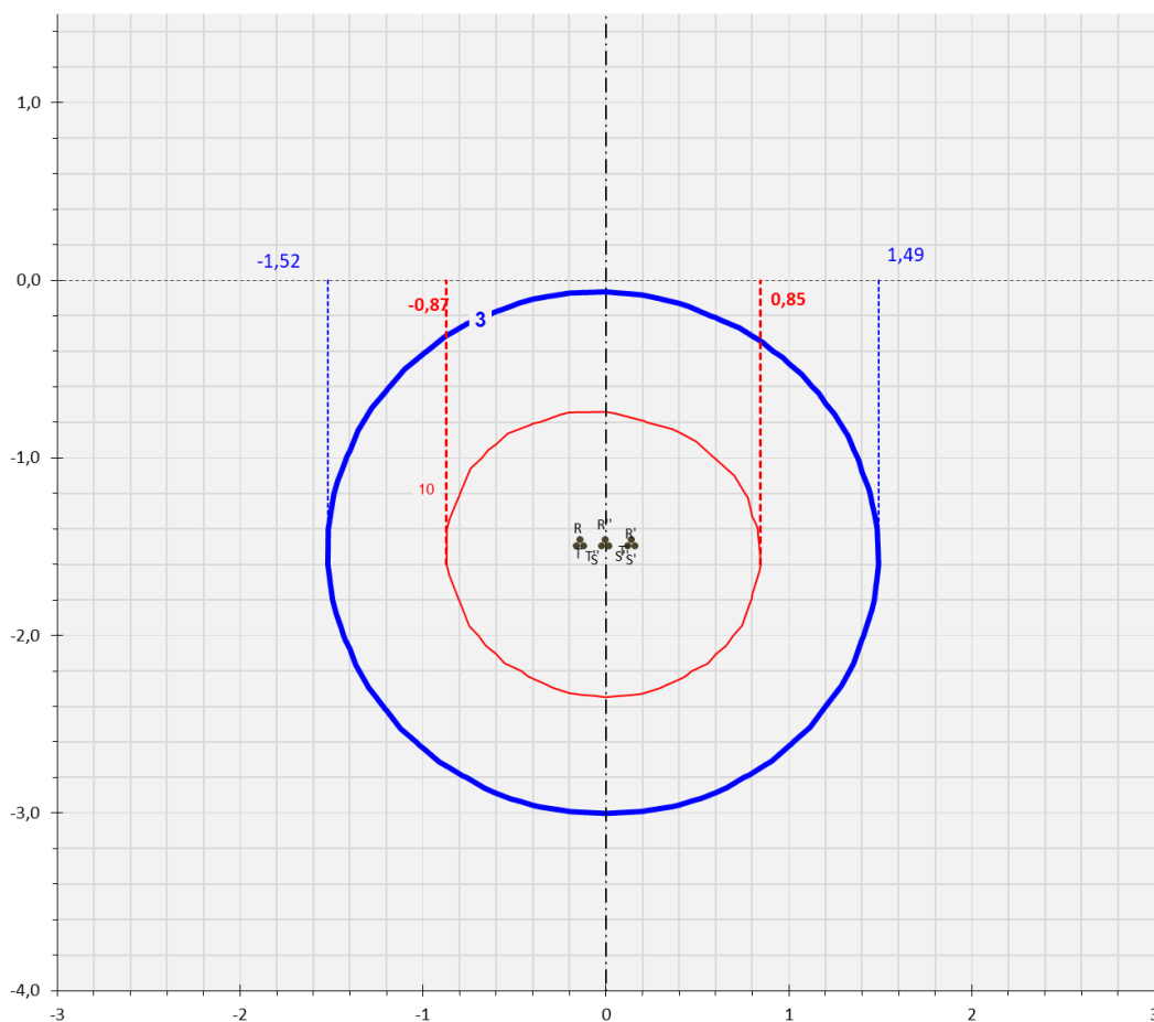
Figura 8: Curve di equilivello per il campo di induzione magnetica generato dalla linea (Sezione 3 – tre terne a 36 kV)
