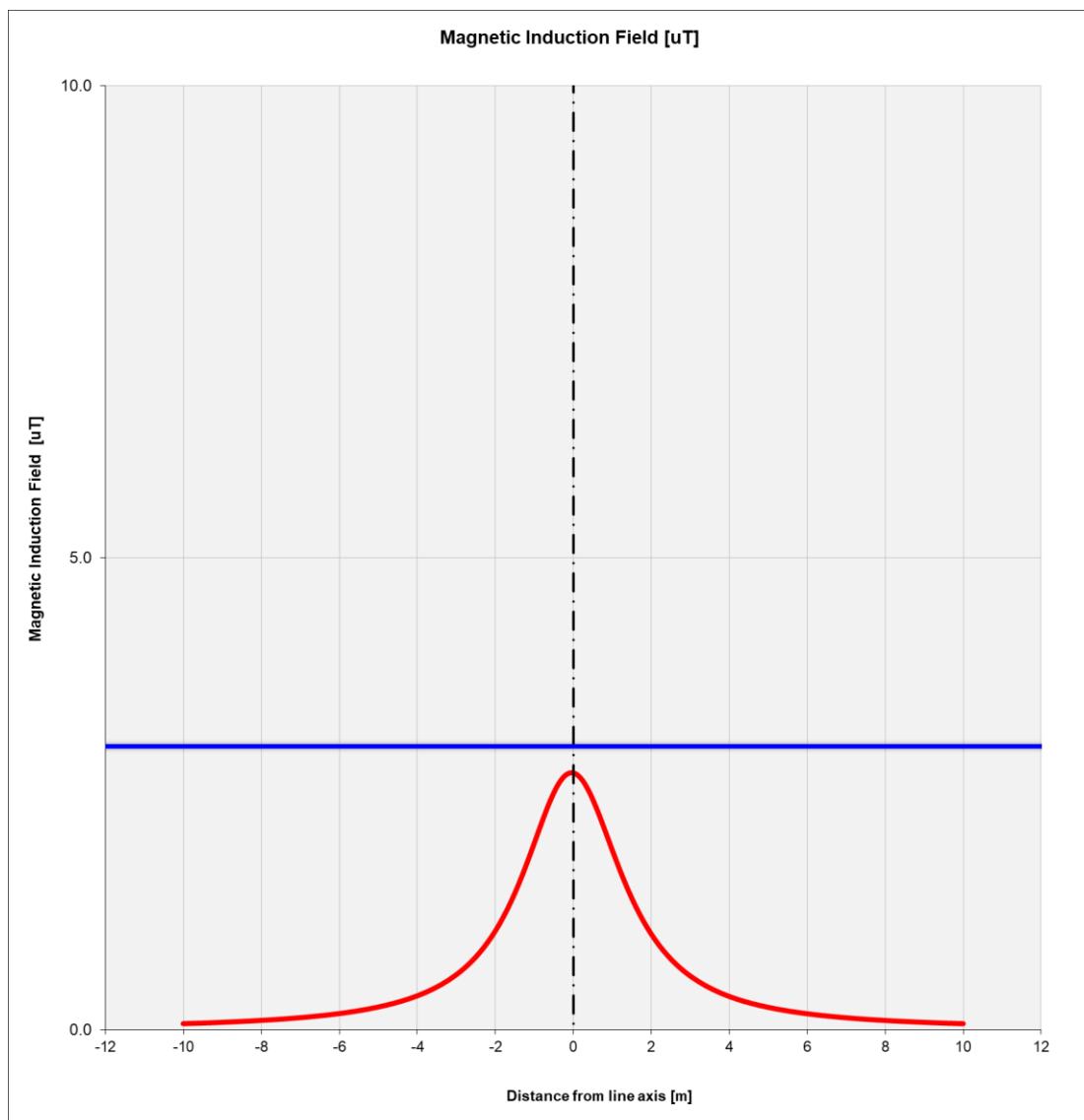
Figura 5: Andamento dell'induzione magnetica prodotta dalla linea in cavo per la sezione 3 (tre terne a 36 kV)
