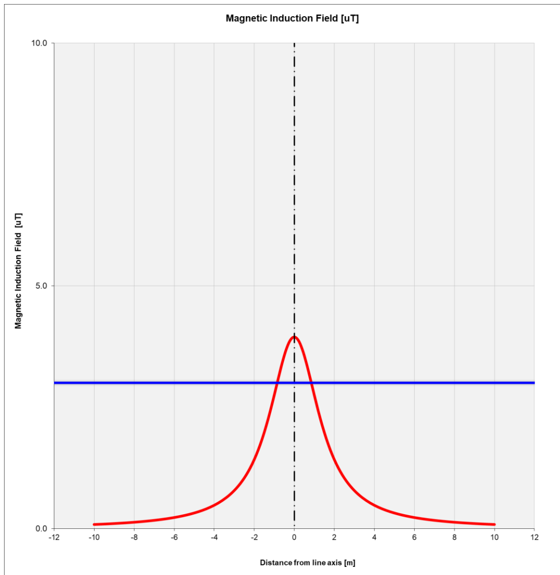
Figura 4: Andamento dell'induzione magnetica prodotta dalla linea in cavo per la sezione 2 (due terne a 36 kV)
