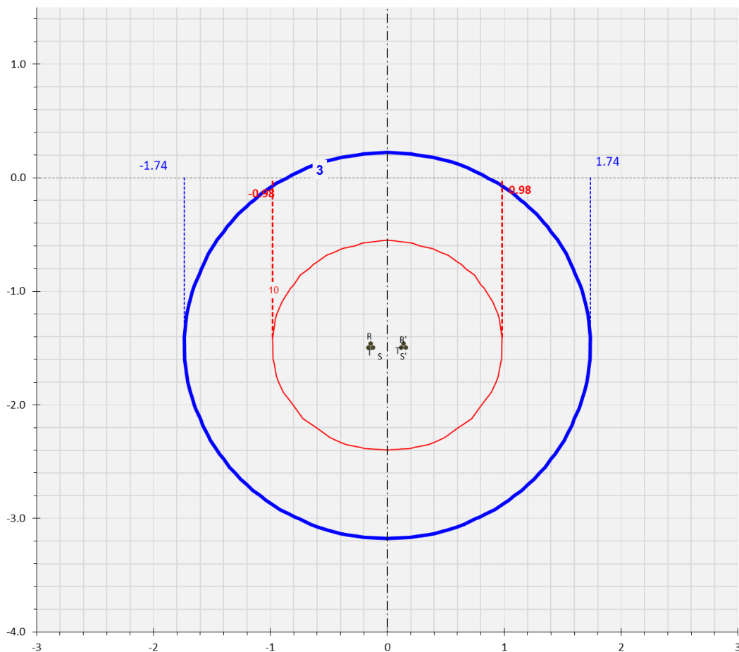
Figura 7: Curve di equilivello per il campo di induzione magnetica generato dalla linea (Sezione 2 – due terne a 36 kV)
