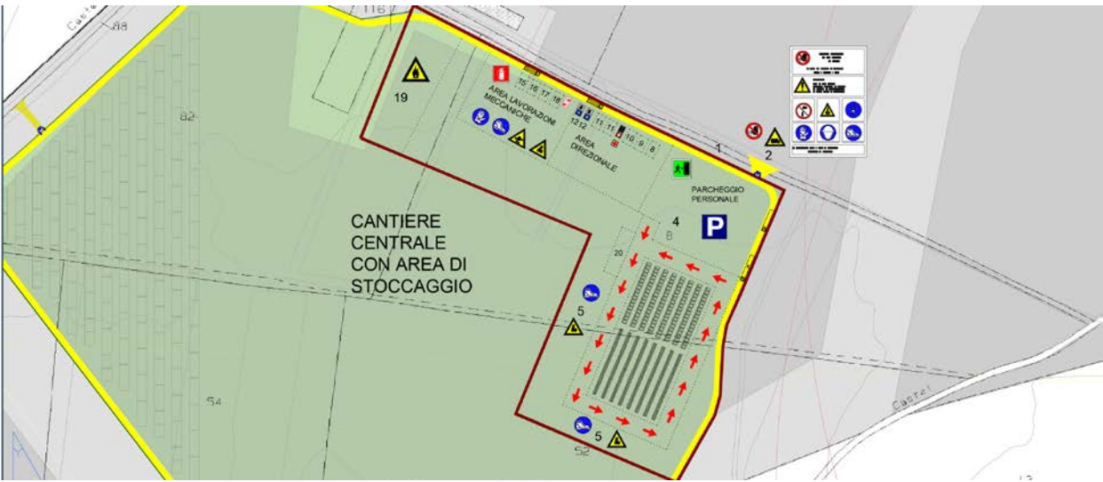
Fig.1 – Fase di ricezione, stoccaggio e movimentazione materiali, dettaglio apprestamenti
