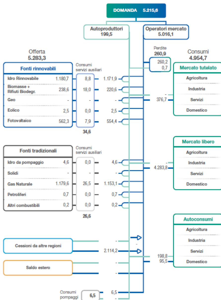
Figura 29 - flussi di energia elettrica, Umbria
