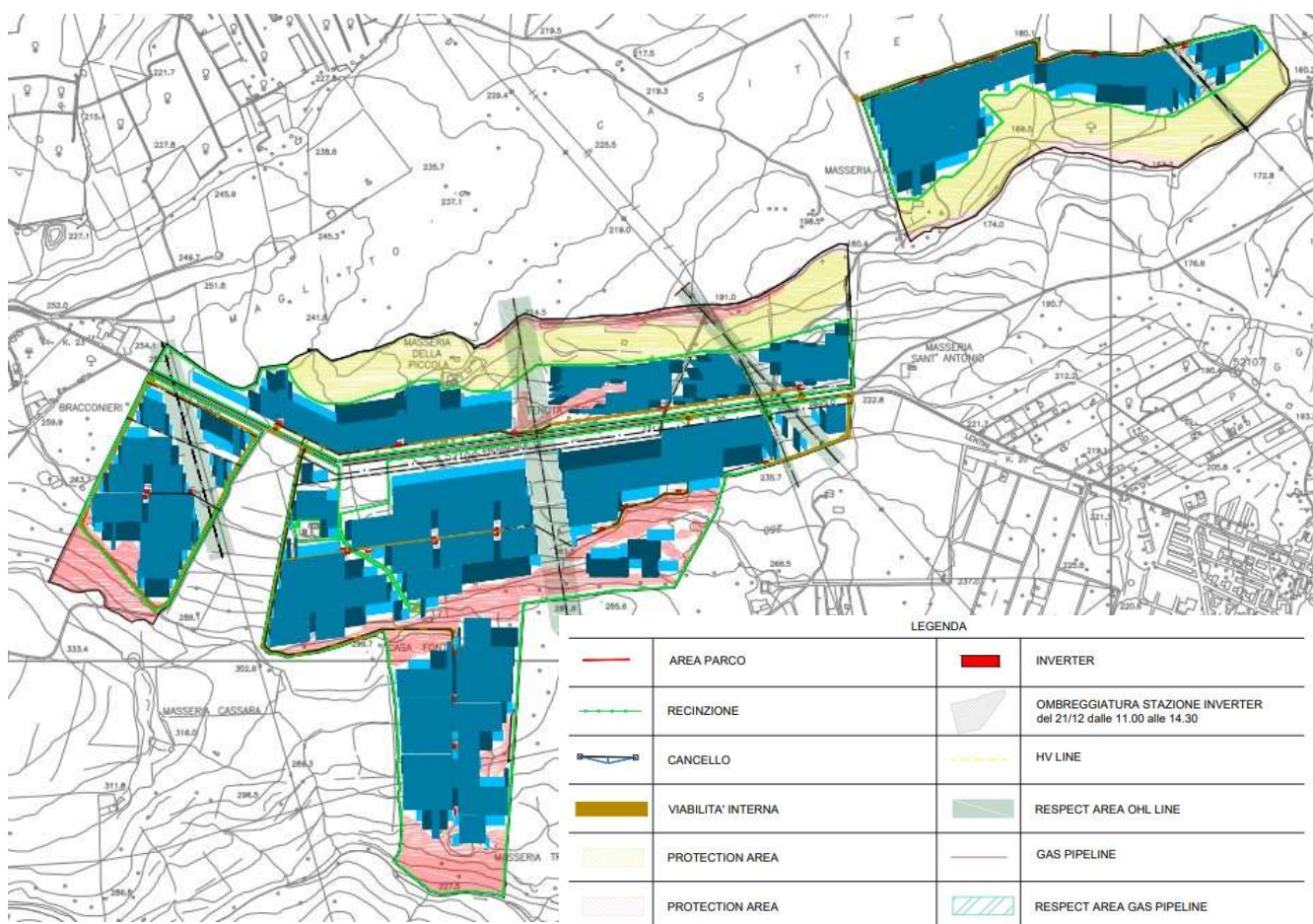
Figura - Layout di impianto
