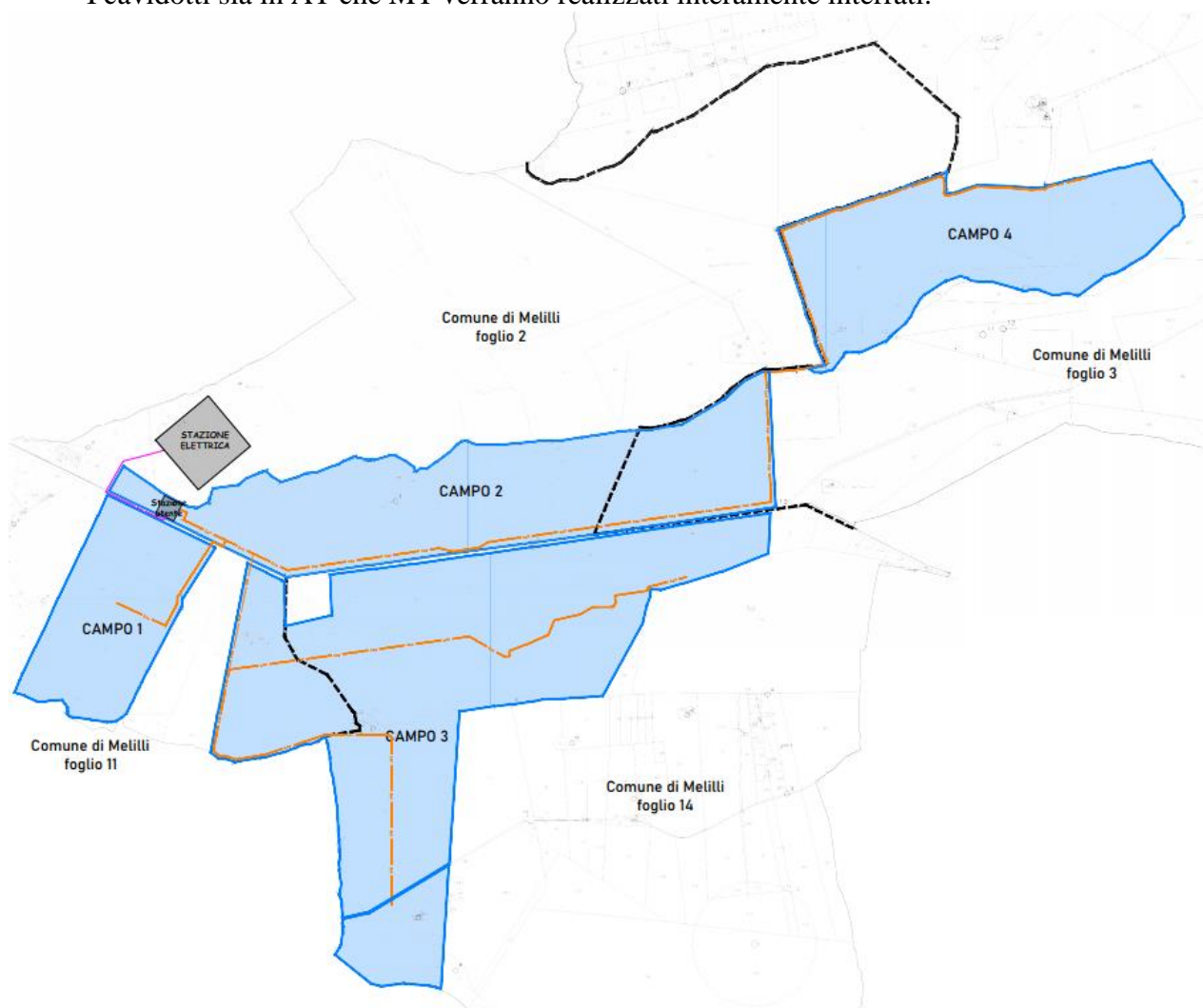
Figura 1 – Percorso cavidotto in MT (arancione) e in AT (magenta)
