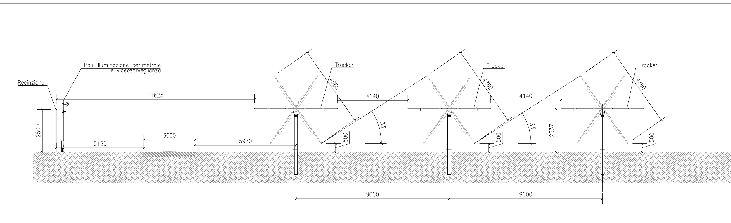
SEZIONE STRADA B1-B1 scala 1:100
