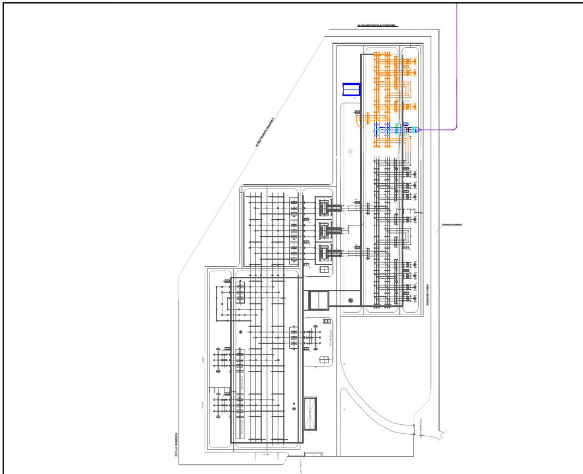
Fig. 5 - Planimetria elettromeccanica dello Stallo di Arrivo nella SE-RTN.
