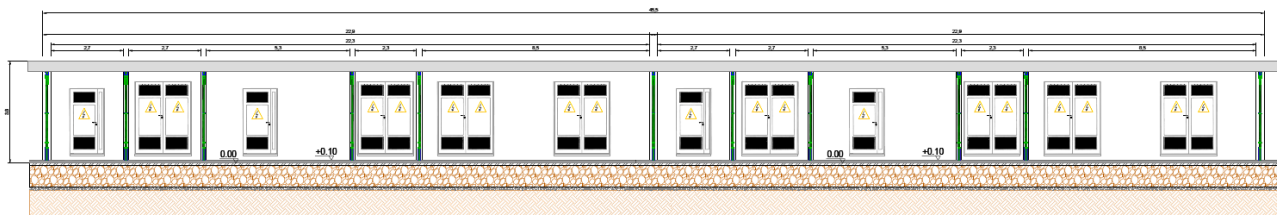
Fig. 11 - Prospetto principale dei locali tecnici della SSE.
