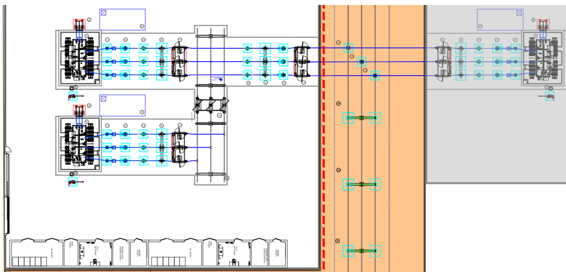
Fig. 7 - Planimetria elettromeccanica della SSE, con stralcio dello stallo di connessione dell'impianto in esame.
