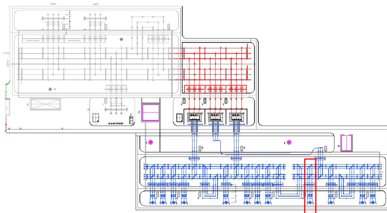
Fig. 12 - Posizione dello Stallo di connessione alla RTN, riquadrato in rosso, così come indicato da TERNA
