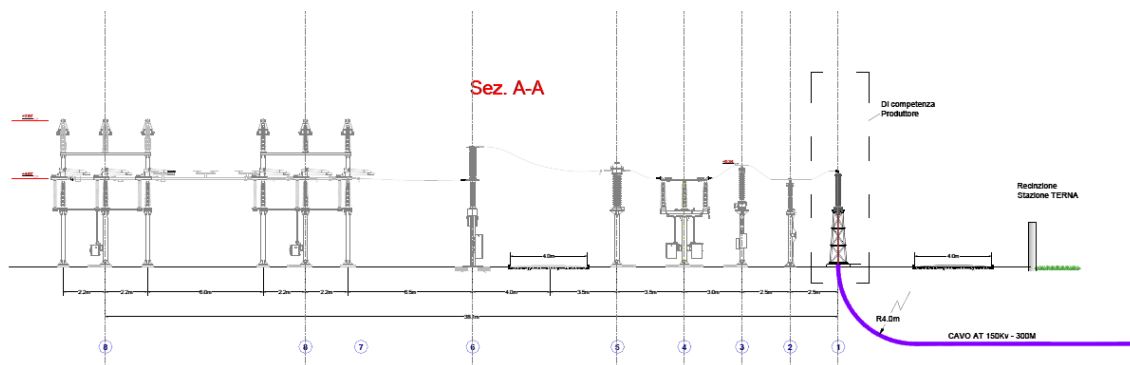
Fig. 15 - Sezione elettromeccanica con i nuovi componenti per lo stallo in area SE-RTN.
