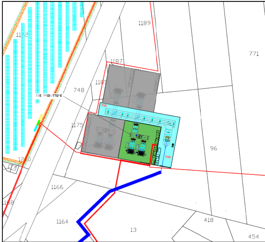
Fig. 1a - Planimetria Sottostazione elettrica condivisa su CTR: in verde lo stallo assegnato all'impianto in esame; in grigio, gli stalli assegnati alle società produttori condividenti; in ciano, il sistema di sbarre comuni a 150 kV; in blu, l'elettrodotto interrato AT per la connessione in SE-RTN; in rosso, i cavidotti in MT per le connessioni interne dell'impianto in esame.
