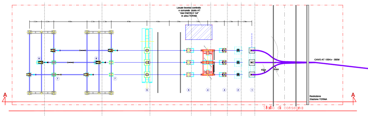
Fig. 14 - Stralcio elettromeccanico con i nuovi componenti per lo stallo in area SE-RTN.
