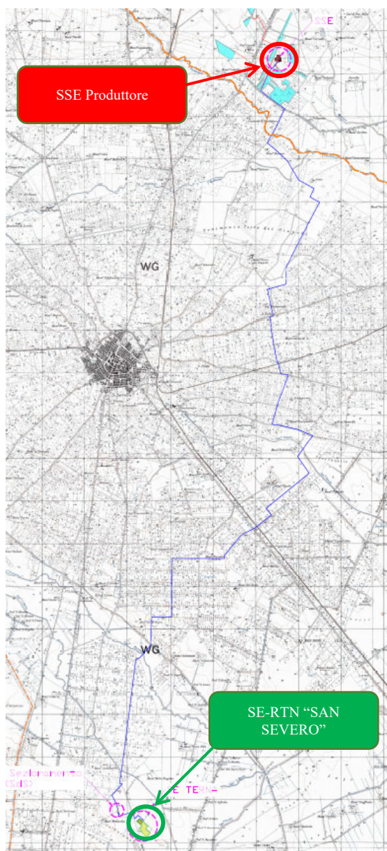
Fig. 2 - Stralcio di dettaglio su IGM con l'ingombro delle opere: cerchiata in verde la Stazione Elettrica TERNA, in rosso la SSE Produttore condivisa; in blu l'elettrodotto AT di connessione alla Stazione Elettrica TERNA; in ciano parte dell'impianto della società AM ENERGY 2Srl.
