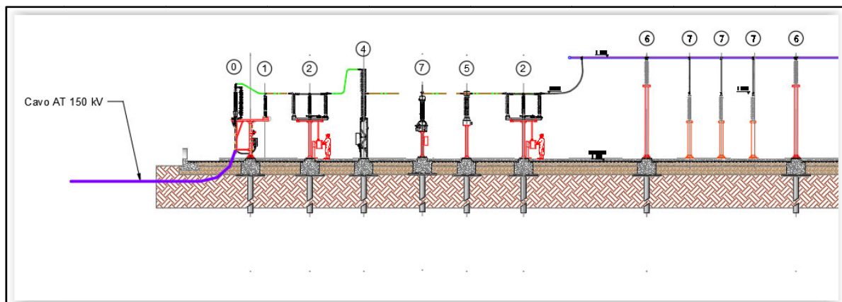
Fig. 6 - Sezione elettromeccanica dello Stallo di Arrivo SE-RTN.
