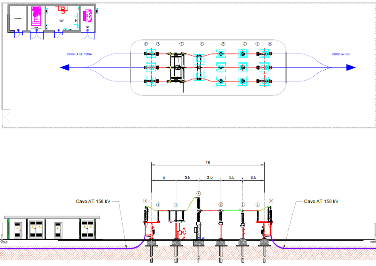
Fig. 9 - Sezione elettromeccanica della Stazione di Sezionamento (SdS)
