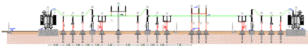
Fig. 8 - Sezione elettromeccanica del montante di trasformazione MT/AT
