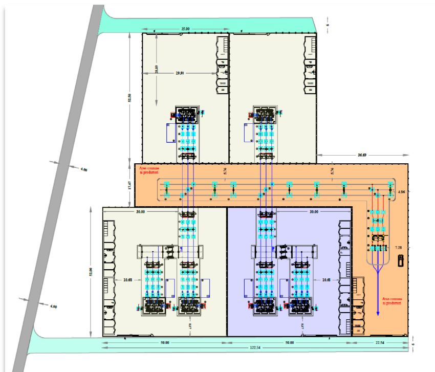
Fig. 4 - Elaborato grafico Sottostazione Produttori per la condivisione: in ciano, la viabilità di accesso; in arancione, l'area comune per la condivisione dello Stallo; in giallo, le sottostazioni di altri produttori; in viola, lo stallo dell'impianto oggetto della presente relazione
