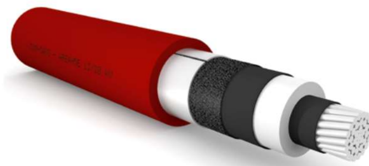
Figura 5 - Particolare degli strati costitutivi di un cavo MT ARE4H5E.
