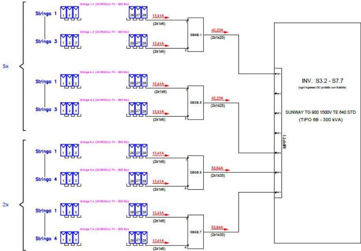
Figura 6- Schema elettrico tipico del collegamento tra quadri di stringa ed inverter Tipo 4-5-6 (7 input DC) centralizzato
