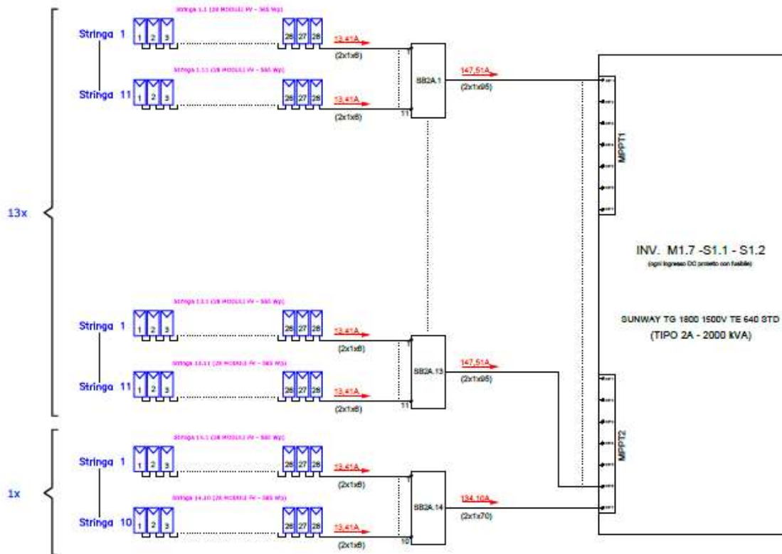
Figura 5 - Schema elettrico tipico del collegamento tra quadri di stringa ed inverter Tipo 2-3 (14 input DC) centralizzato.
