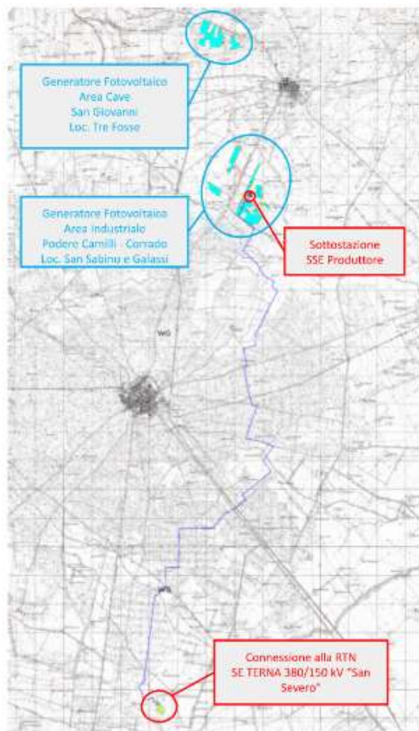
Figura 1 -Inquadramento di ampio raggio su IGM dell'area di intervento. A Nord, in celeste, la centrale agri-fotovoltaica; in blu il percorso dell'elettrodotto AT dorsale, che si sviluppa per circa 24,6 km prevalentemente lungo rete viaria esistente; in località San Sabino la Sottostazione SSE Produttore, a Sud la Stazione elettrica di Trasformazione SE-TERNA 380/150kV.
