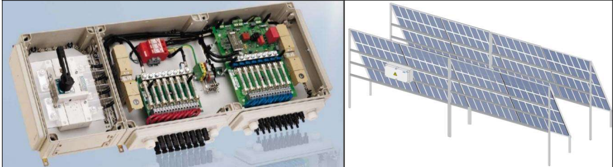
Figura 3 - Particolari Sunny String Monitor.
