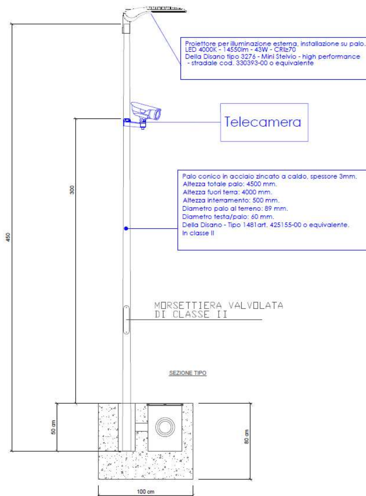
Figura 7 - Installazione telecamera su palo di illuminazione.
