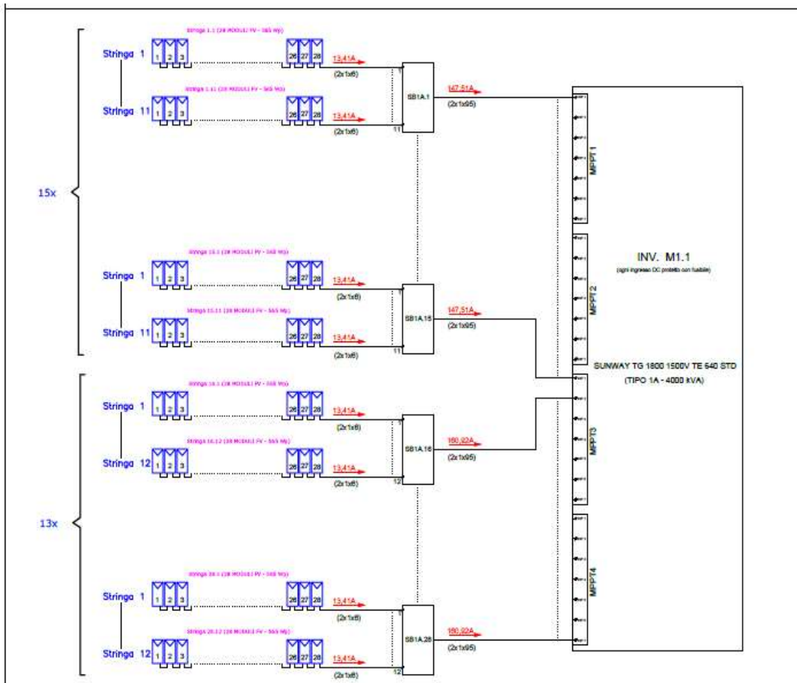
Figura 4 - Schema elettrico tipico del collegamento tra quadri di stringa ed inverter Tipo 1 (28 input DC) centralizzato.
