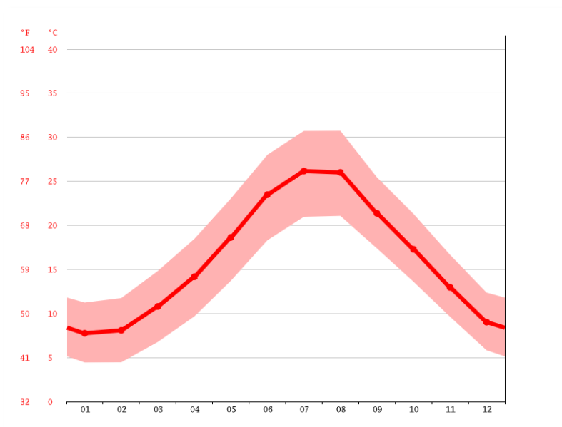
Fig. 2.3 – Temperature medie annue del Tavoliere - Data: 1991 - 2021
