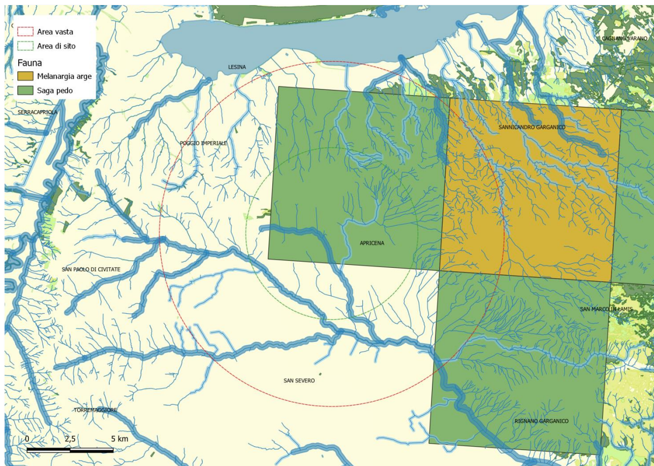
Fig. 2.8 – Quadranti in cui sono state segnalate Saga pedo e Melanargia arge .
