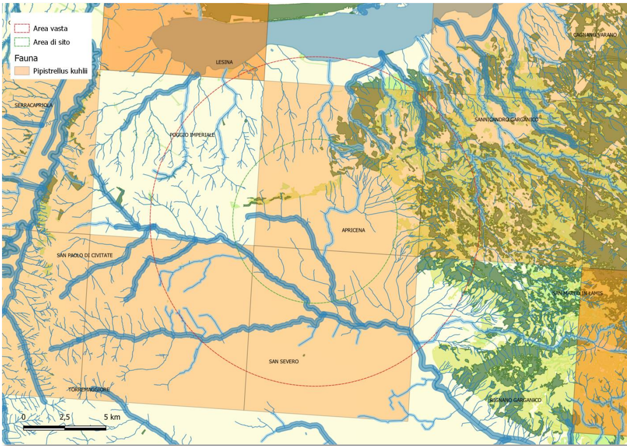
Fig. 2. 12 – Quadranti in cui è stata segnalata Pipistrellus kuhlii .
