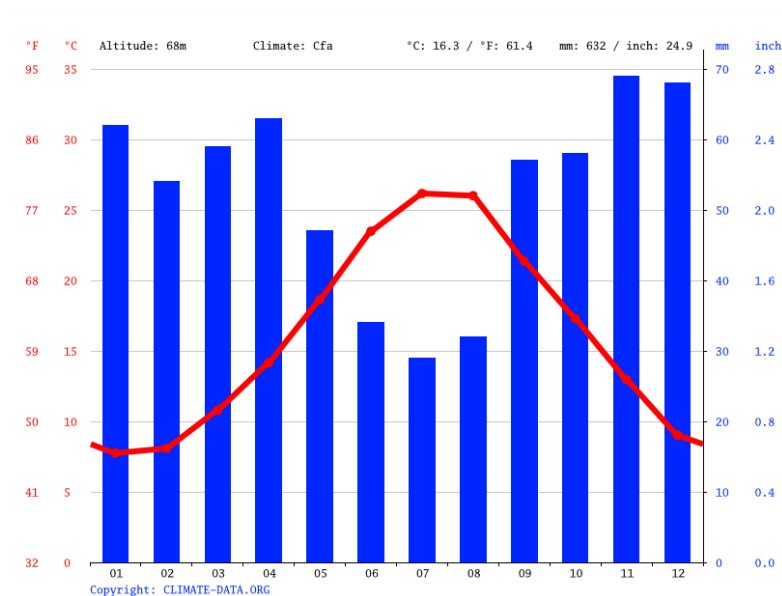
Fig. 2.2 – Climogramma del Tavoliere - Data: 1991 - 2021
