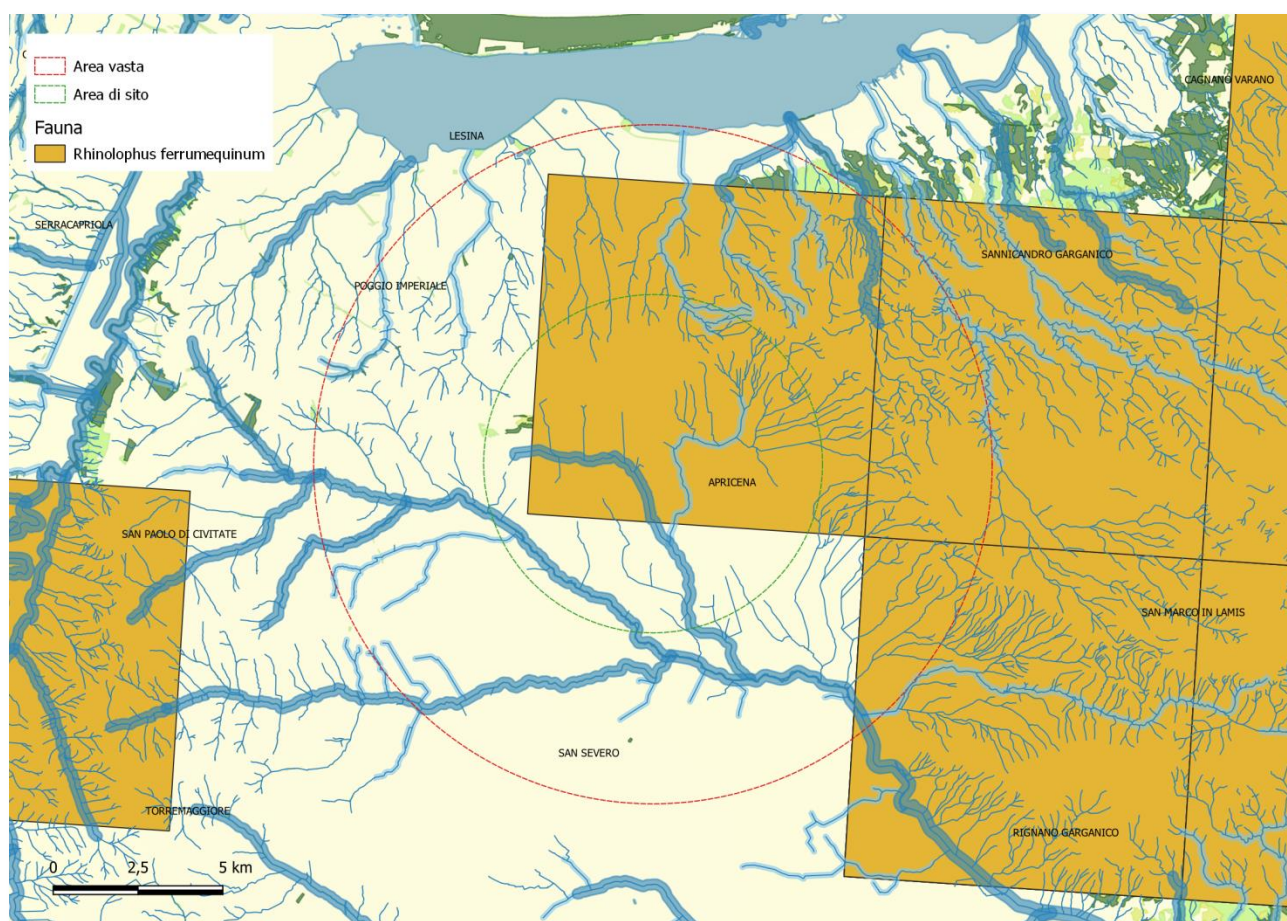
Fig. 2. 11 – Quadranti in cui è stata segnalata Rhinolophus ferrumequinum .
