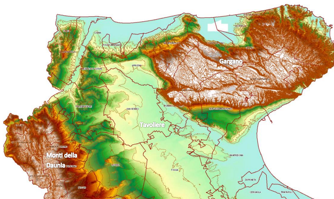
Fig. 2.1 – Macro distretti geomorfologici
