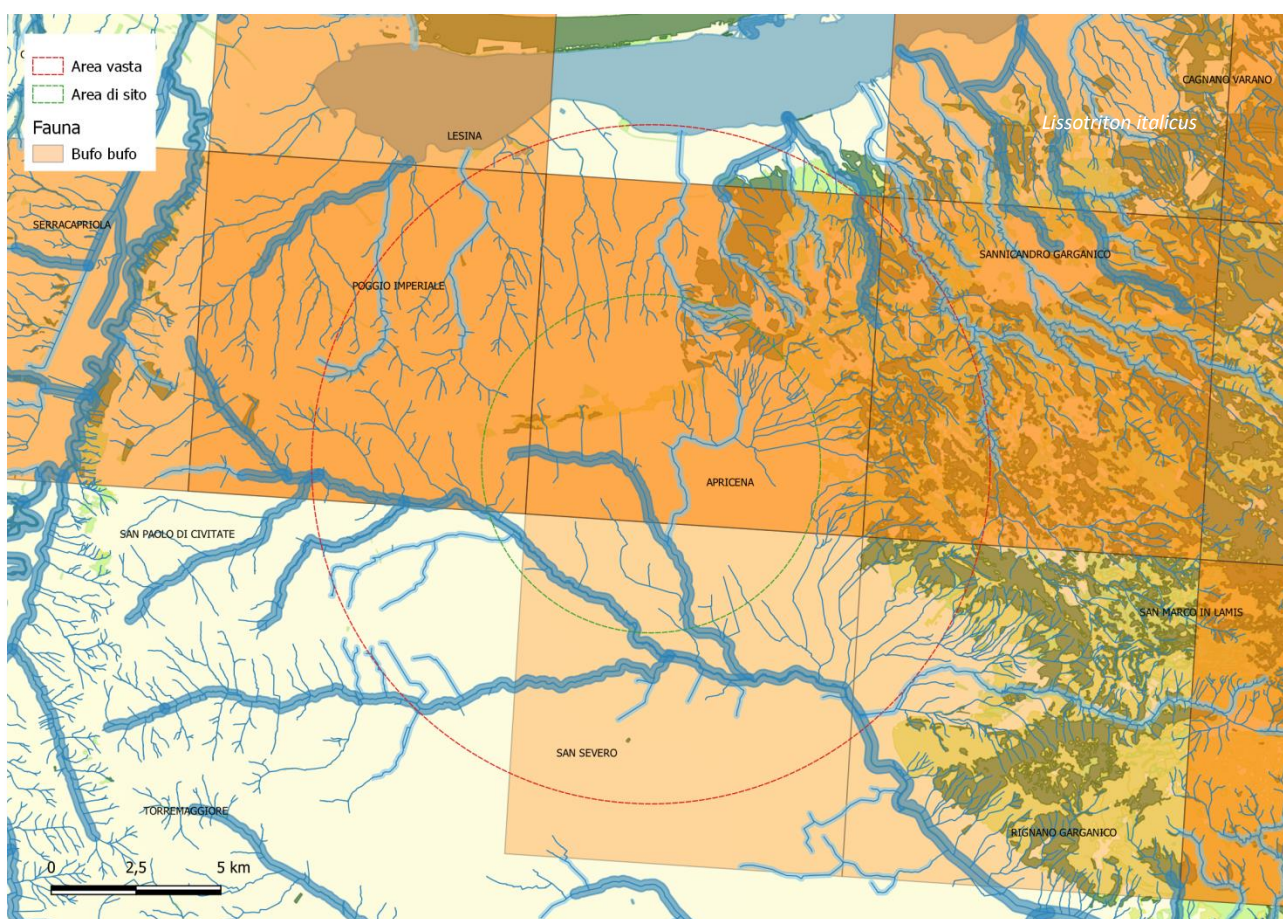
Fig. 2.9 – Quadranti in cui è stata segnalata Bufo bufo .
