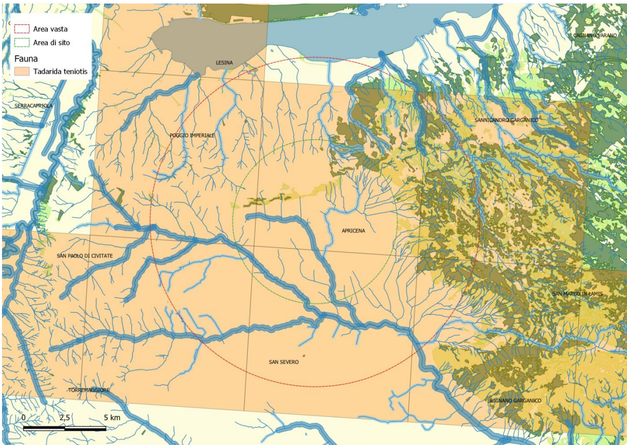
Fig. 2. 13 – Quadranti in cui è stata segnalata Tadarida teniotis .
