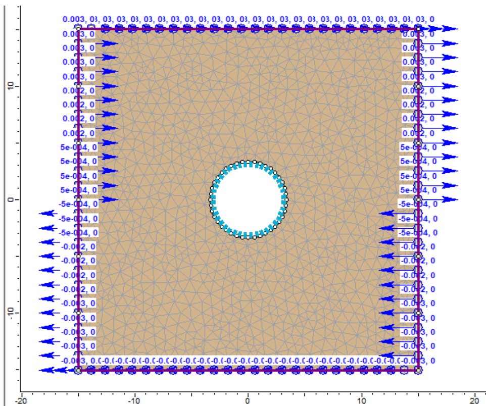
Figura 4.2 – Modello relativo alla galleria idraulica per le condizioni sismiche all'ultimo step di analisi
