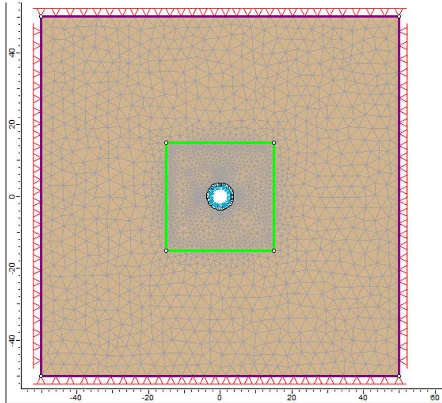
Figura 4.1 – Modello relativo alla galleria idraulica per le condizioni statiche all'ultimo step di analisi
