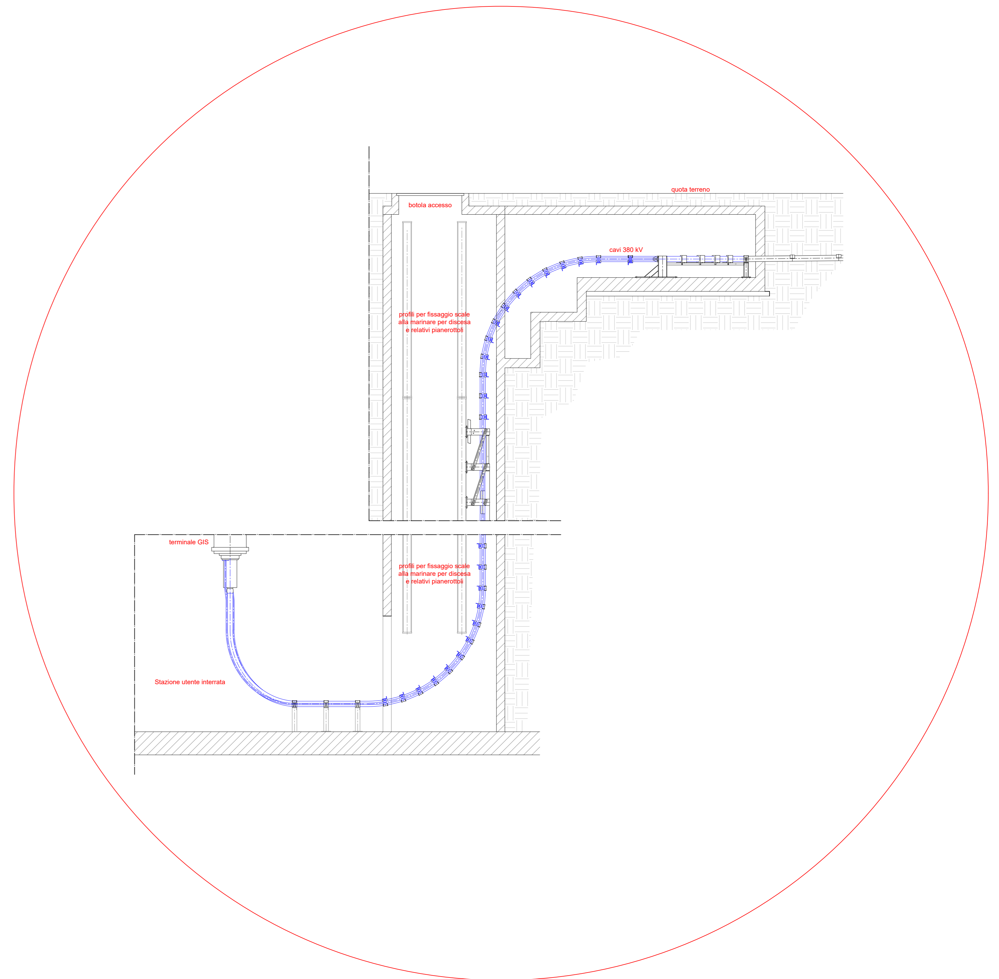
Tipologico galleria discesa cavi Scala 1:50
