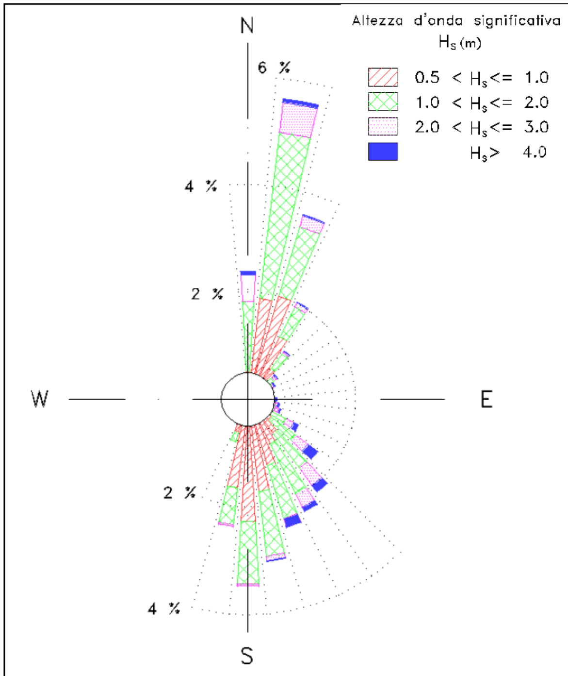
Figura 4 - Rosa della distribuzione direzionale degli eventi di moto ondoso annuali alla boa ondometrica di Crotona.
