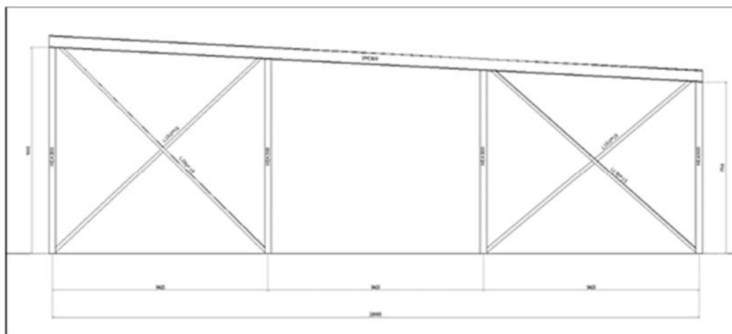
Figura 45 - Prospetto struttura pensilina di copertura della baia di carico
