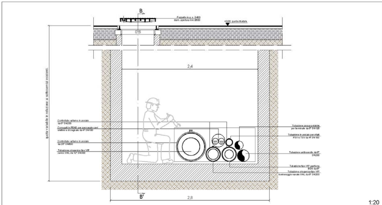
Figura 14 – Sezione trasversale sul pozzetto di ispezione
