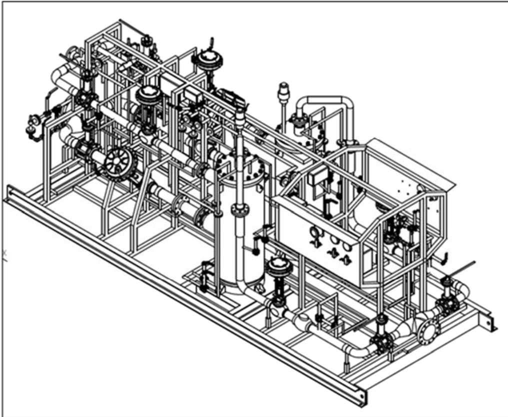
Figura 22 - “Skid” tipologico con doppia pompa per GNL
