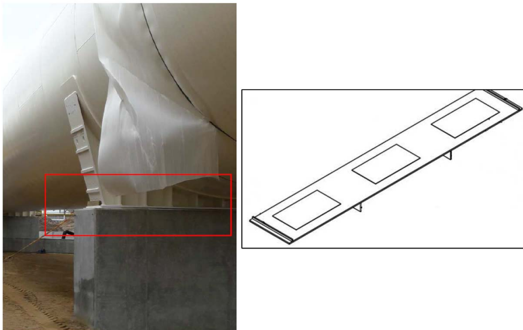
Figura 19 – Esempio piastra di scorrimento per dilatazione
