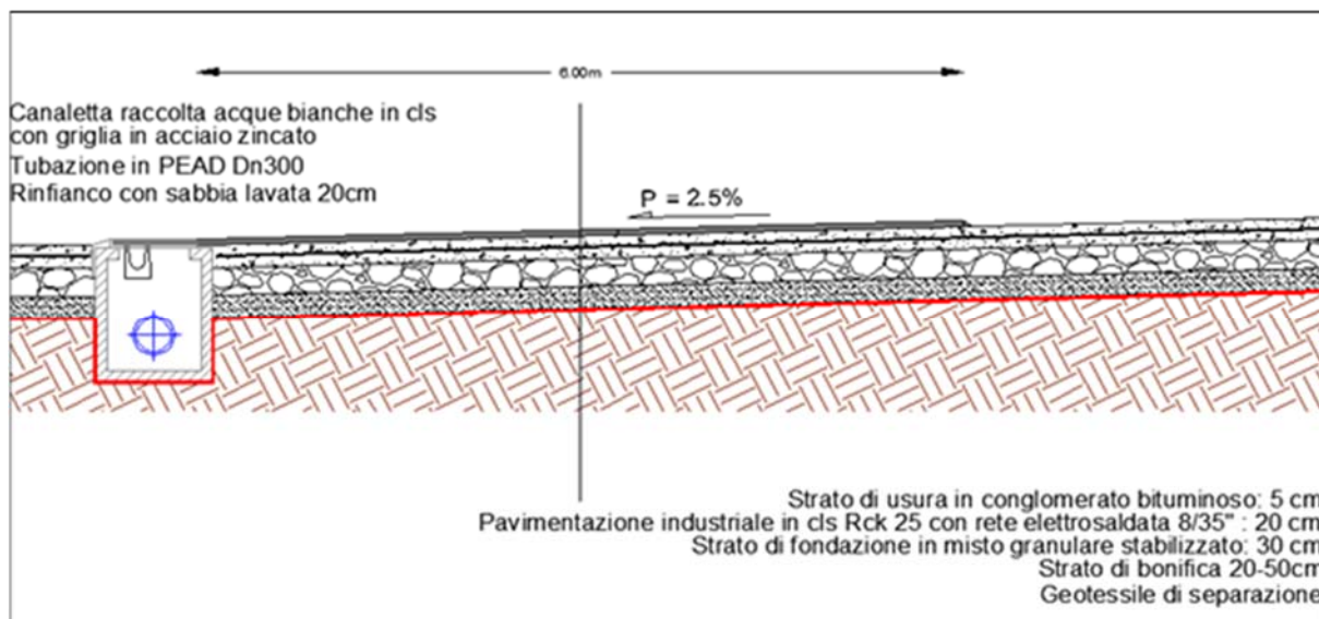
Figura 37 - Pacchetto Stradale
