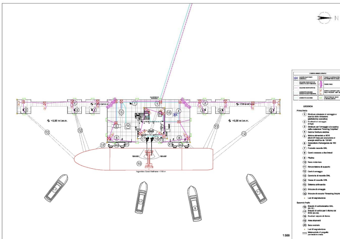
Figura 40 - Impianto elettrico e di illuminazione area Terminale
