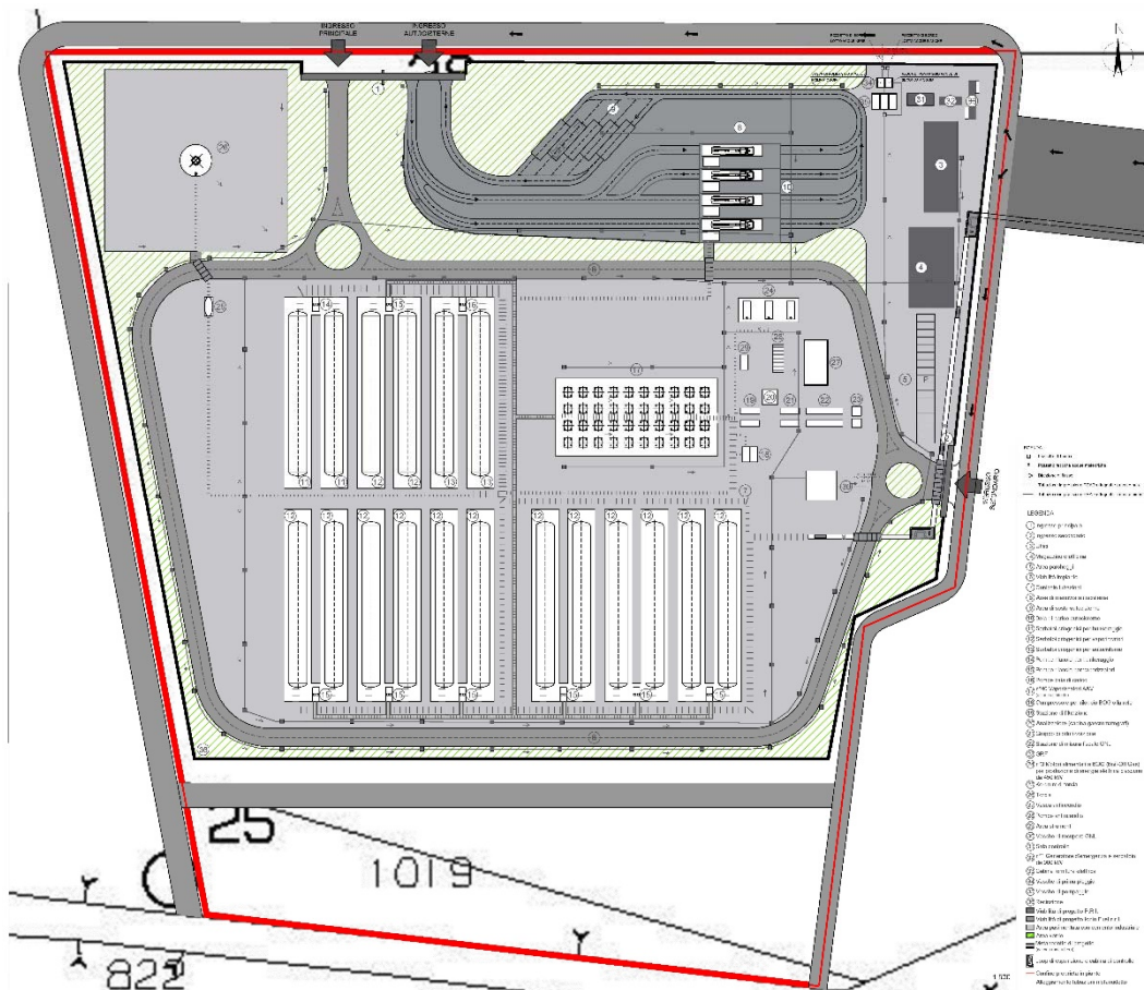
Figura 46 - Planimetria rete di raccolta acque meteoriche
