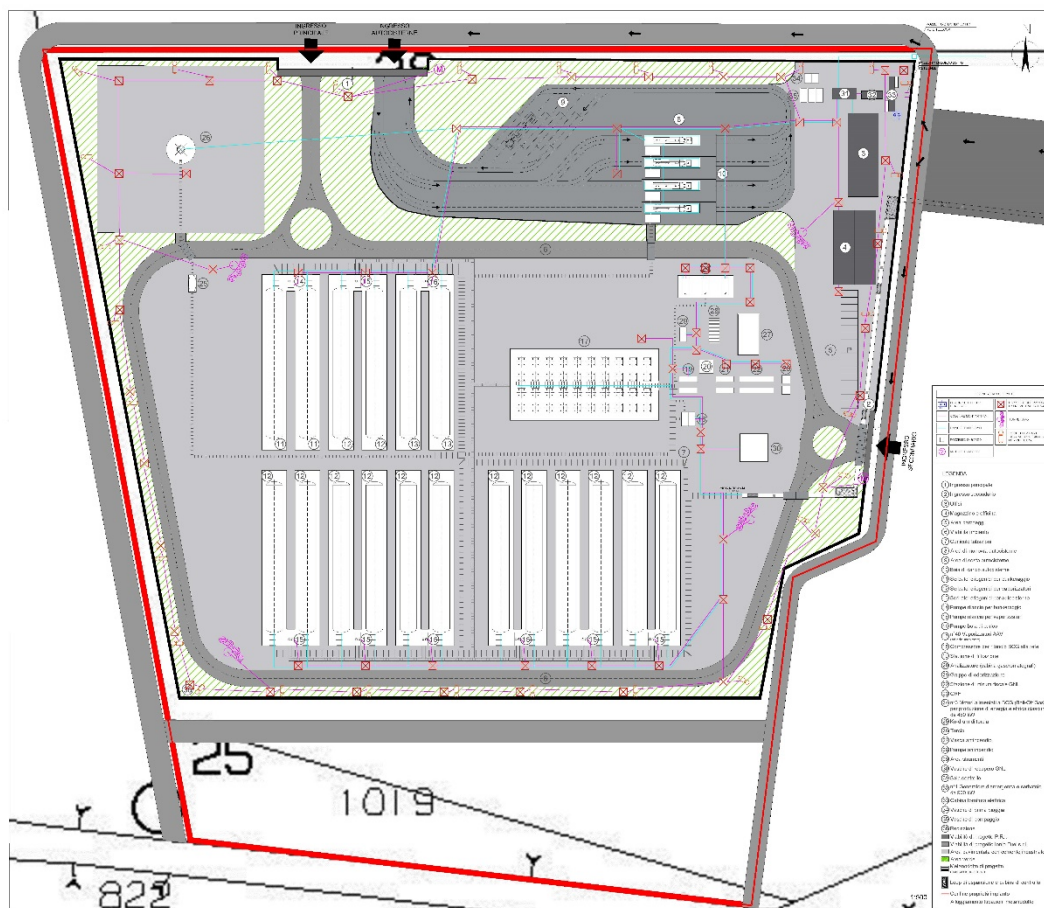
Figura 39 - Impianto elettrico e di illuminazione area deposito
