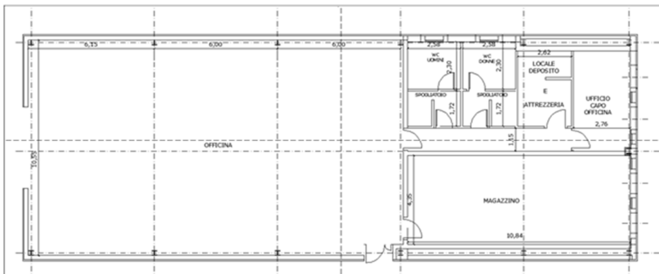
Figura 44 - Pianta edificio magazzino e officina
