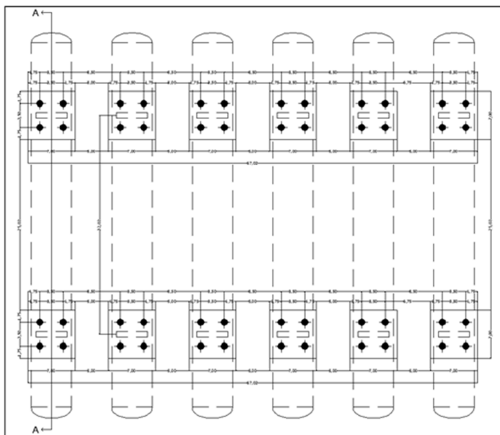
Figura 36 - Pianta fondazioni serbatoi
