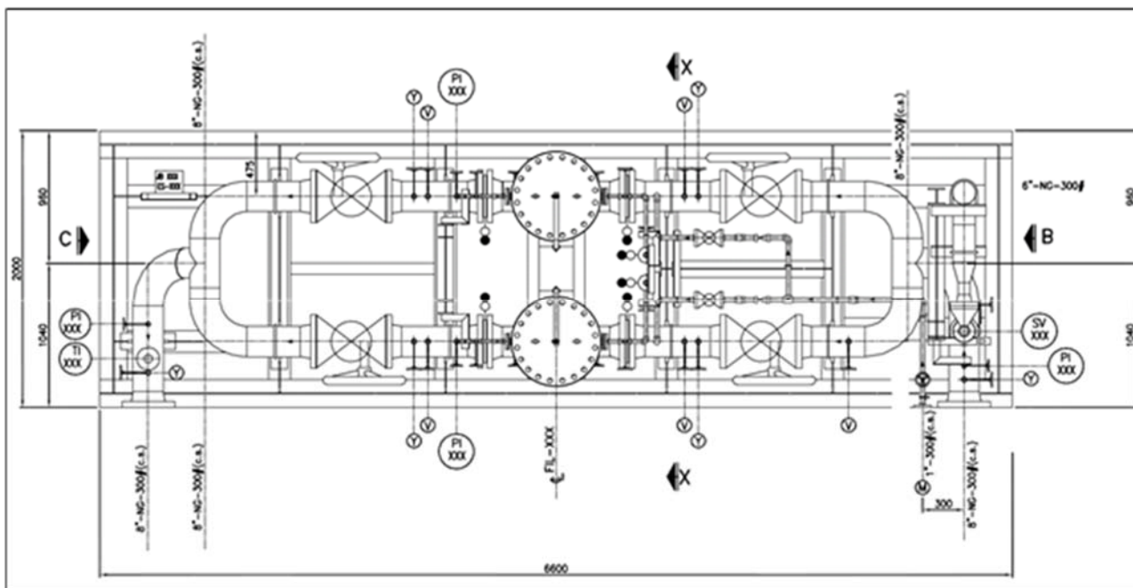
Figura 29 - Skid Sistema di filtrazione
