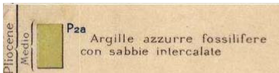
Figura 2 - Stralcio della Carta Geologica d'Italia "Crotona" F.228
