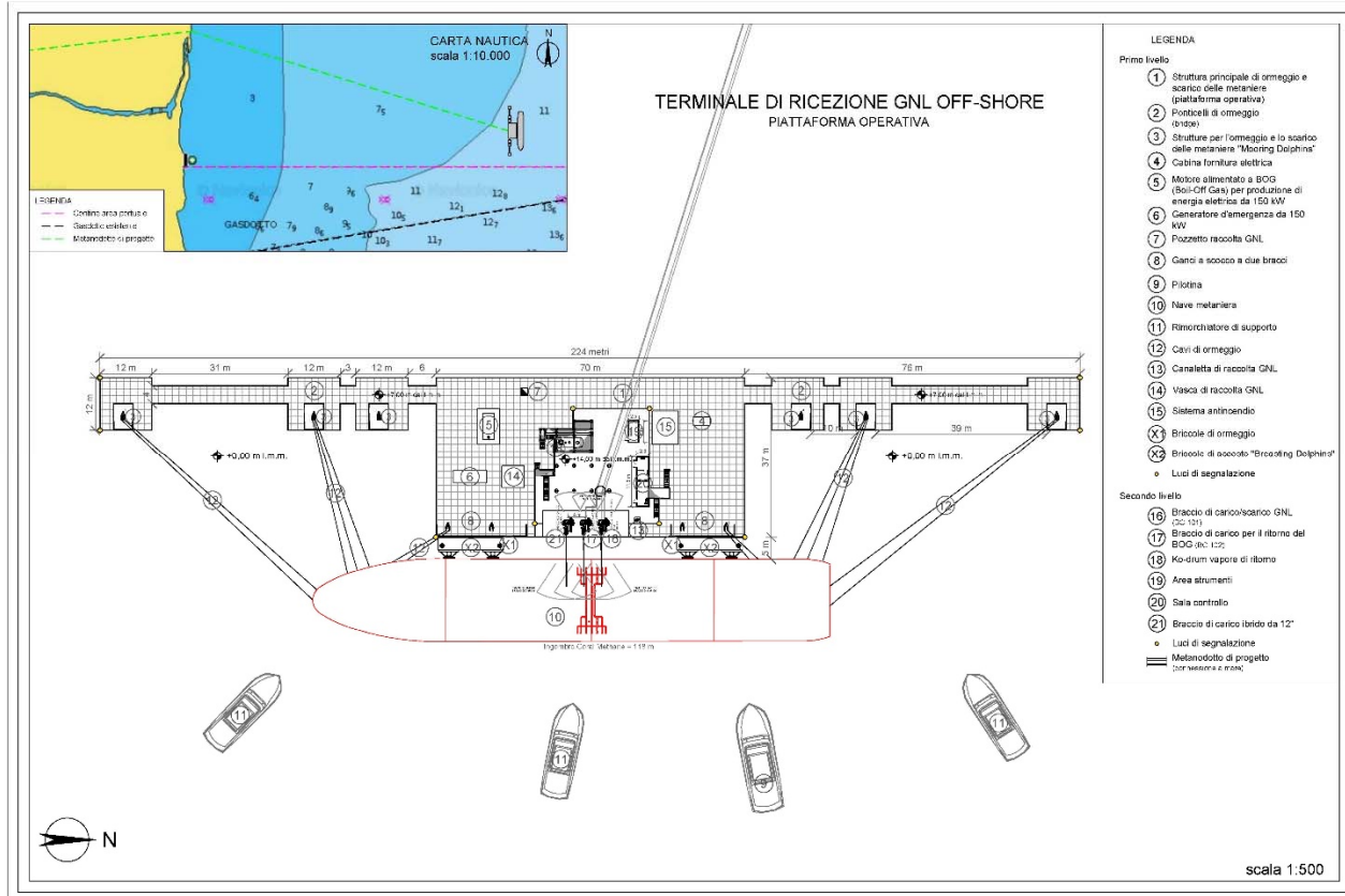
Figura 6 – Planimetria generale del Terminale Off-Shore
