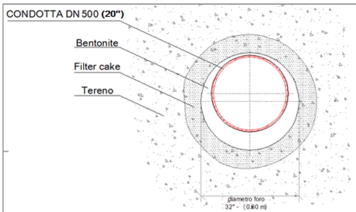
Figura 35 -sezione tipo con Filter cake
