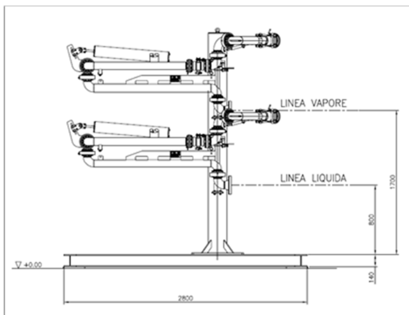
Figura 26 - Bracci di carico per autocisterne criogeniche
