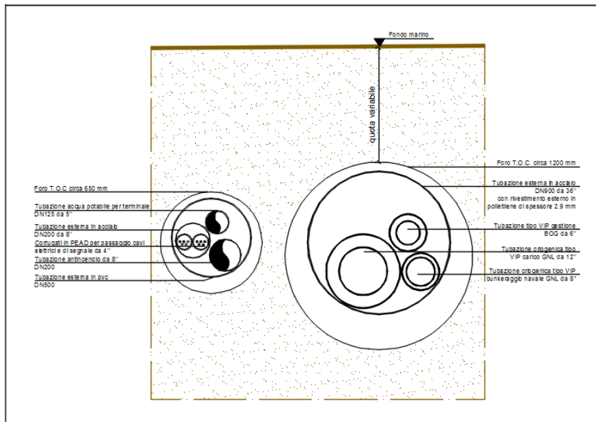
Figura 15 – Sezione trincea gasdotto condotta a mare
