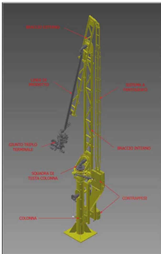
Figura 9 - Esempio braccio di carico marino con tubazioni inox – Assieme generale
