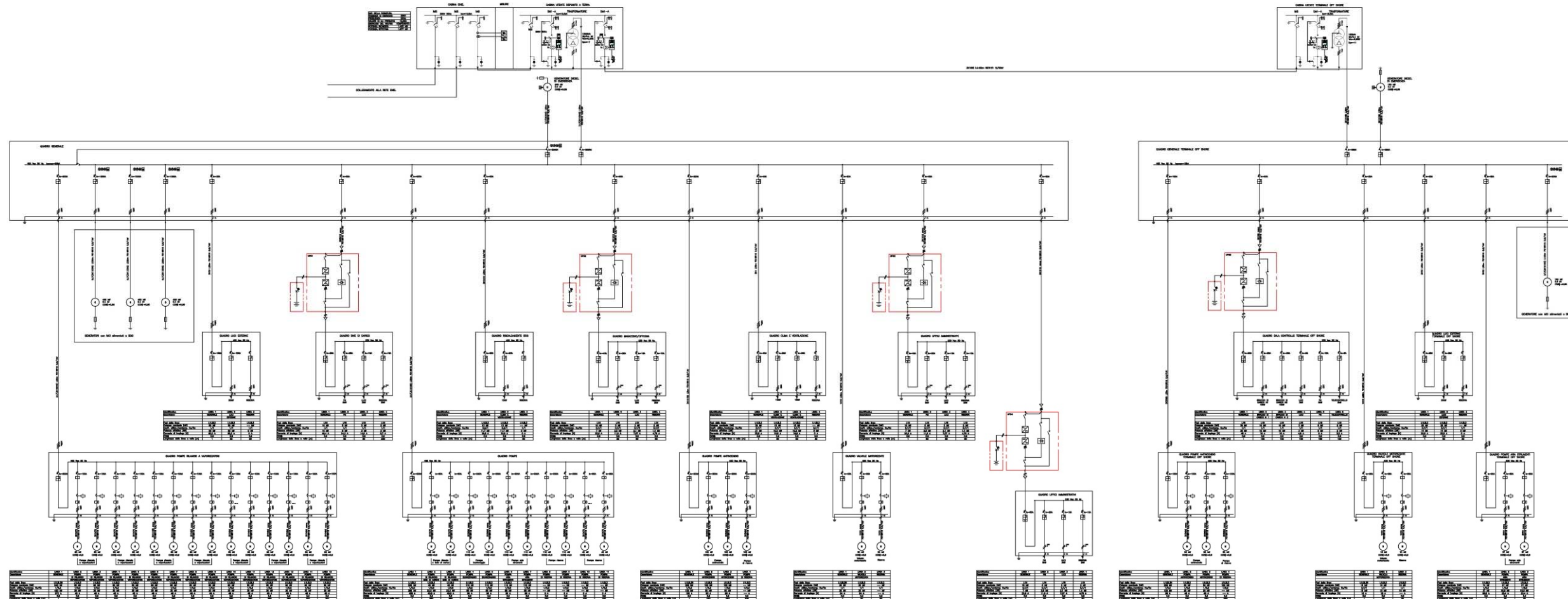
Figura 8 - Schema elettrico del Deposito costiero e del Terminale Off-Shore
