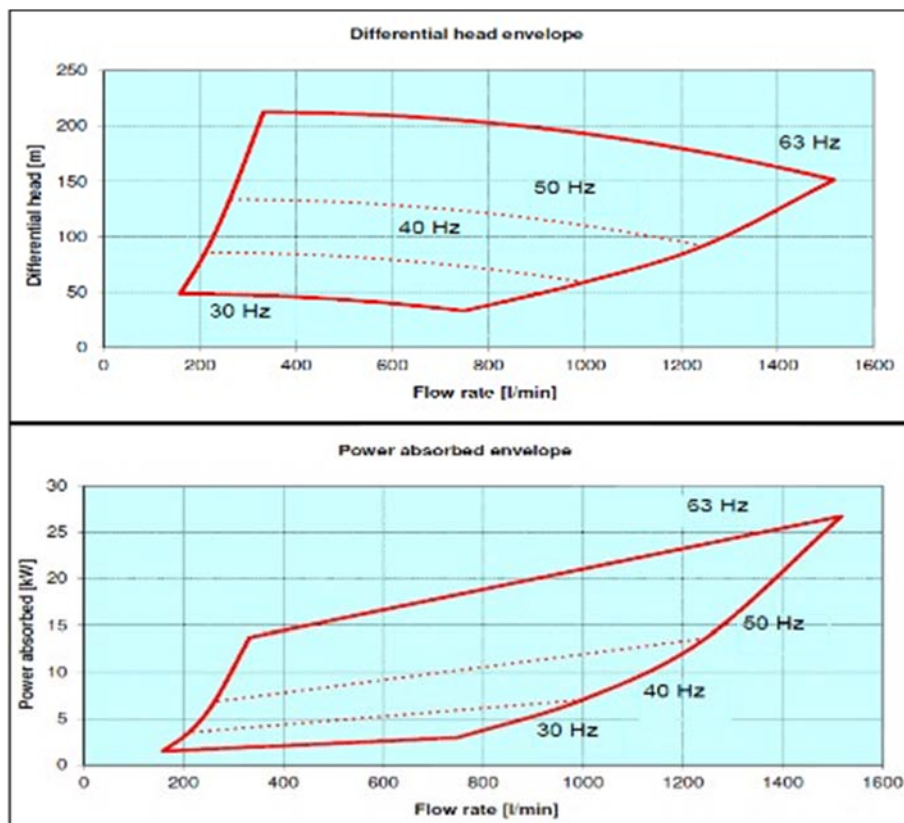
Figura 23 - Curva caratteristica delle pompe criogeniche per le baie di carico
