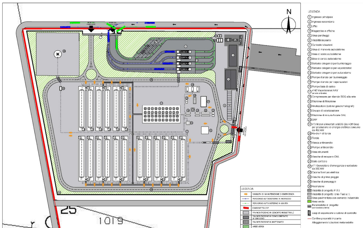
Figura 38 - P_05_UR_01_VIA_R00 Planimetria viabilità impianto
