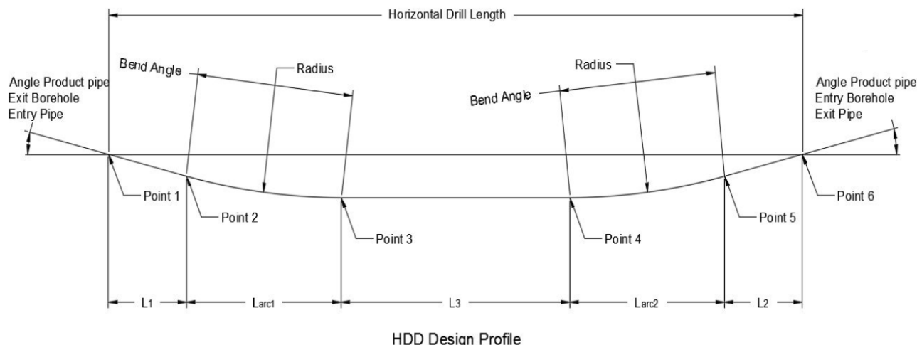
Figura 34 – Asse di perforazione
