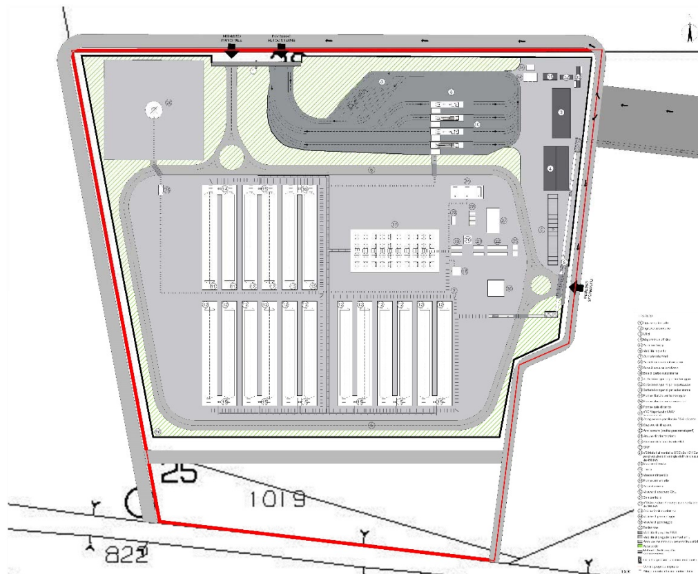
Figura 5 – Planimetria generale del Deposito
