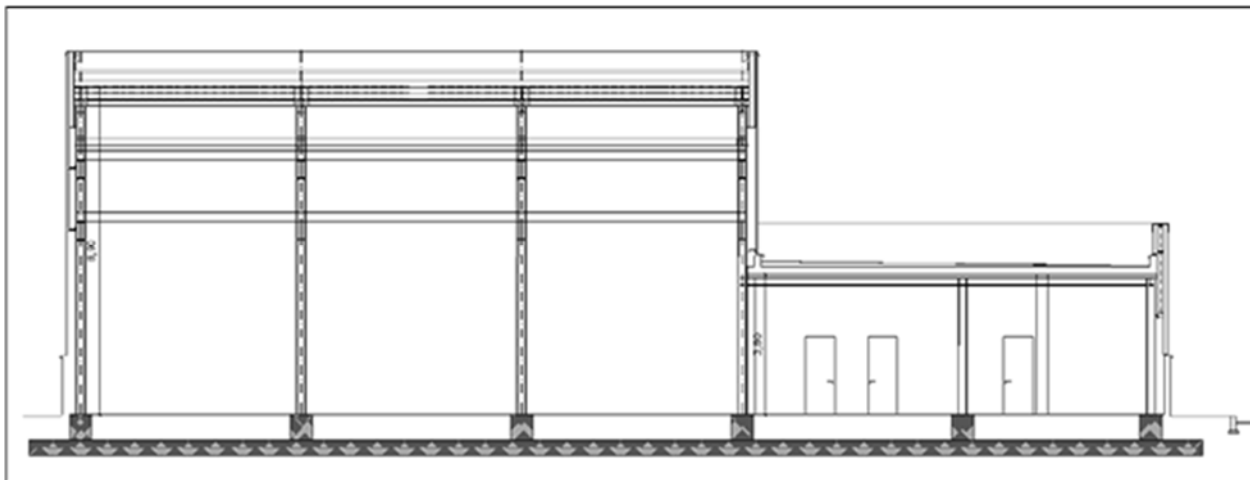
Figura 43 - Sezioni edificio officina e magazzino
