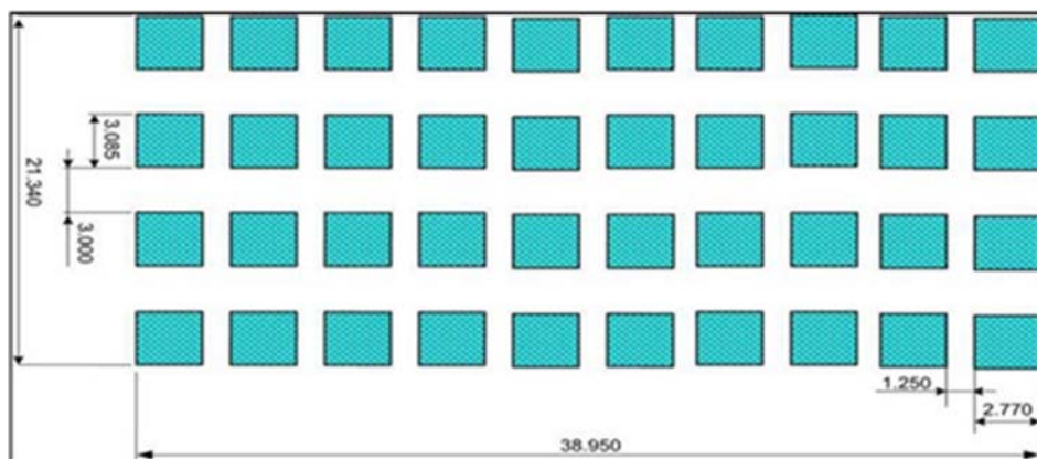
Figura 24 - Disposizione planimetrica dei Vaporizzatori
