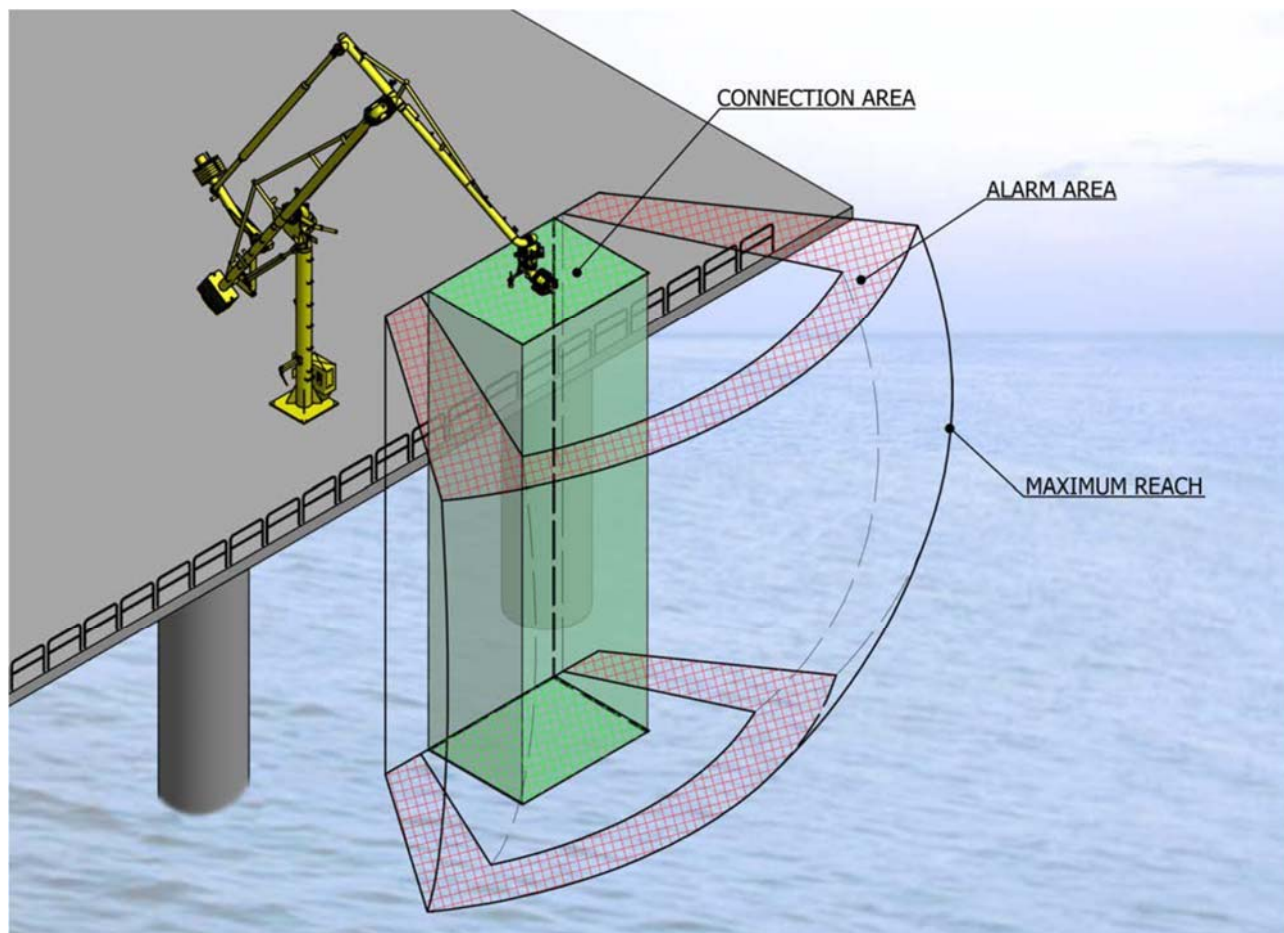
Figura 10 - Schema illustrativo campo di lavoro
