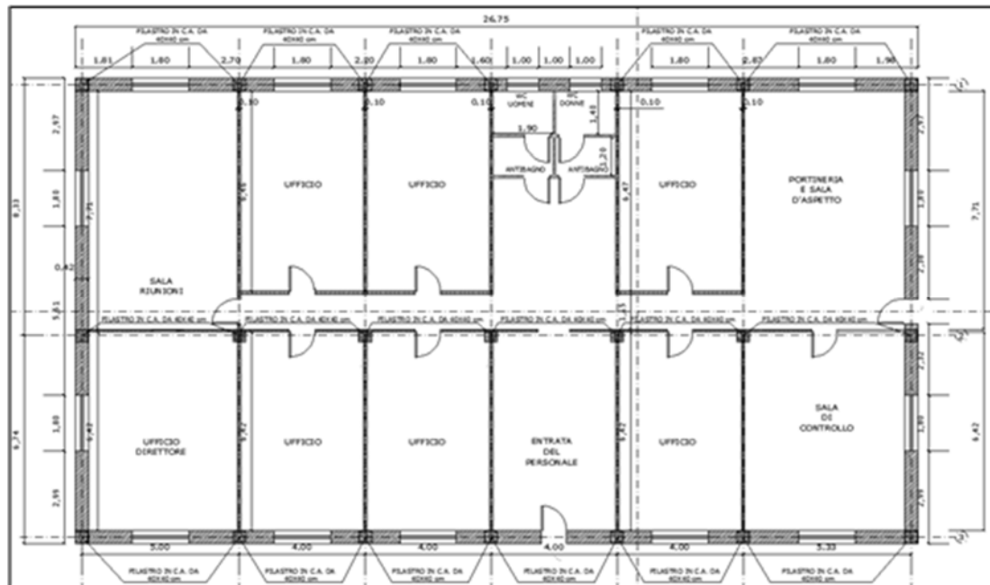
Figura 42 - Edificio amministrazione Pianta
