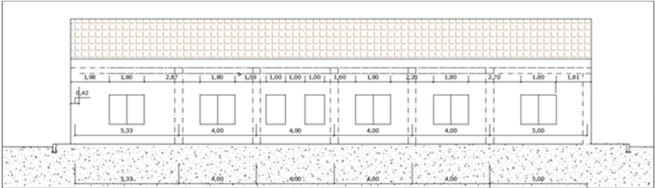
Figura 41 - Prospetto Ovest edificio amministrazione
