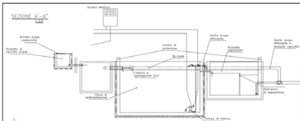
Figura 47 - Sezione dell'impianto di trattamento previsto
