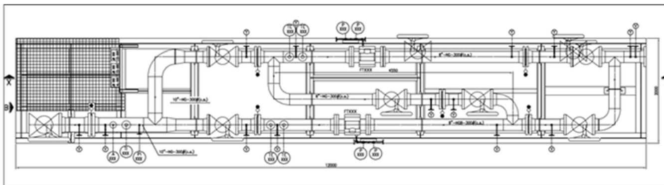
Figura 32 - Skid stazione di misura fiscale
