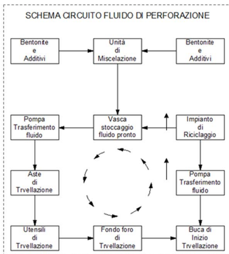
Schema circuito fango bentonitico
