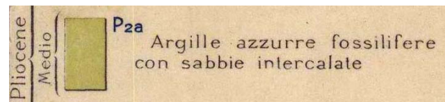
Figura 2 - Stralcio della Carta Geologica d'Italia "Crotona" F.228
