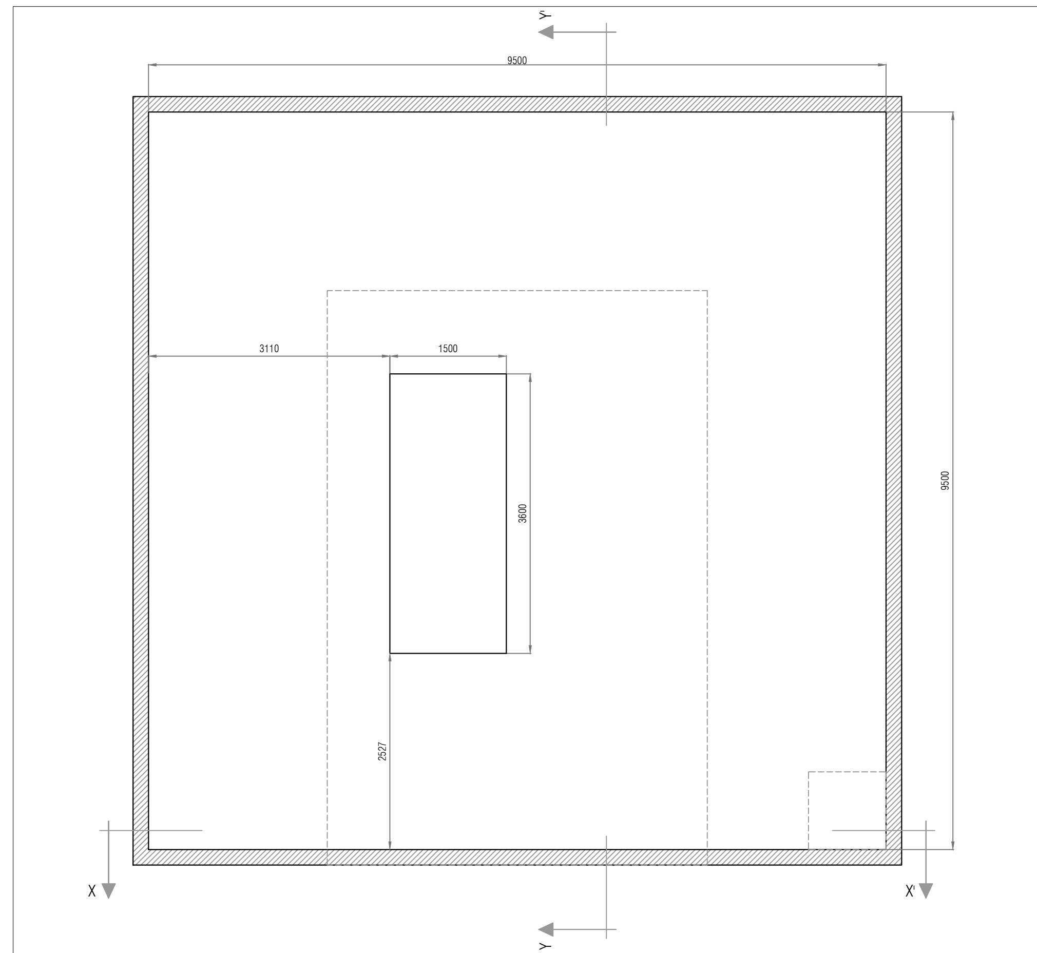
PLANIMETRIA
