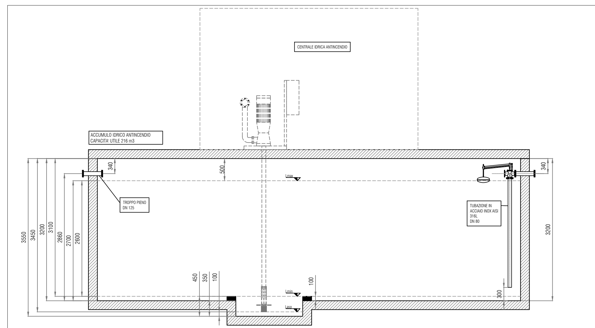
SEZIONE X-X
