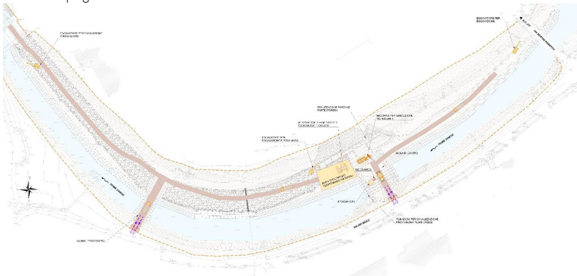
Figura 3 - Estratto planimetrico del cantiere della nuova traversa (PE-000-CAN-GE-005-PL): Macrofase 1
