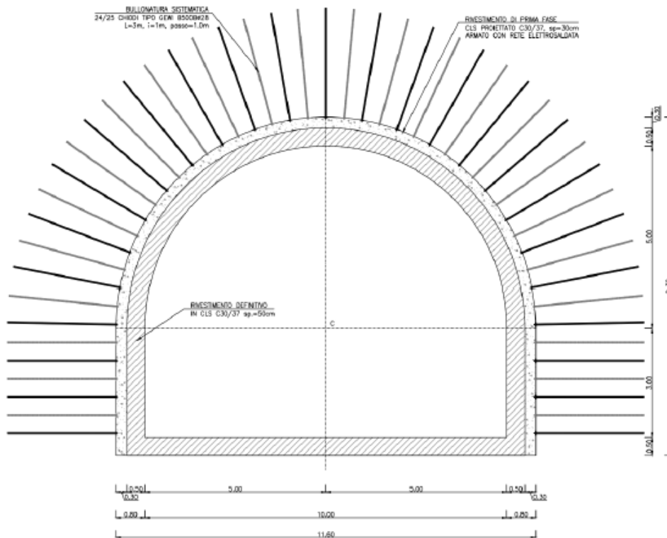
Figura 3.1: Sezione tipo della discenderia
