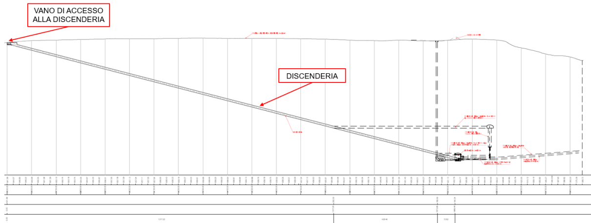
Figura 6.1: Profilo longitudinale della discenderia (Profilo longitudinale 1351-A-FN-D-06-1)
