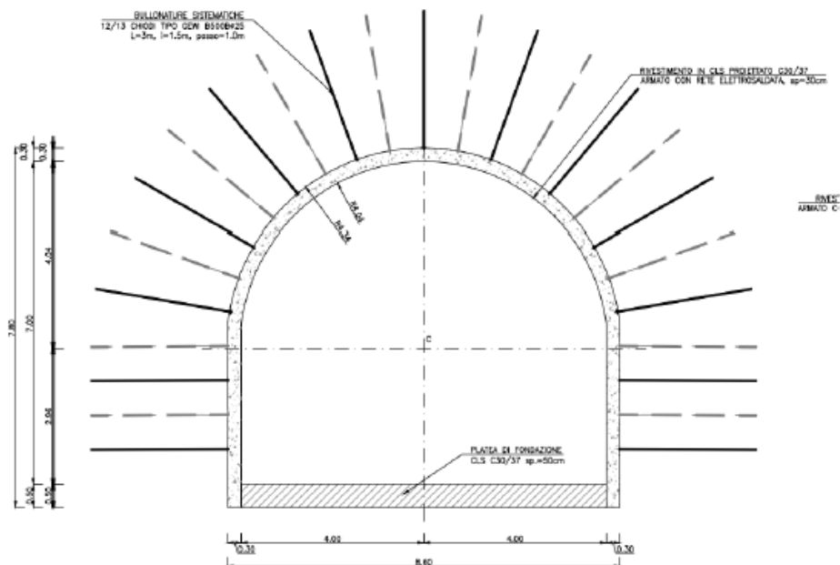
Figura 3.3: Sezione tipo della galleria d'accesso al pozzo piezometrico
