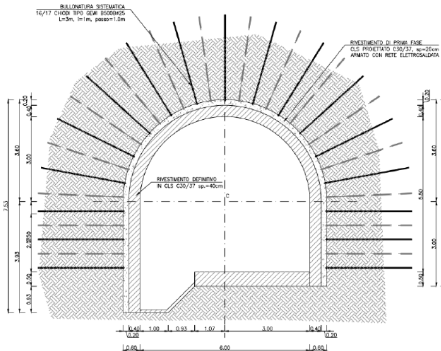
Figura 3.2: Sezione tipo della galleria ventilazione e cavi
