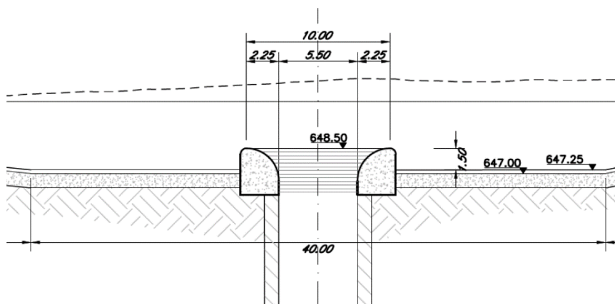
Figura 36 Sezione dell'opera di presa
