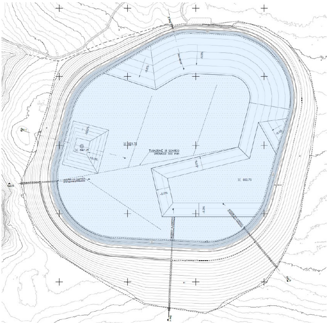
Figura 34 Planimetria del bacino di monte
