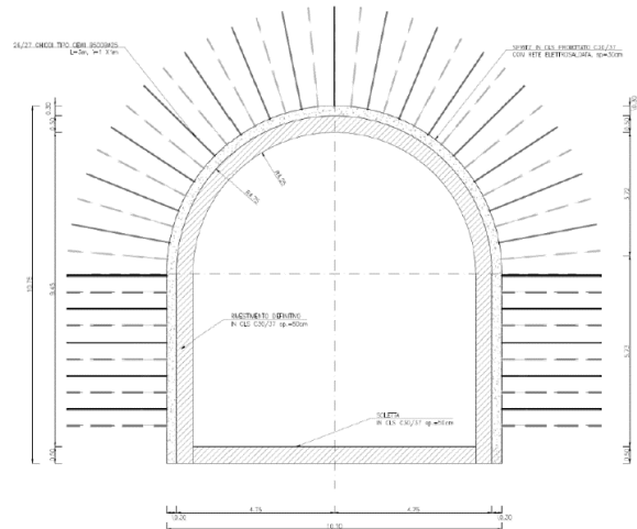
Figura 32 Sezioni tipo della galleria d'accesso al pozzo paratoie
