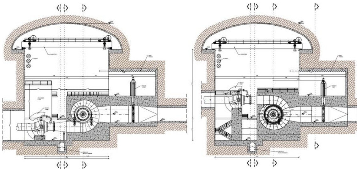
Figura 30 Sezioni della centrale in corrispondenza della turbina e della pompa
