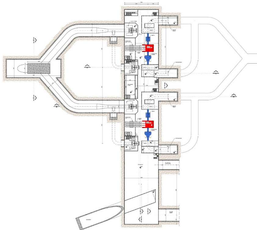
Figura 31 Pianta della centrale e biforcazioni di monte e di valle
