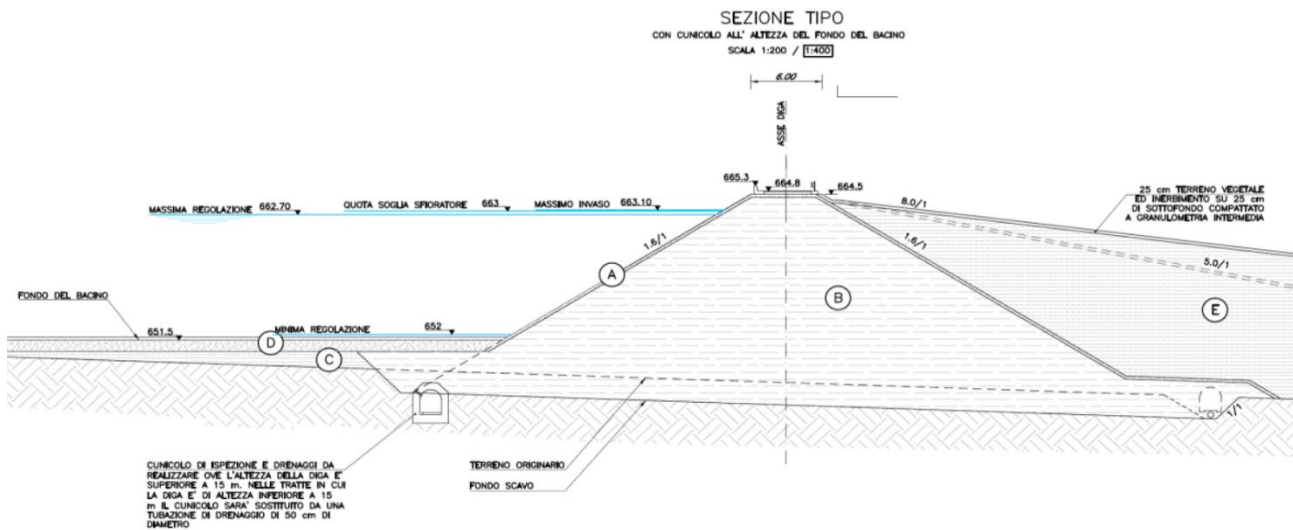
Figura 35 Sezione tipo del rilevato
