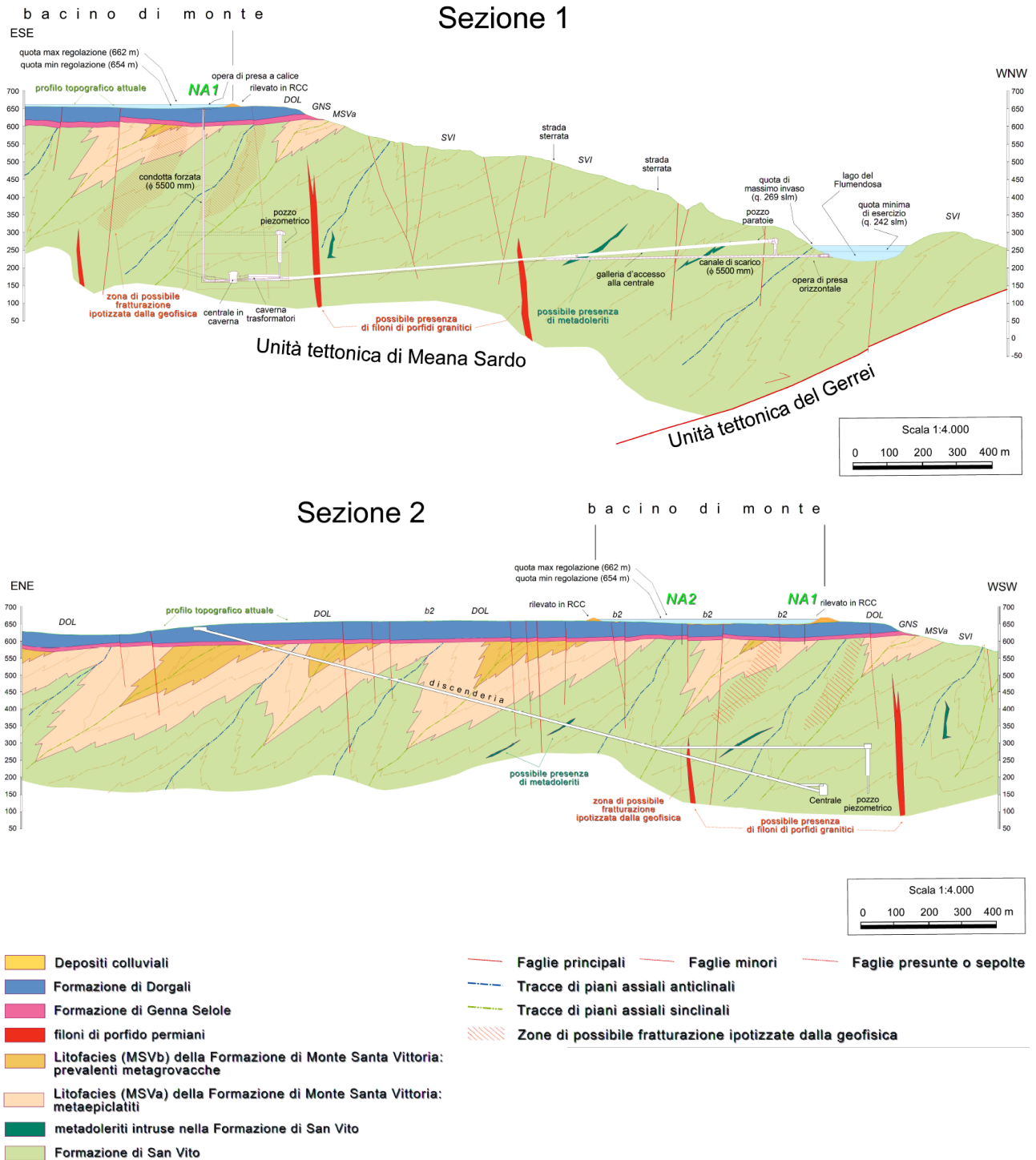
Figura 18 Sezioni geologiche lungo gli assi della galleria (Sez. 1) e della discenderia (Sez. 2)
