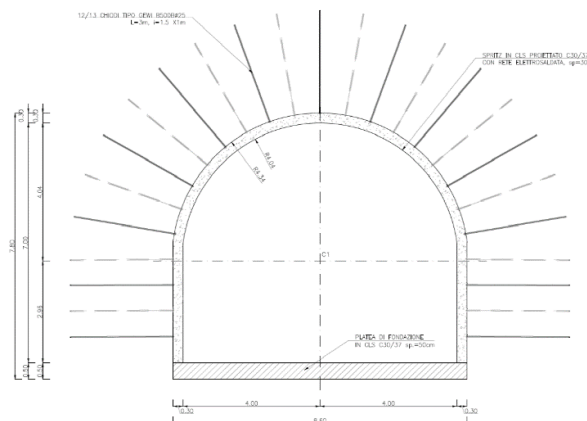
Figura 33 Sezioni tipo della galleria d'accesso al pozzo piezometrico
