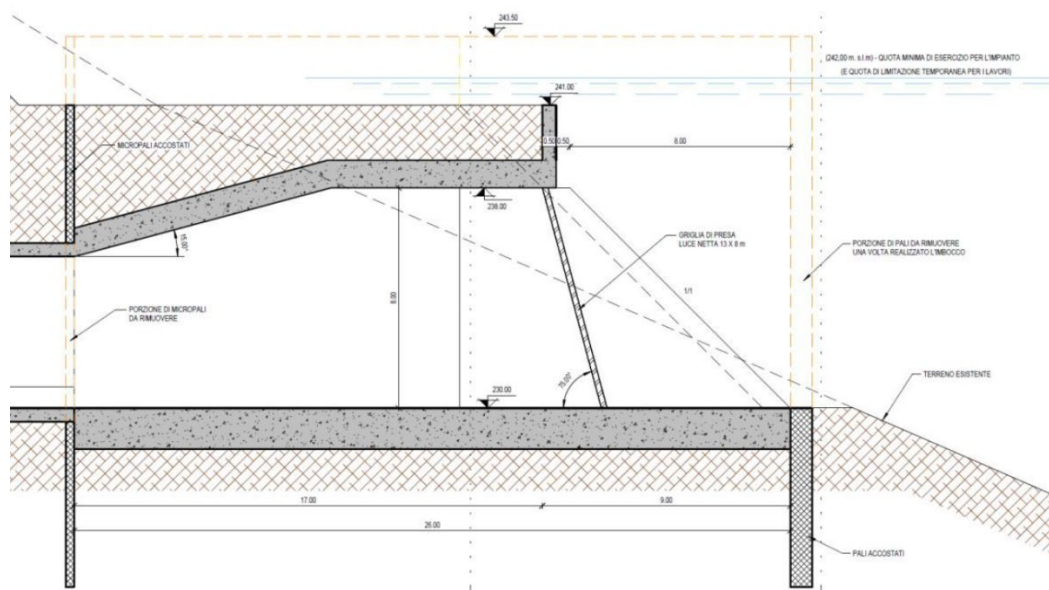
Figura 28 Sezione longitudinale dell'opera di presa di valle
