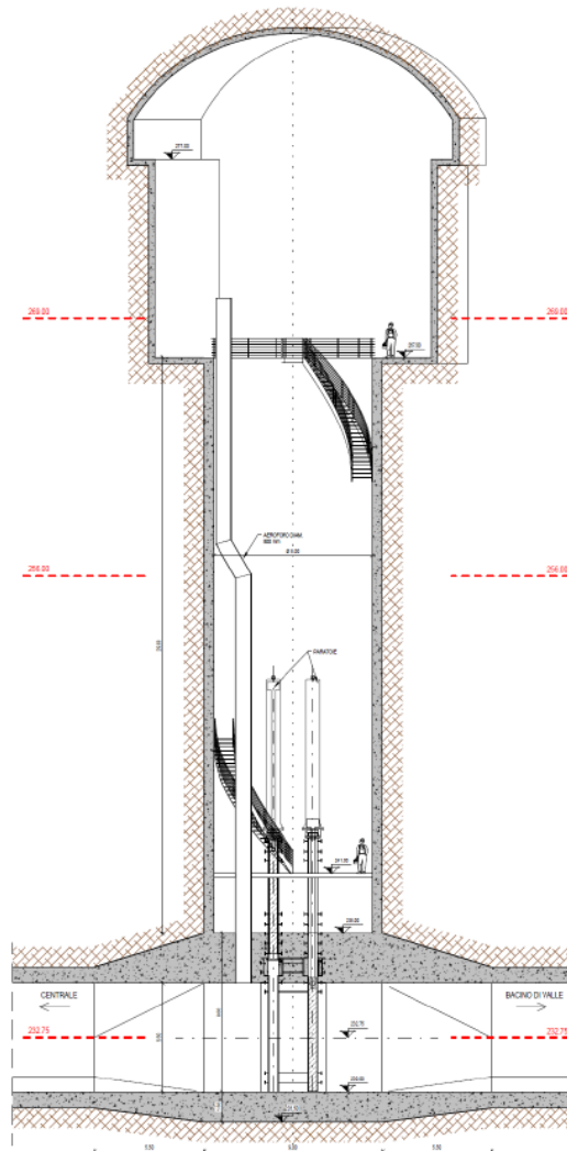
Figura 29 Sezione del pozzo paratoie
