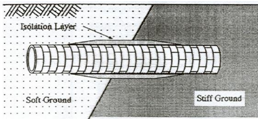
Figura 4.3 – Isolamento esteso del tunnel (Kawashima, 2000)
