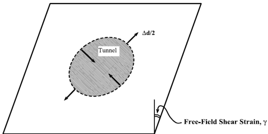
Figura 3.1 – Applicazione delle deformazioni di taglio sui bordi del modello per l'applicazione del Metodo delle deformazioni di taglio puro in campo libero
