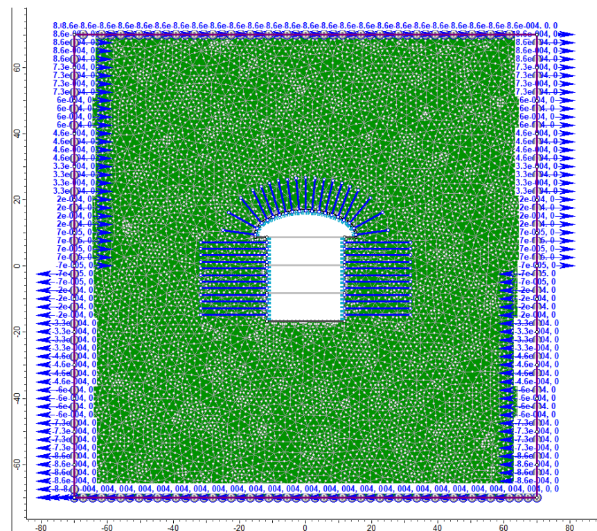
Figura 4.2 – Modello relativo alla Centrale in Caverna per le condizioni sismiche all'ultimo step di analisi
