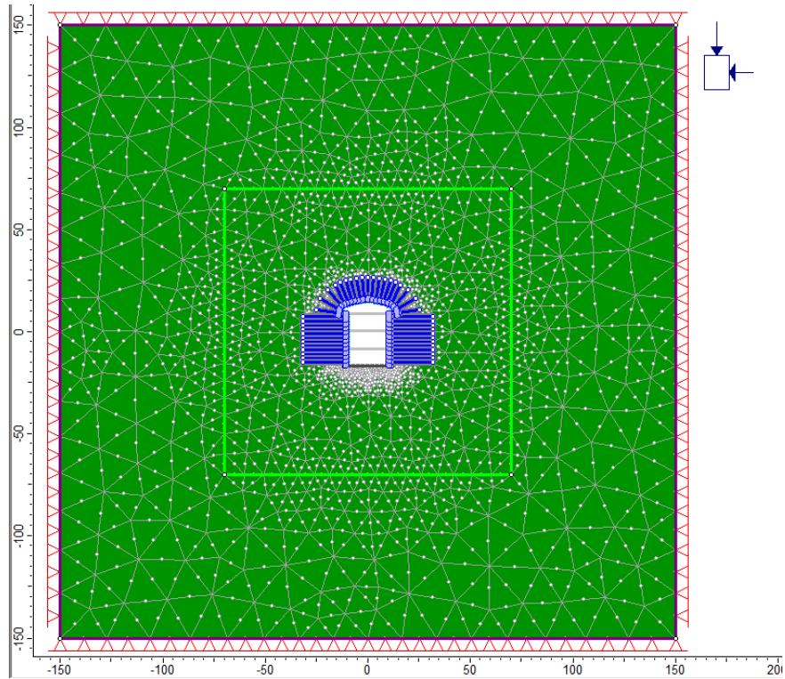
Figura 4.1 – Modello relativo alla Centrale in Caverna per le condizioni statiche all'ultimo step di analisi
