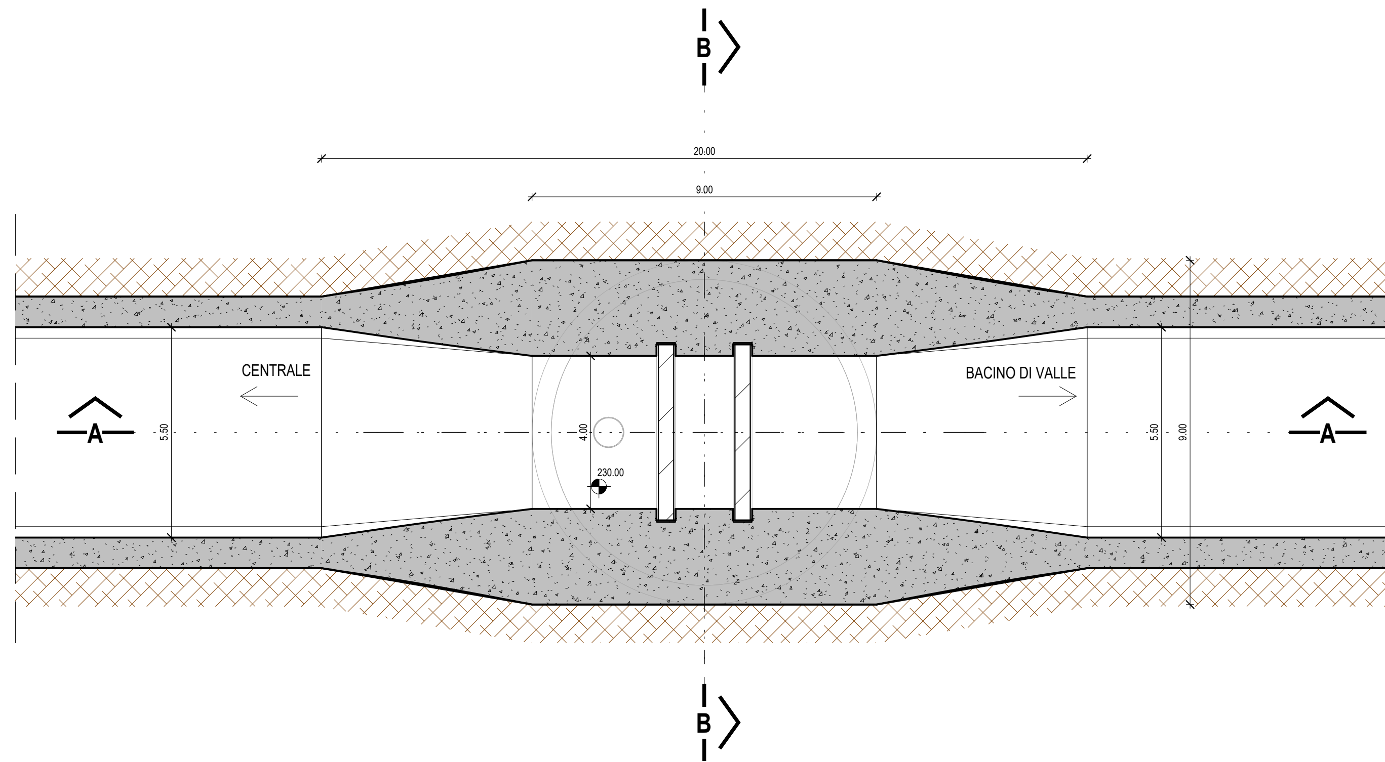
PIANTA A QUOTA 232.75 m slm 1 : 100
