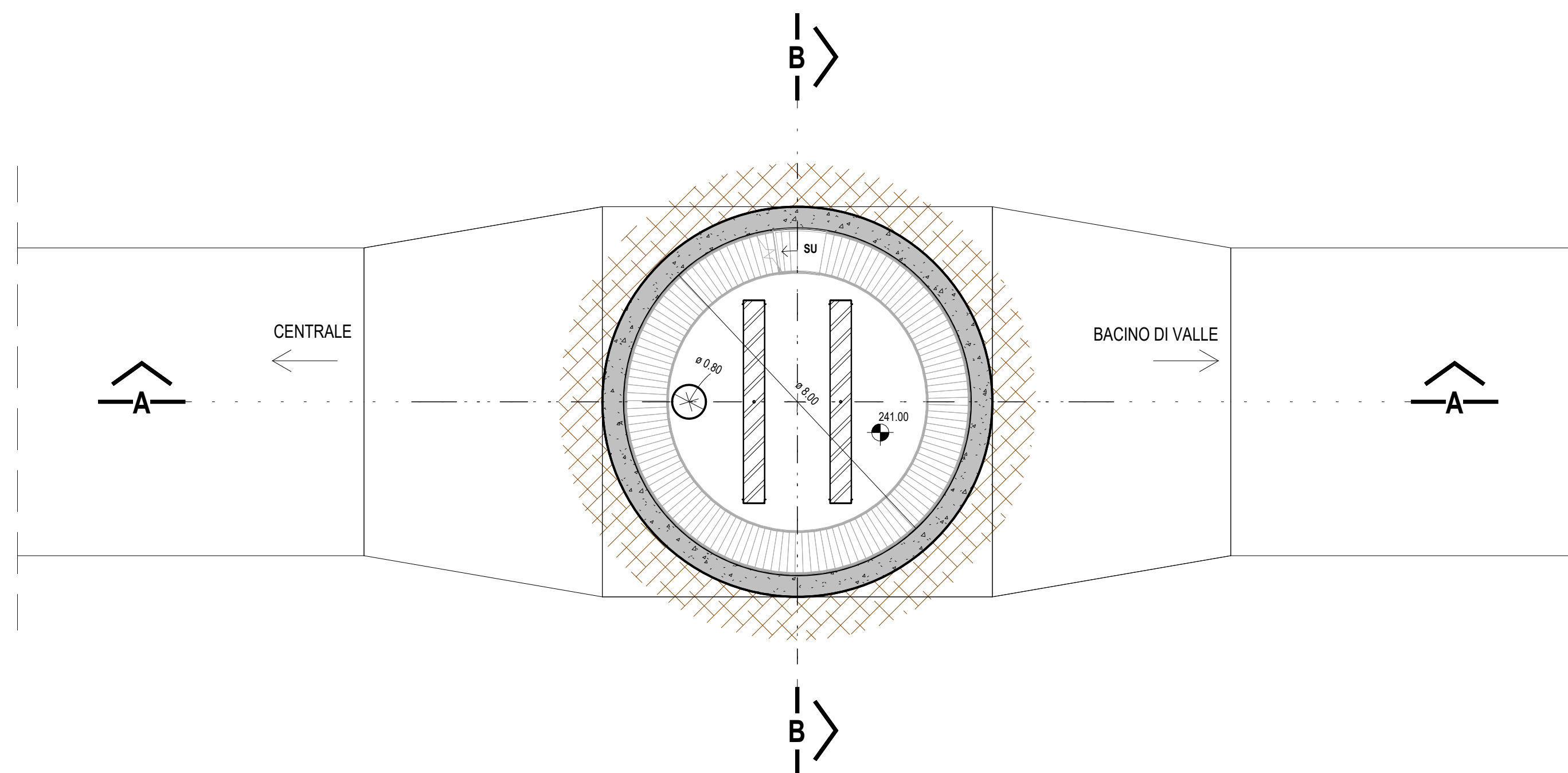
PIANTA A QUOTA 256.00 m slm 1 : 100
